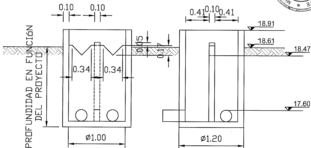
CORTE BB
