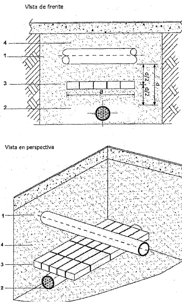
Figura 2b Protección con ladrillos Cruce
