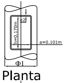
Detalle refuerzo de Ventana Vista de Frente
