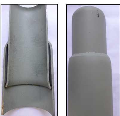
DETALLE 2: Unión de dos tramos contiguos de la columna mediante abocardado doble con soldadura exterior e interior s/Normas IRAM.
