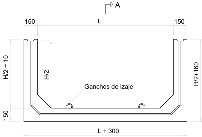
Vista Frontal Módulo Inferior Esc. 1:25
