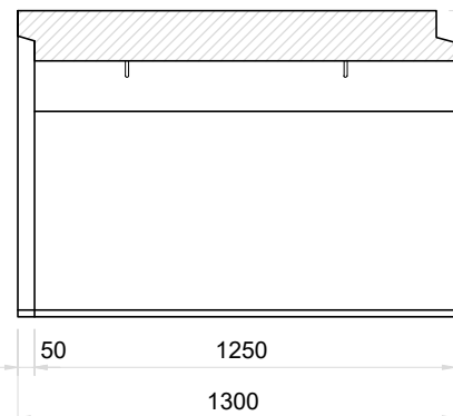
Sección A-A Módulo Superior Esc. 1:25
