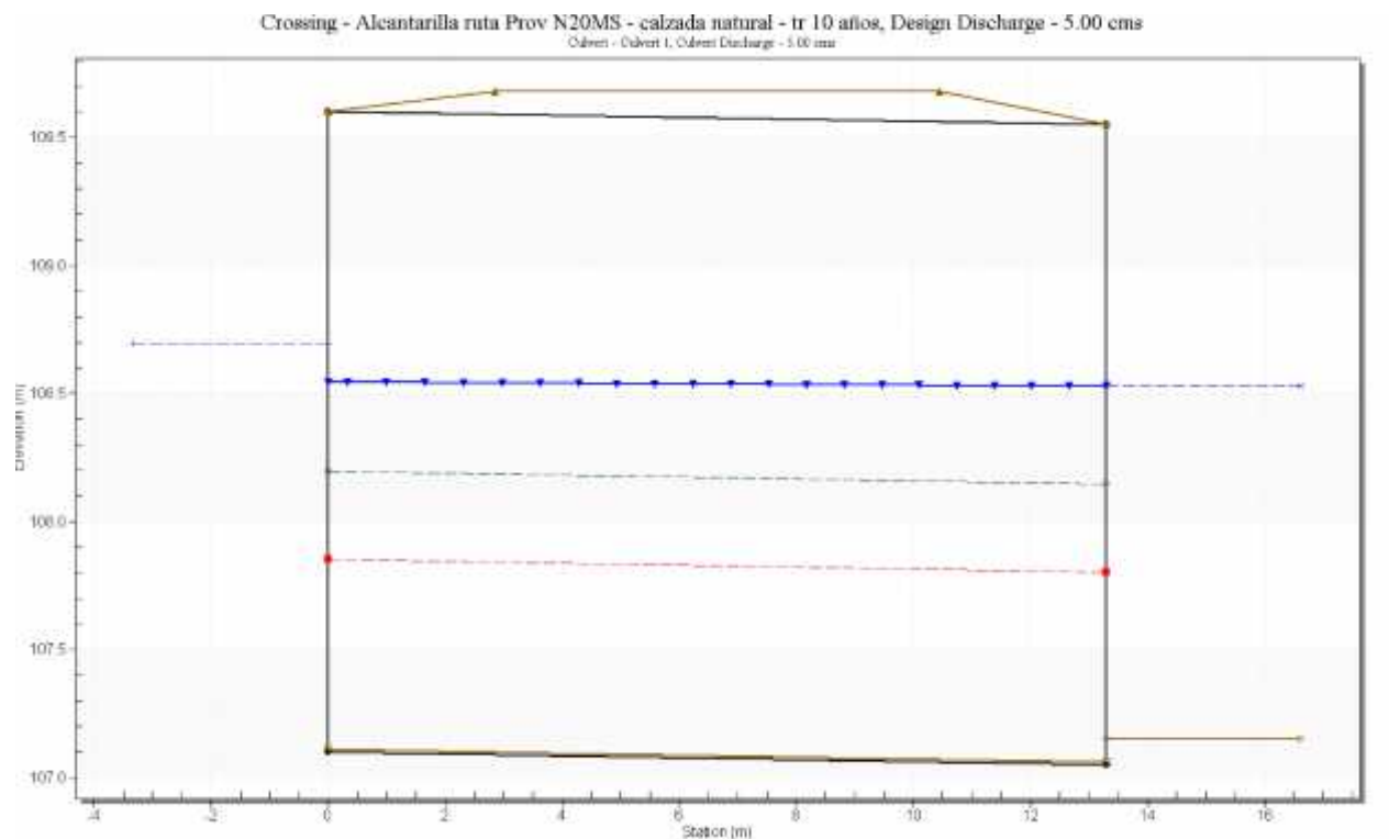
Imagen9: Salida del software HY-8 para caudal de diseño de 10 años.
