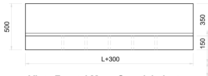
Vista Frontal Muro Guardabalastos Esc. 1:25
