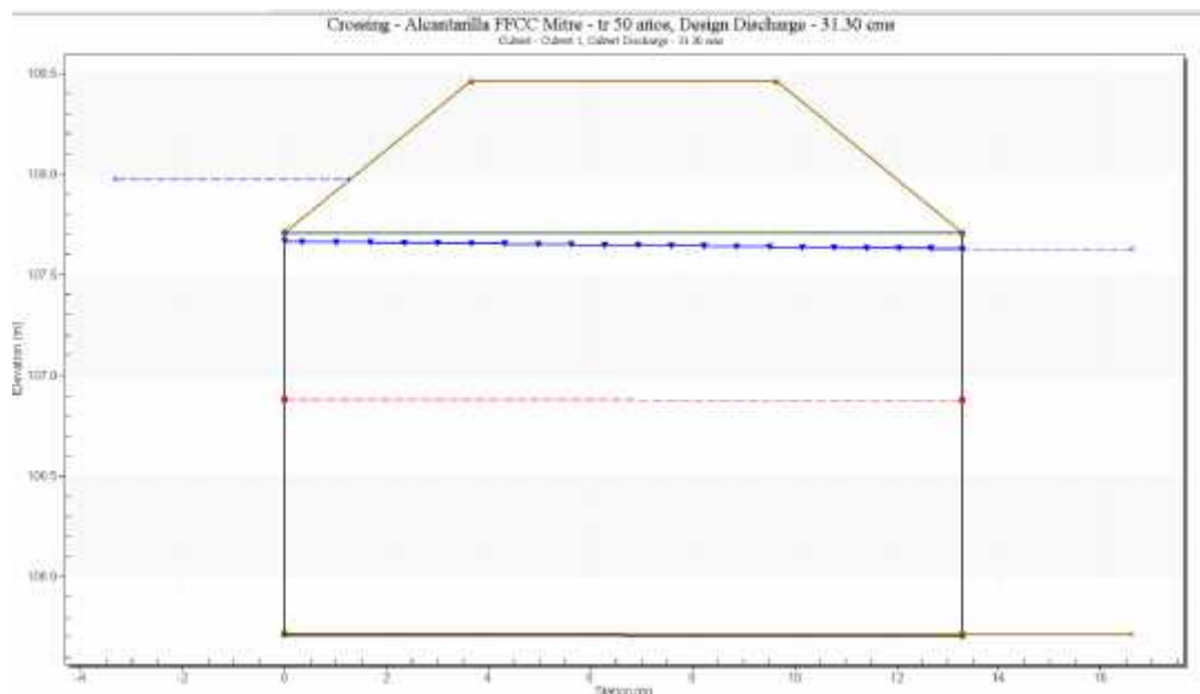
Imagen9: Salida del software HY-8 para caudal de diseño de 50 años.
