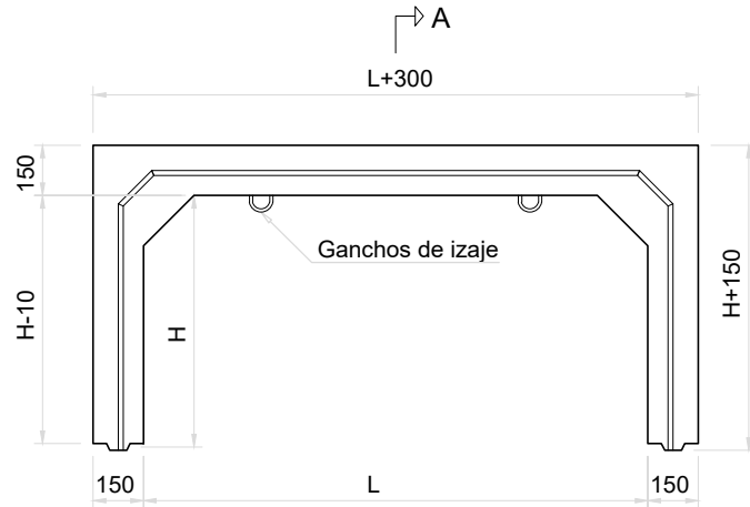
Vista Frontal Módulo Superior Esc. 1:25
