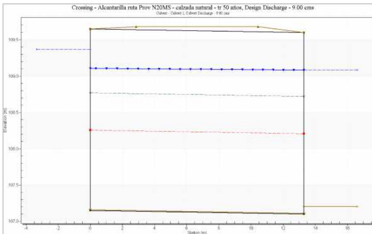
Imagen10: Salida del software HY-8 para caudal de diseño de 50 años.
