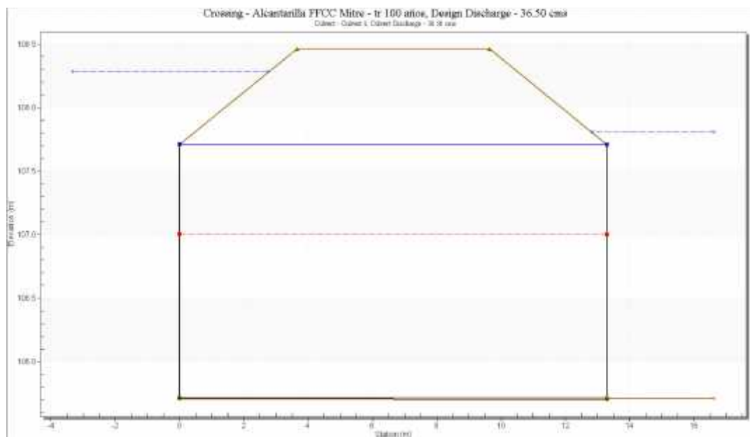
Imagen10: Salida del software HY-8 para caudal de diseño de 100 años.
