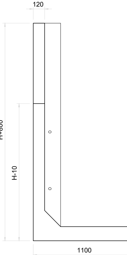
Vista Frontal Muro de Ala Tipo A Esc. 1:25
