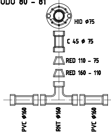
NUDO 80 - 81
