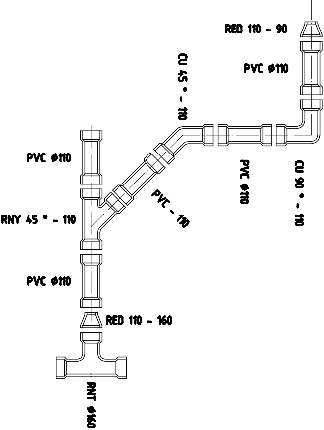
NUDOS DE PERFORACIONES 2 Y 5
