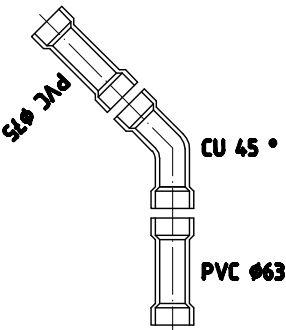
NUDO 70
