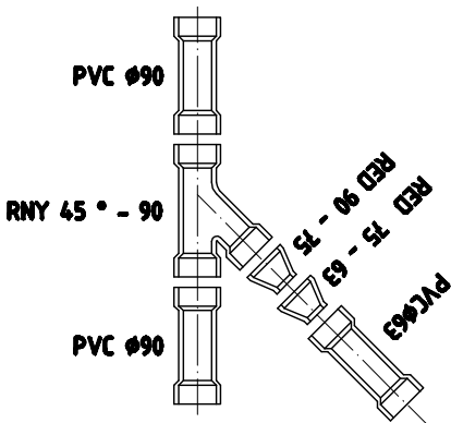
NUDO 66
