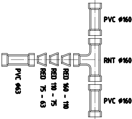
NUDOS 29 - 31 - 33 - 35 - 37 - 39 - 40 - 55
