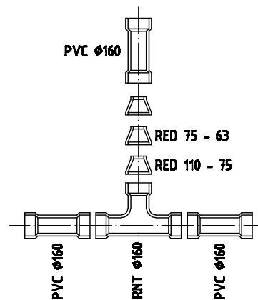
NUDO R'
