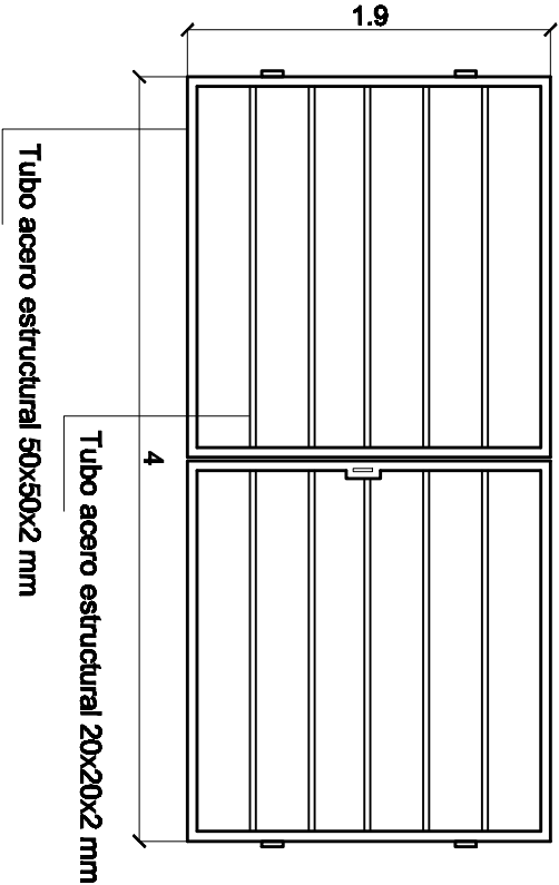
Detalle P1
