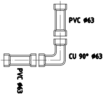
NUDOS 26 - 27
