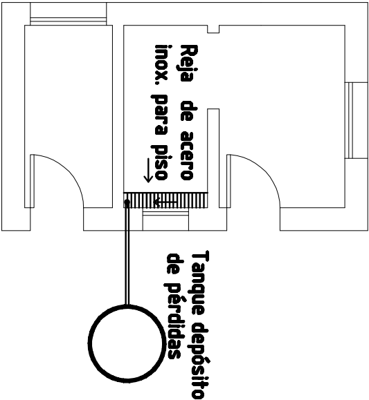
Planta de instalación de desagüe de pérdidas de cloro
