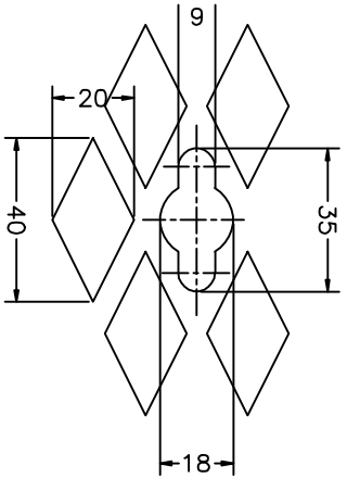
DETALLE "C"
