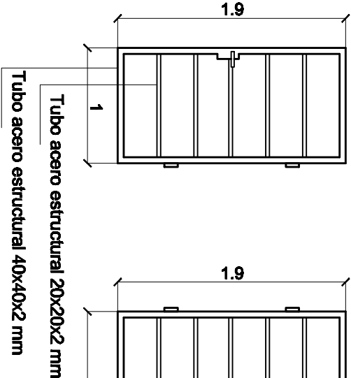
Detalle P2
