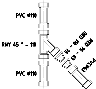
NUDO 70
