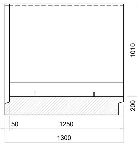
Sección A-A Módulo Inferior Esc. 1:25
