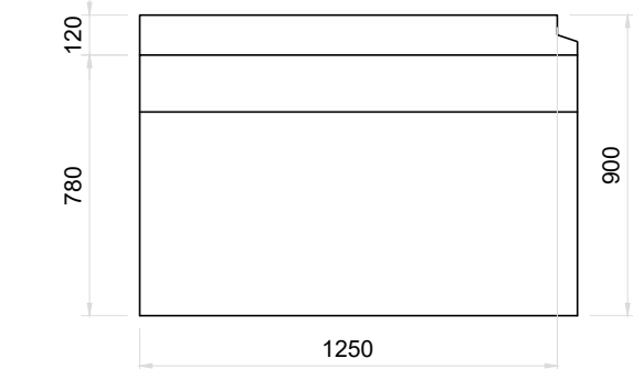
Vista Superior Muro de Ala Tipo B Esc. 1:25
