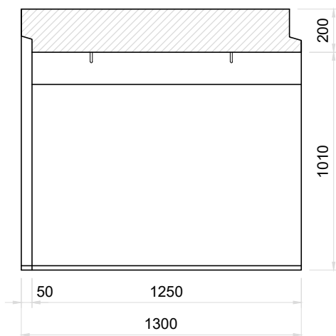
Sección A-A Módulo Superior Esc. 1:25
