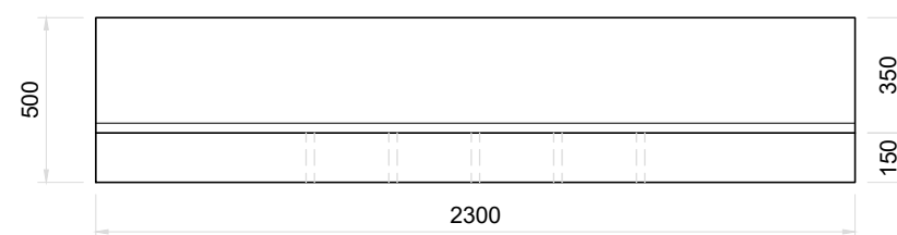
Vista Frontal Muro Guardabalastos Esc. 1:25
