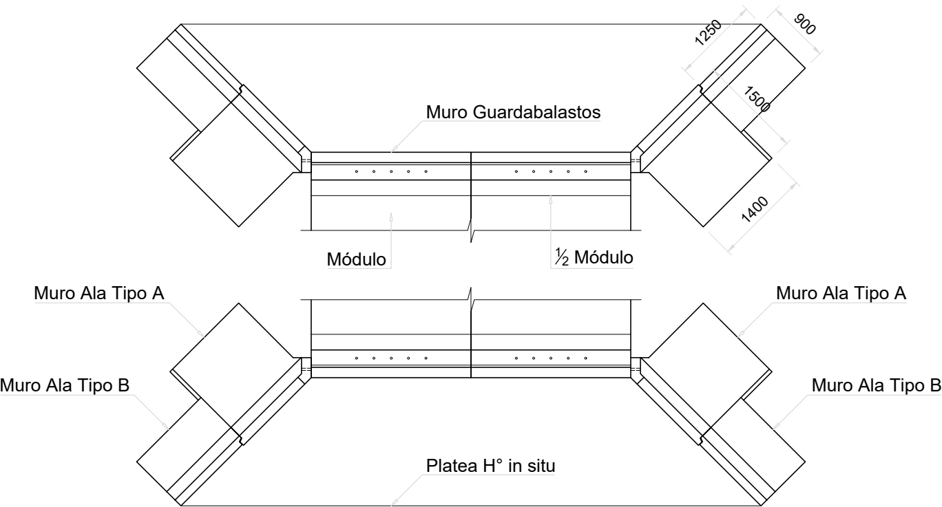
Vista Superior de la Alcantarilla Esc. 1:75
