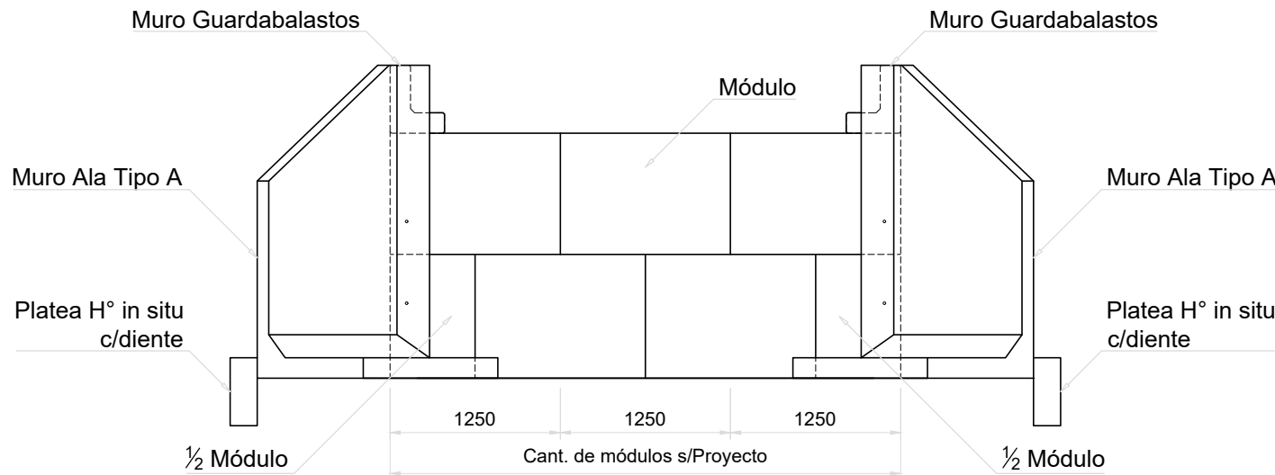
Vista Lateral de la Alcantarilla Esc. 1:50
