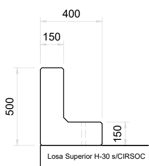
Vista Lateral Muro Guardabalastos
