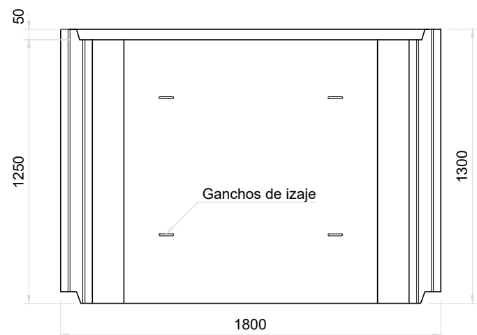
Vista Superior Módulo Inferior Esc. 1:25
