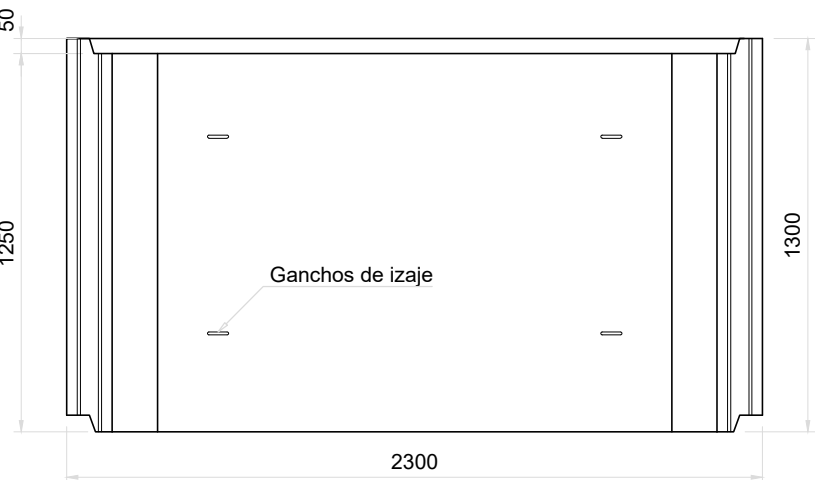
Vista Superior Módulo Inferior Esc. 1:25
