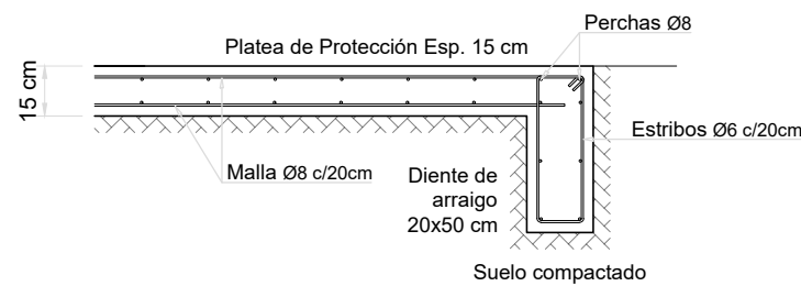
Detalle Placa de Protección Esc. 1:25
