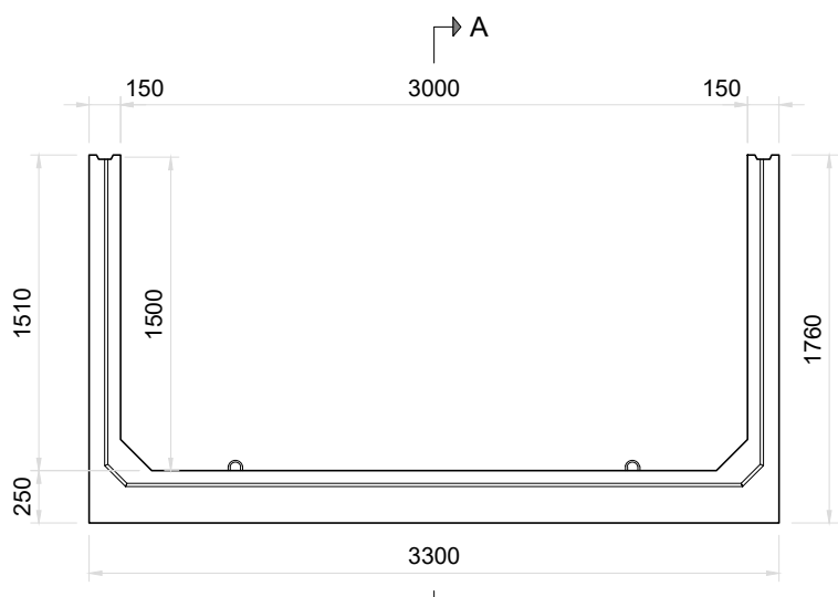
Vista Frontal Módulo Inferior
