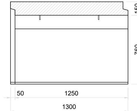
Sección A-A Módulo Superior Esc. 1:25
