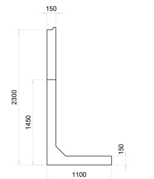
Vista Frontal Muro de Ala Tipo C
