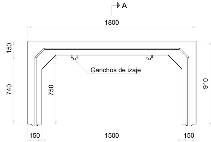
Vista Frontal Módulo Superior Esc. 1:25
