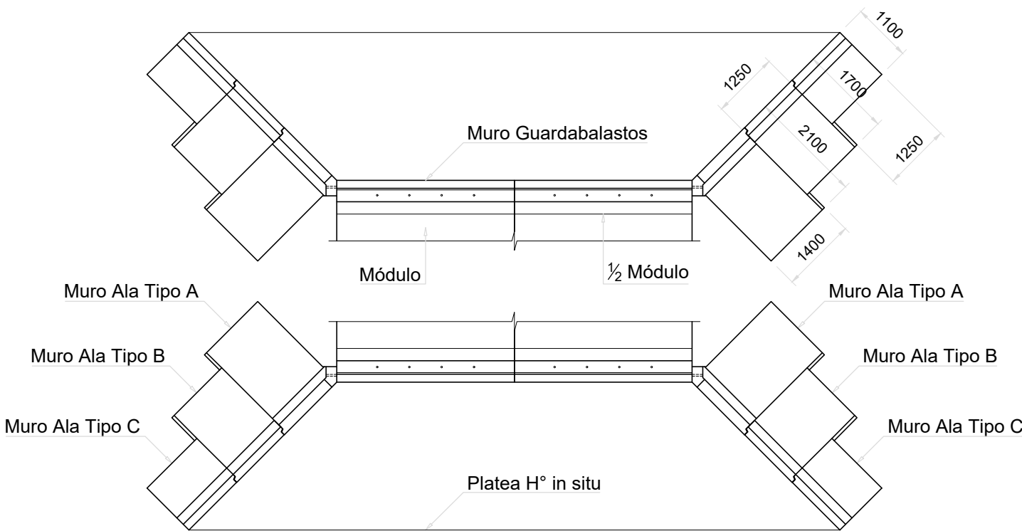
Vista Superior de la Alcantarilla
