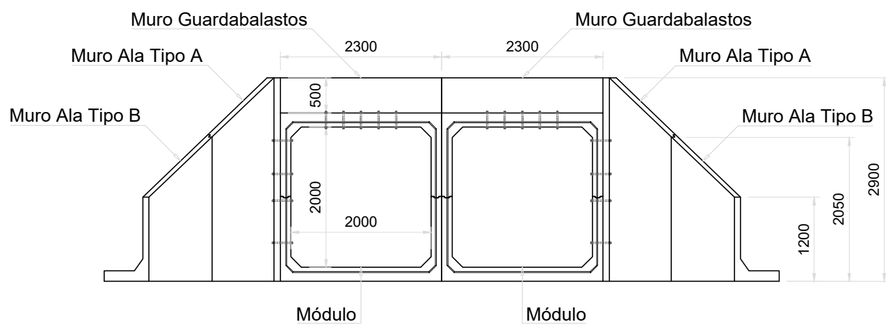
Vista Frontal de la Alcantarilla Esc. 1:75
