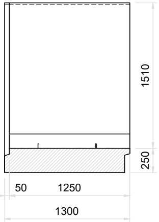
Sección A-A Módulo Inferior
