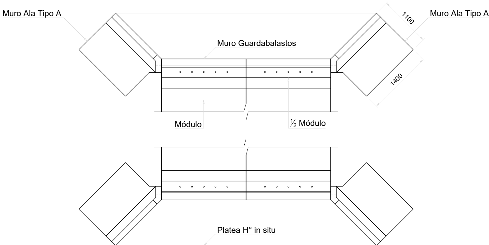
Vista Superior de la Alcantarilla Esc. 1:50
