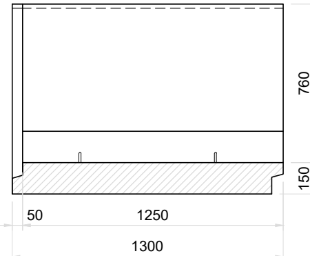
Sección A-A Módulo Inferior Esc. 1:25
