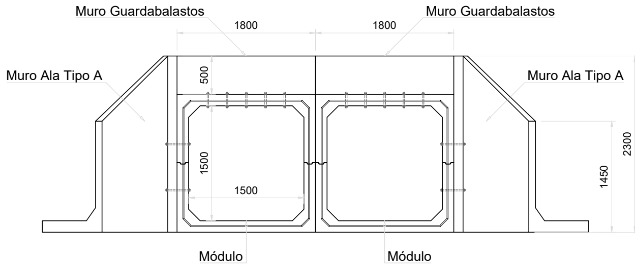
Vista Frontal de la Alcantarilla Esc. 1:50
