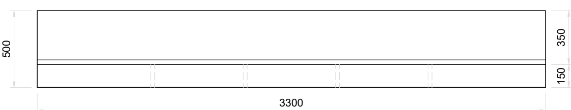
Vista Frontal Muro Guardabalastos
