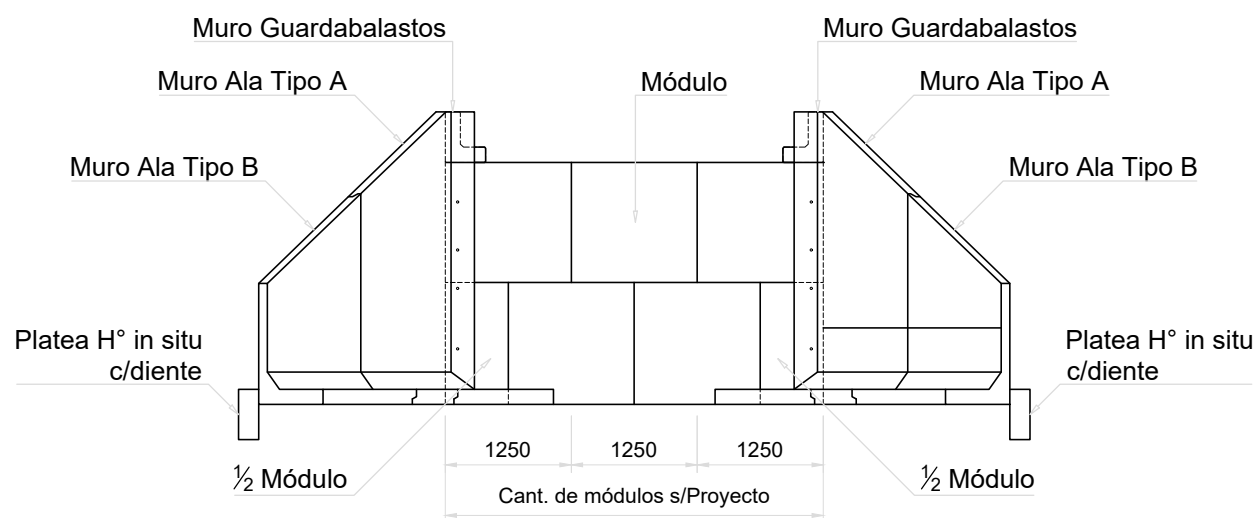
Vista Lateral de la Alcantarilla Esc. 1:75
