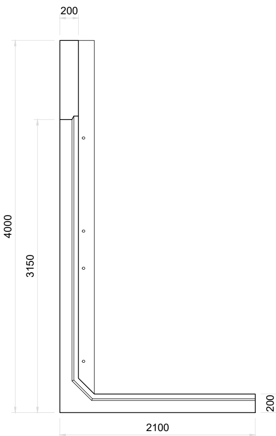
Vista Frontal Muro de Ala Tipo A
