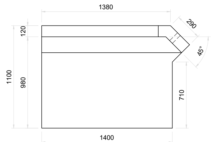
Vista Superior Muro de Ala Tipo A Esc. 1:25
