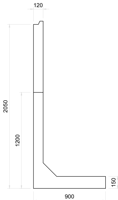
Vista Frontal Muro de Ala Tipo B Esc. 1:25
