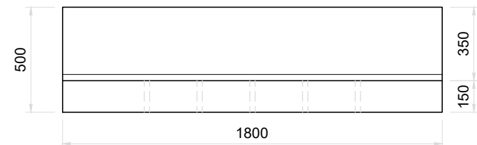
Vista Frontal Muro Guardabalastos Esc. 1:25
