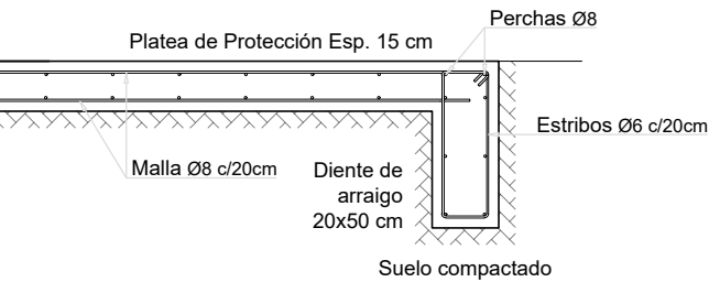
Detalle Platea de Protección
