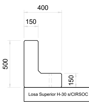
Vista Lateral Muro Guardabalastos Esc. 1:25
