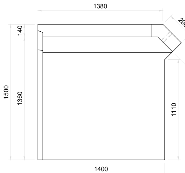
Vista Superior Muro de Ala Tipo A Esc. 1:25
