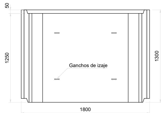
Vista Superior Módulo Superior Esc. 1:25
