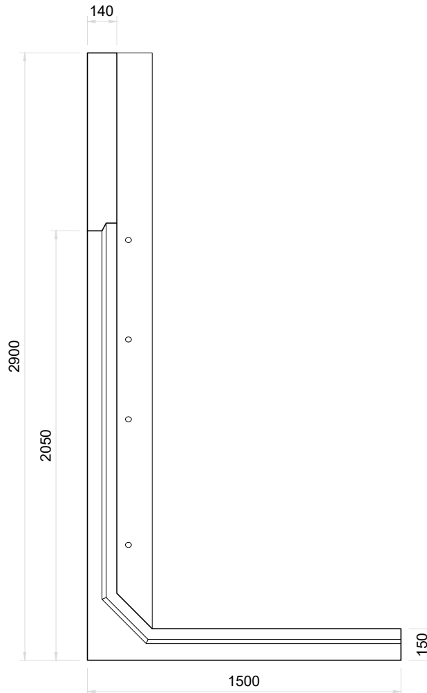
Vista Frontal Muro de Ala Tipo A Esc. 1:25
