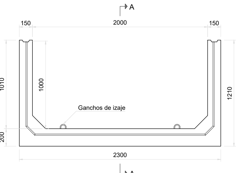
Vista Frontal Módulo Inferior Esc. 1:25
