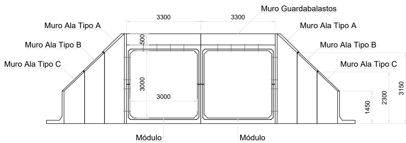
Vista Frontal de la Alcantarilla
