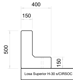
Vista Lateral Muro Guardabalastos Esc. 1:25
