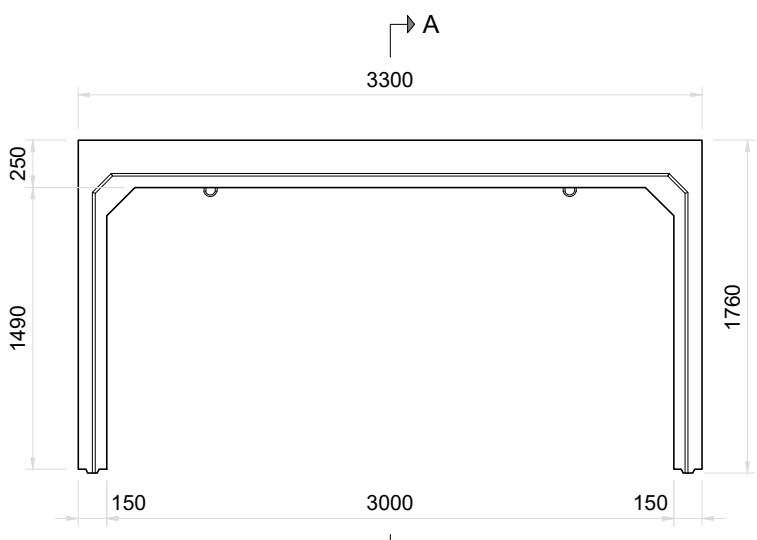
Vista Frontal Módulo Superior
