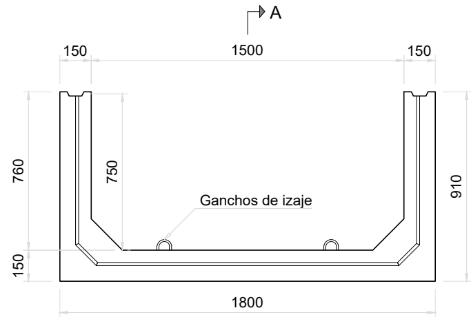
Vista Frontal Módulo Inferior Esc. 1:25
