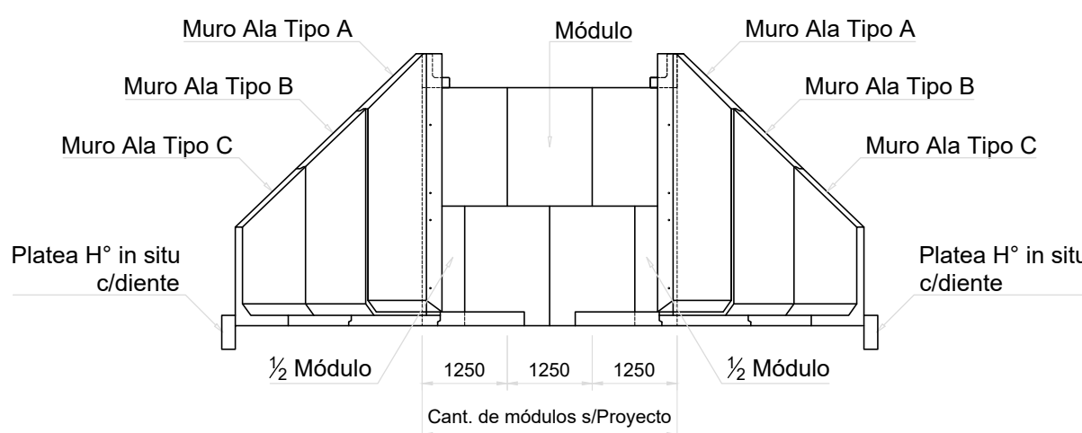
Vista Lateral de la Alcantarilla
