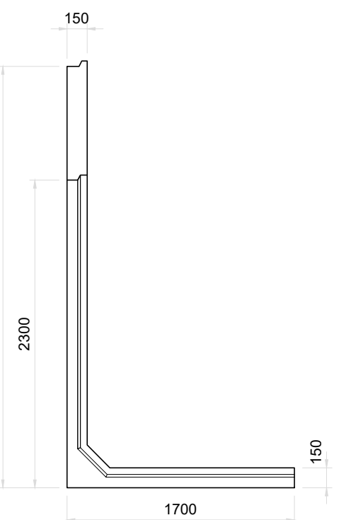
Vista Frontal Muro de Ala Tipo B
