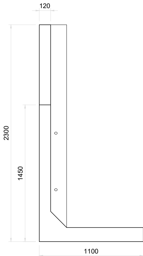
Vista Frontal Muro de Ala Tipo A Esc. 1:25
