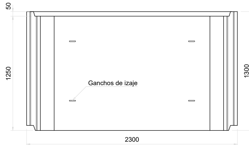
Vista Superior Módulo Superior Esc. 1:25
