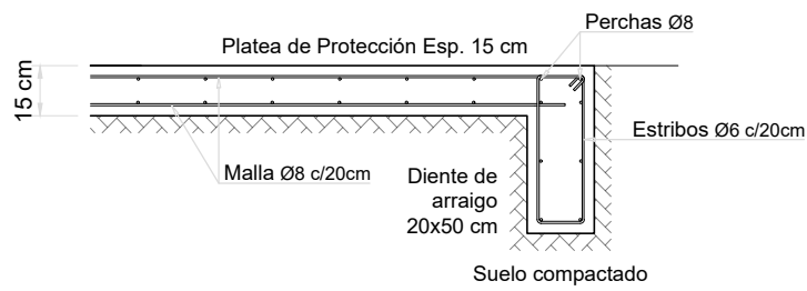
Detalle Platea de Protección Esc. 1:25
