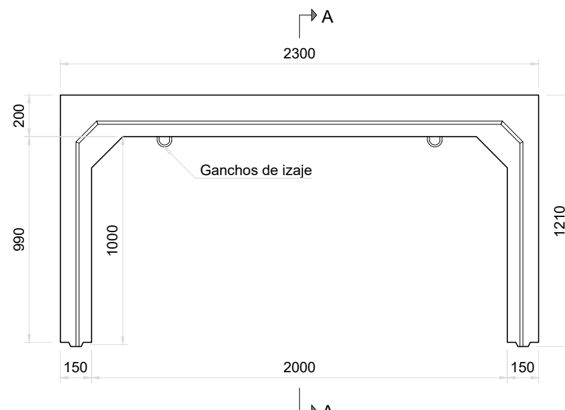
Vista Frontal Módulo Superior Esc. 1:25
