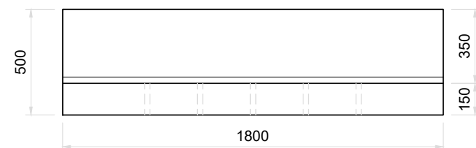
Vista Frontal Muro Guardabalastos Esc. 1:25
