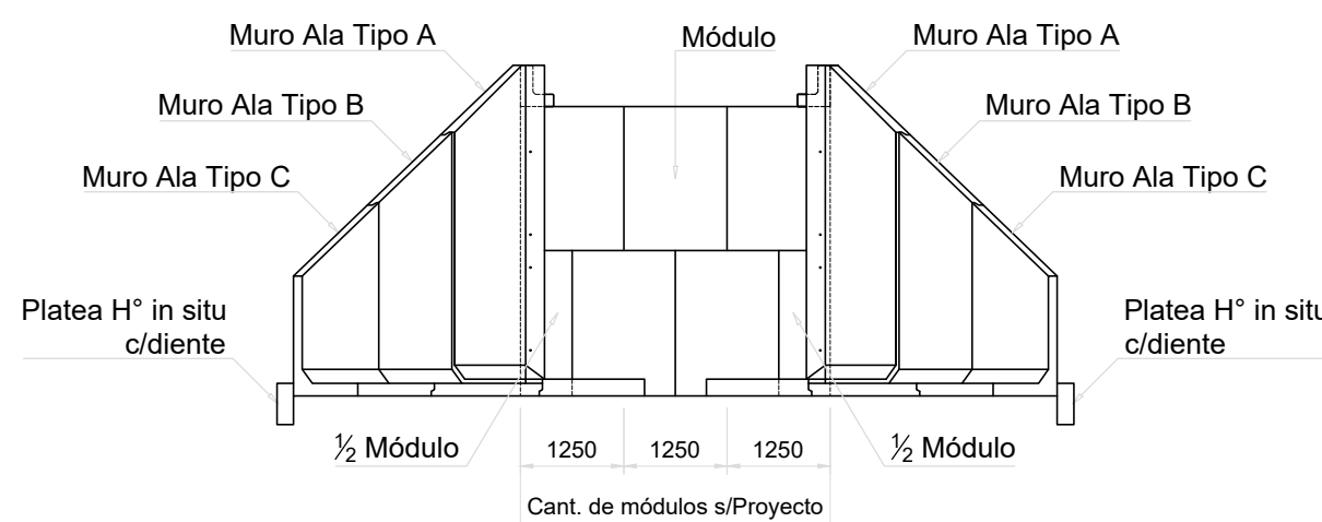
Vista Lateral de la Alcantarilla Esc. 1:100
