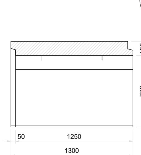
Sección A-A Módulo Superior Esc. 1:25
