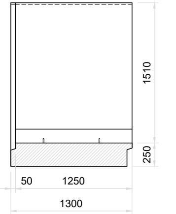
Sección A-A Módulo Inferior Esc. 1:40
