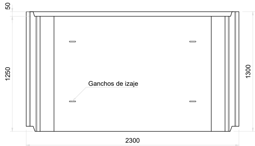
Vista Superior Módulo Inferior Esc. 1:25
