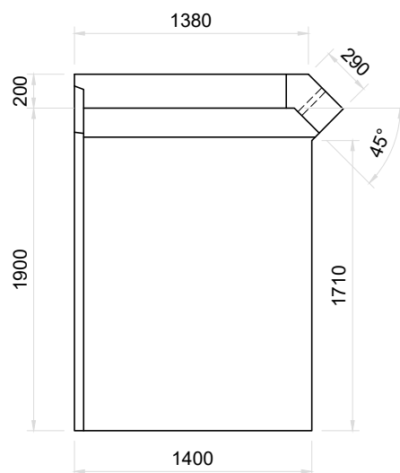
Vista Superior Muro de Ala Tipo A Esc. 1:40
