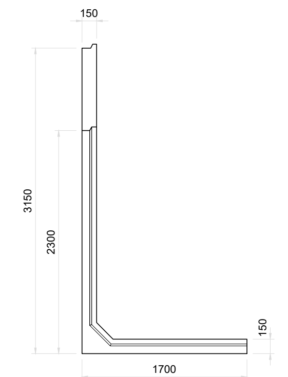
Vista Frontal Muro de Ala Tipo B Esc. 1:40
