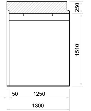
Sección A-A Módulo Superior Esc. 1:40
