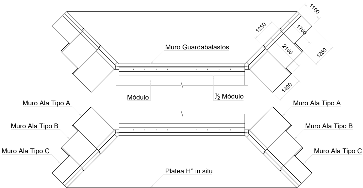
Vista Superior de la Alcantarilla Esc. 1:100
