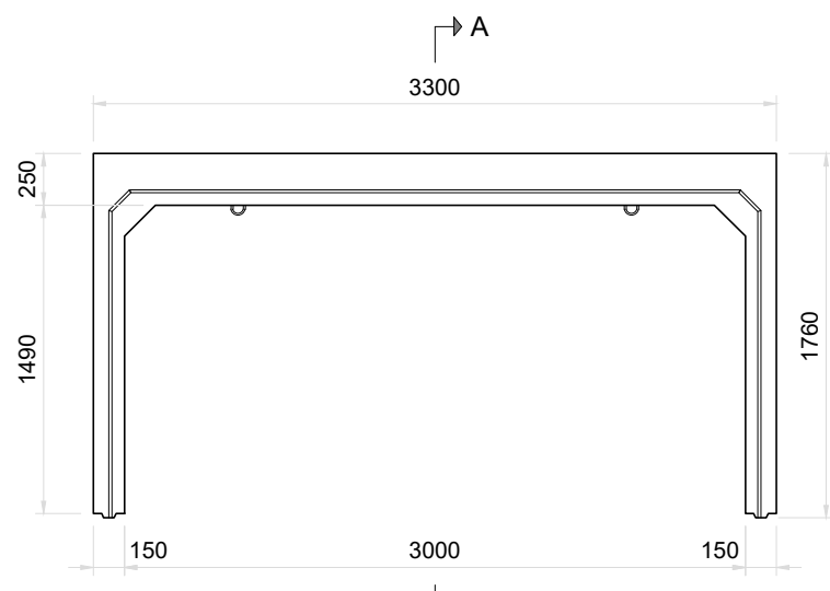
Vista Frontal Módulo Superior Esc. 1:40
