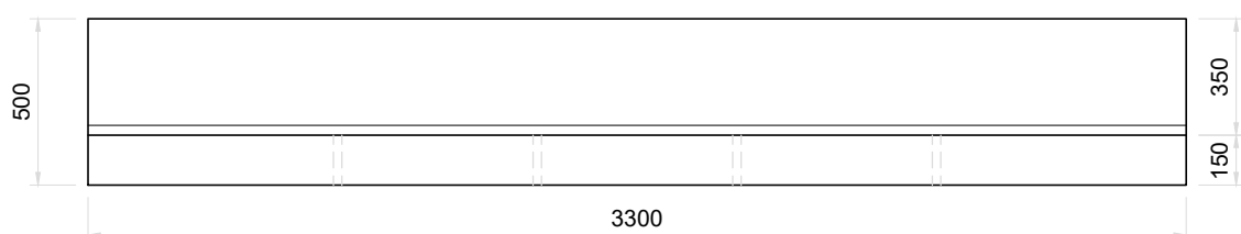
Vista Frontal Muro Guardabalastos Esc. 1:25
