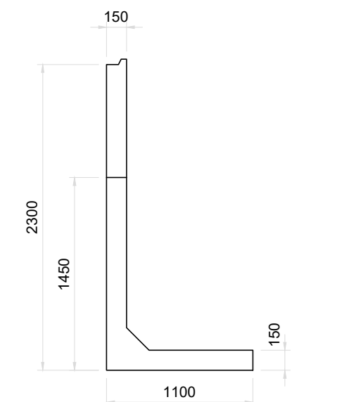
Vista Frontal Muro de Ala Tipo C Esc. 1:40
