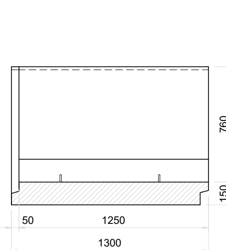
Sección A-A Módulo Inferior Esc. 1:25
