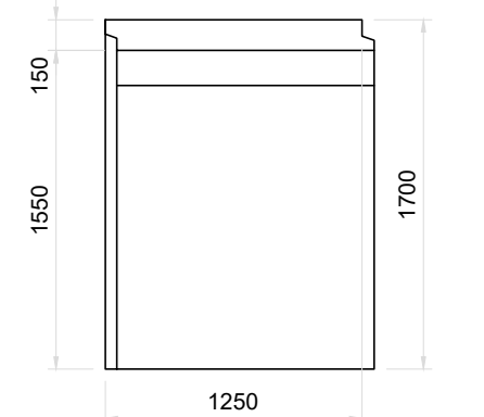
Vista Superior Muro de Ala Tipo B Esc. 1:40
