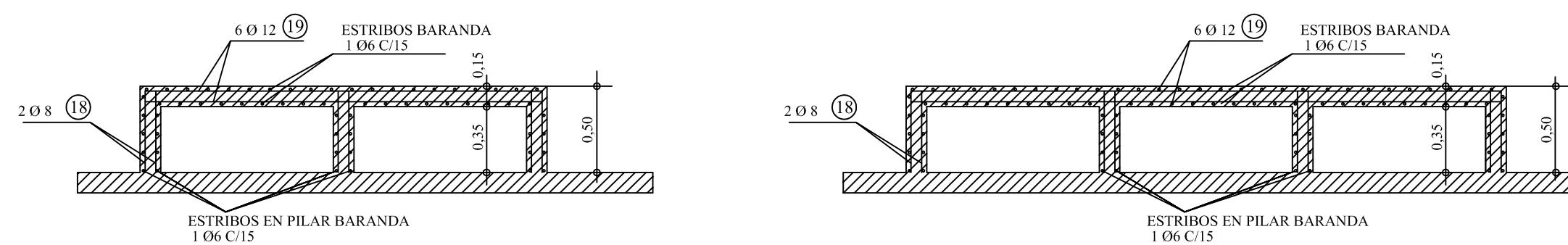
DETALLE DE ARMADURA BARANDA SIN ESCALA
