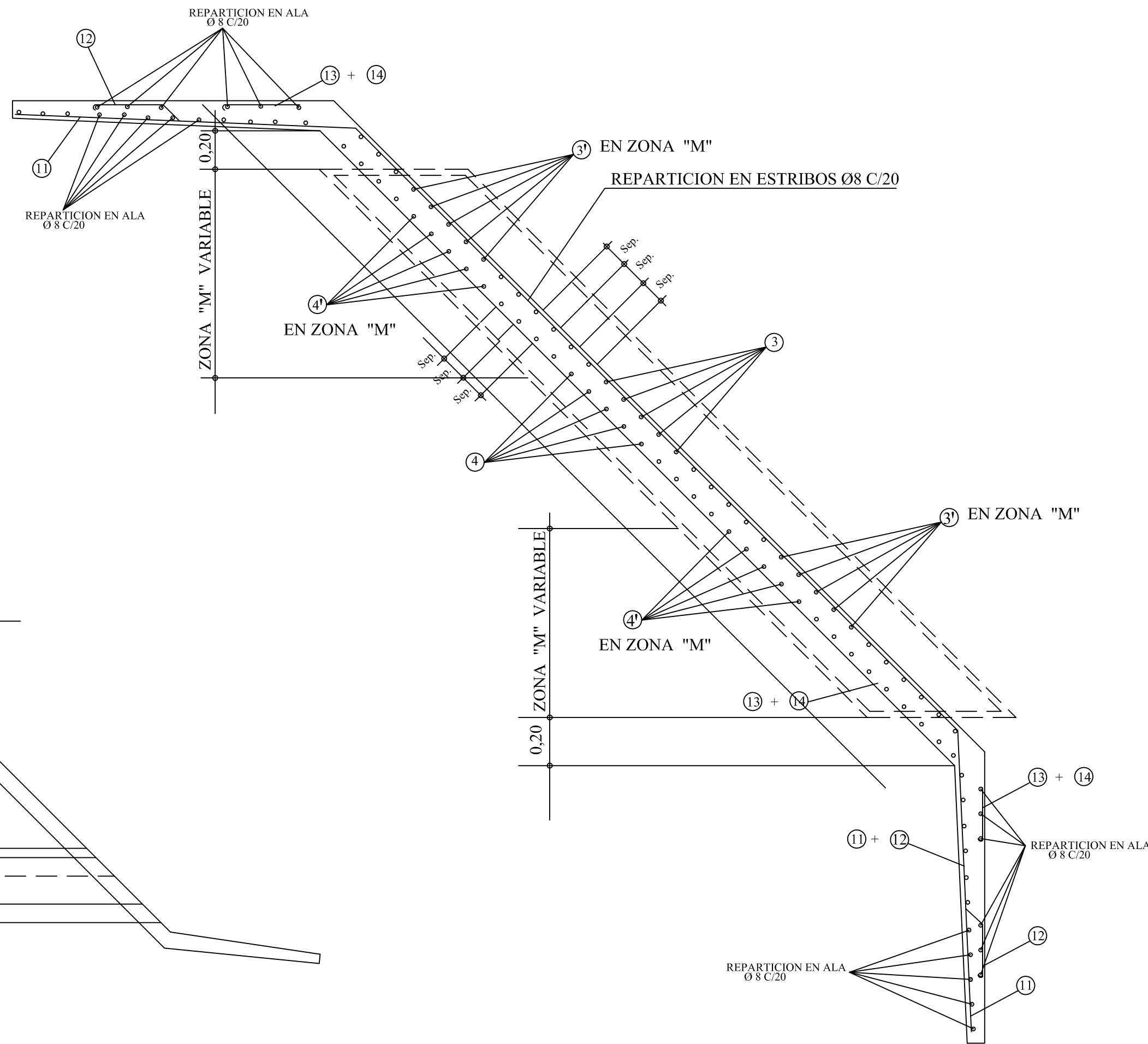
DETALLE DE ARMADURAS EN ESTRIBOS SIN ESCALA
