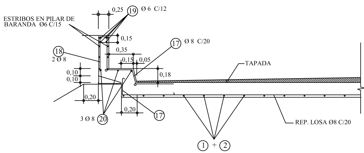
DETALLE DE ARMADURAS EN BARANDA Y LOSA SIN ESCALA
