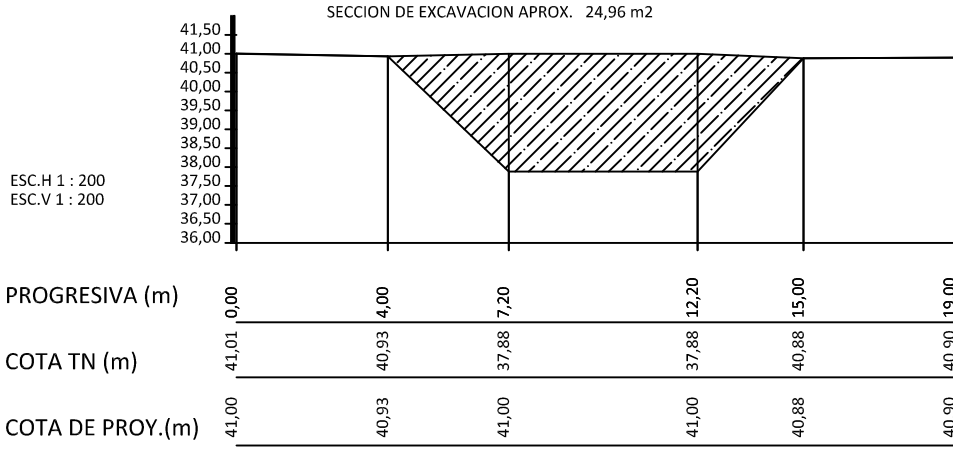
PERFIL TRANSVERSAL Nº 1 PERFIL TRANSVERSAL A DEL SAUCE Y CRUCE FUTURO CAMINO
