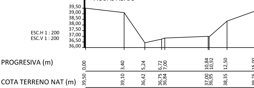
PERFIL TRANSVERSAL Nº 3 PERFIL TRANSVERSAL A DEL SAUCE EN LA DESCARGA AGUAS ABAJO
