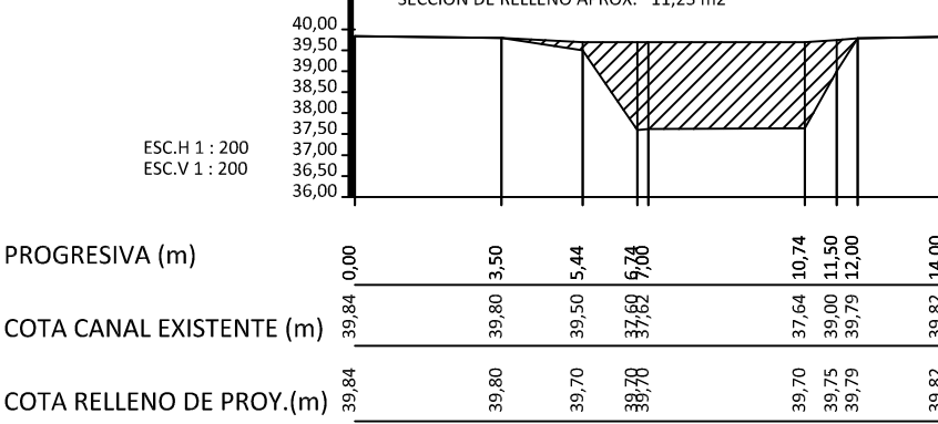
PERFIL TRANSVERSAL Nº 2 PERFIL TRANSVERSAL A DEL SAUCE SECTOR A RELLENAR
