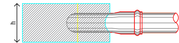
VISTA LATERAL Anclaje anclaje Curva 90°
