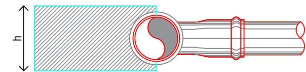
VISTA LATERAL Anclaje Ramal Normal Te
