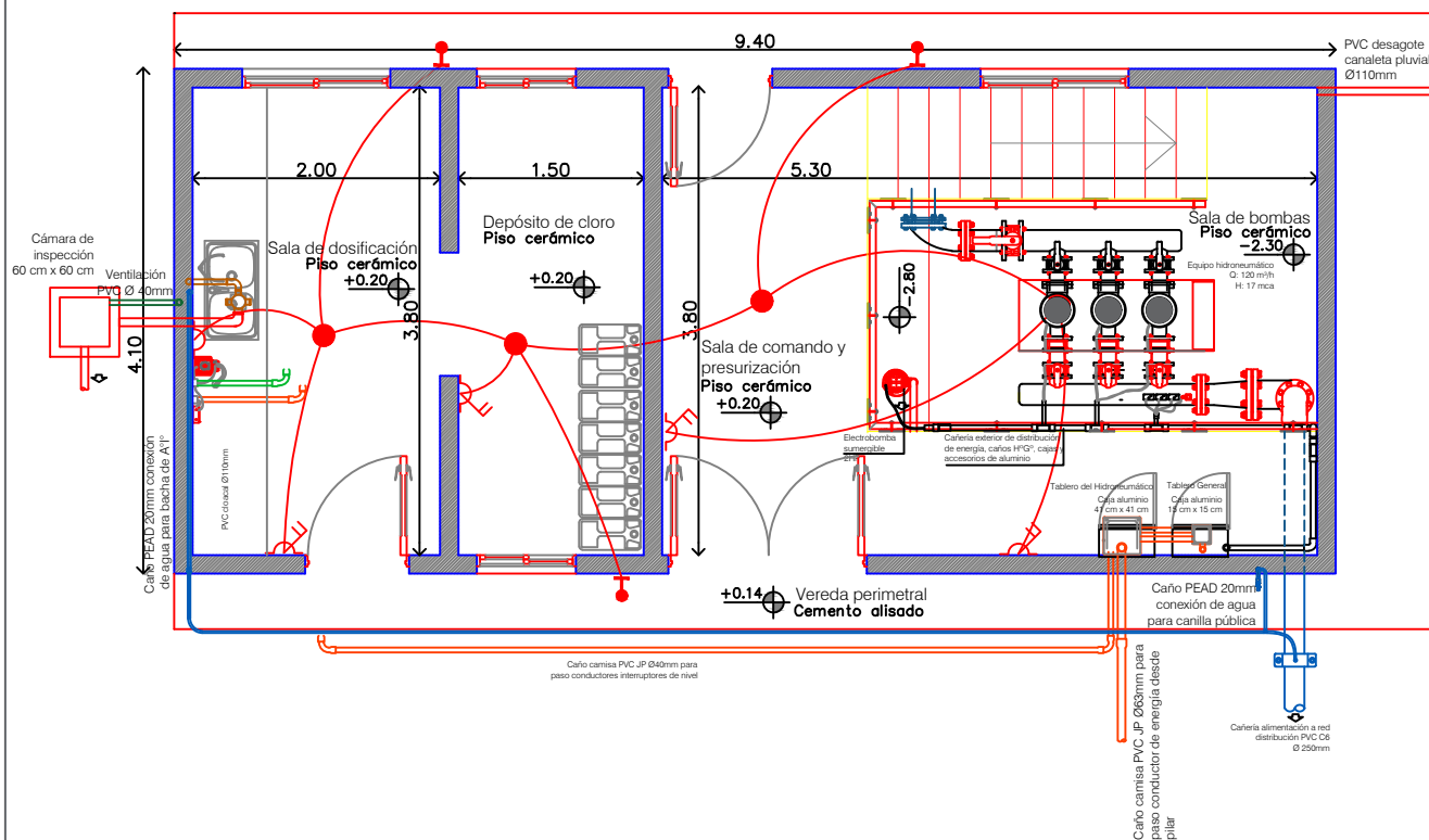
Instalaciones Esc. 1:50
