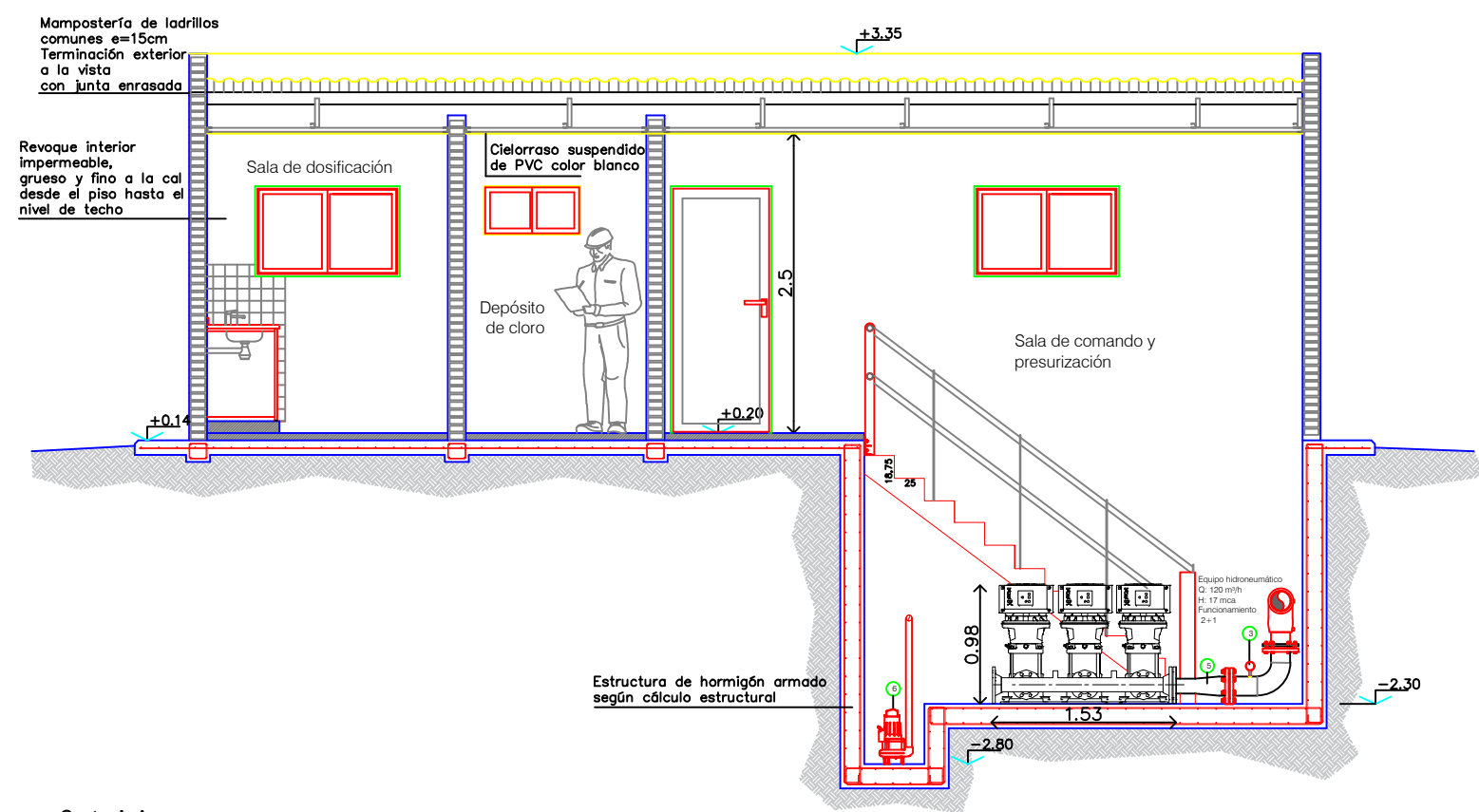
Corte A-A
