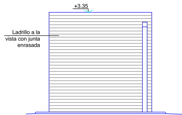
Fachada Norte Esc. 1:50
