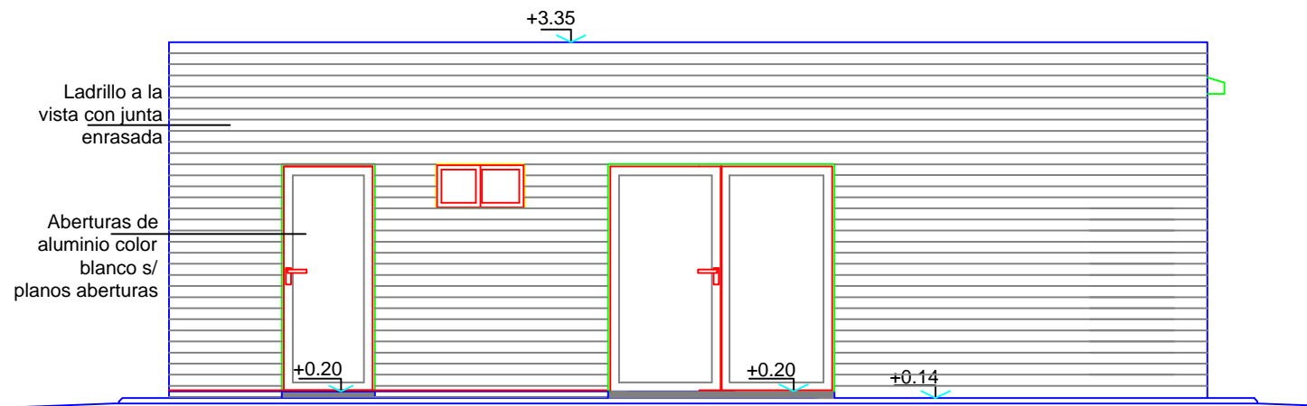
Fachada Este Esc. 1:50
