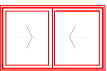
Ventana doble hoja corrediza Aluminio color blanco tipo Módena Vidrio laminado 6mm Cantidad: 1
