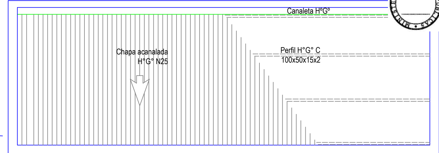
Planta de techos Esc. 1:50
