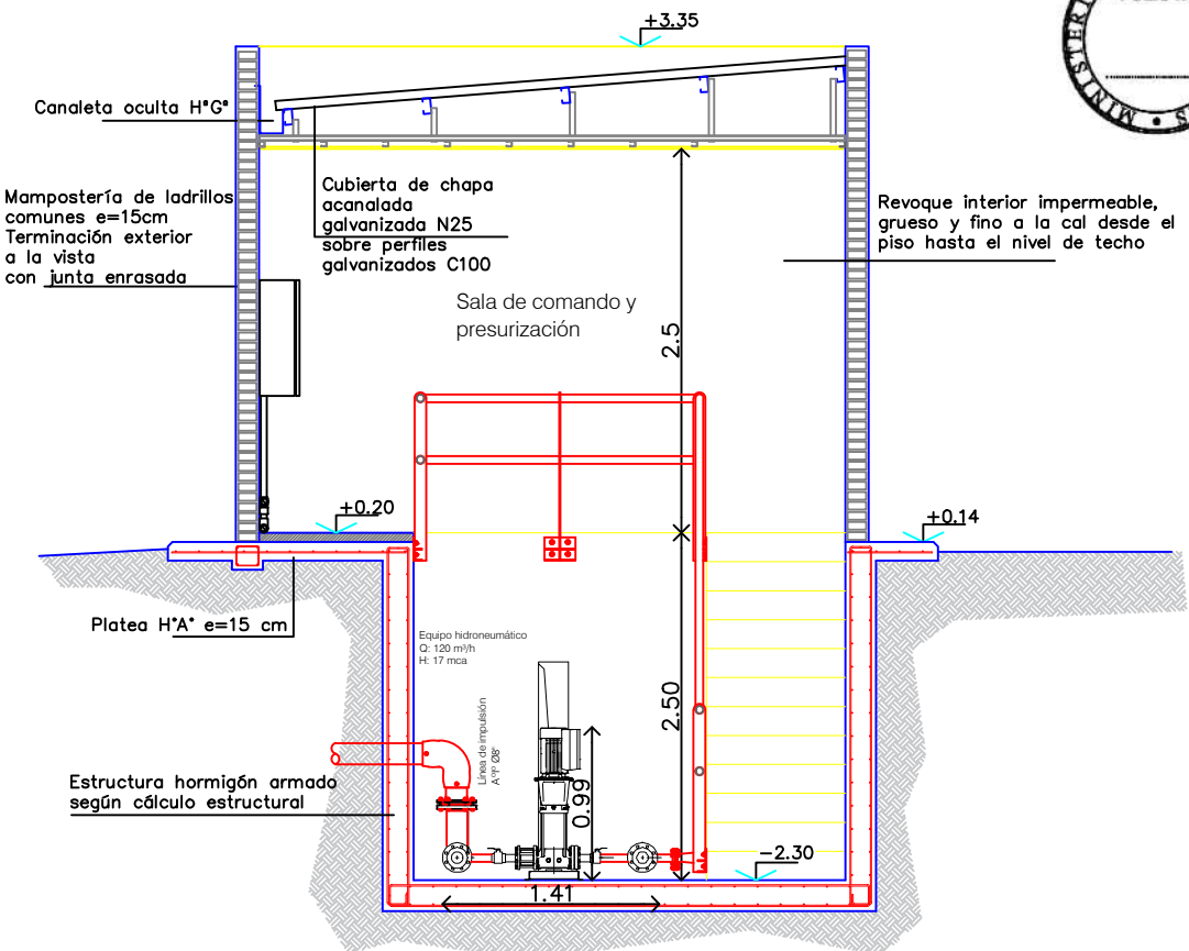
Corte B-B
