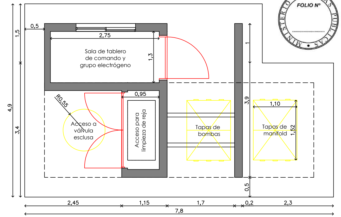
PLANTA DE ARQUITECTURA
