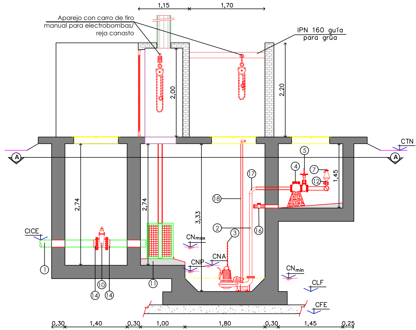
CORTE 1-1
