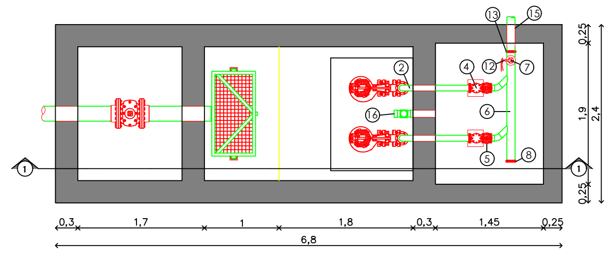
CORTE A-A
