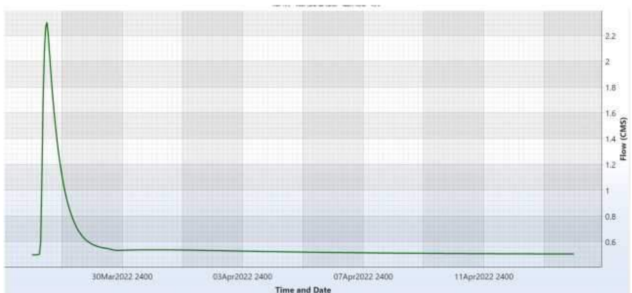
Figura 10: Hidrograma calculado a la salida del canal para 2 años de recurrencia.
