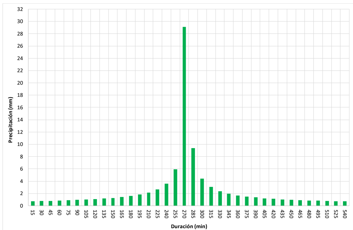
Figura 4: Hietograma de lluvia para una recurrencia de 5 años.
