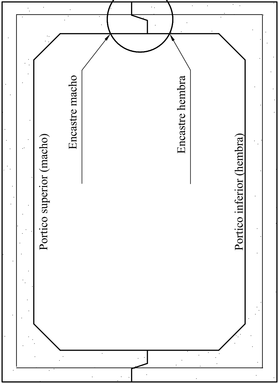
DETALLES SECCIÓN TRANSVERSAL DEL MÓDULO
