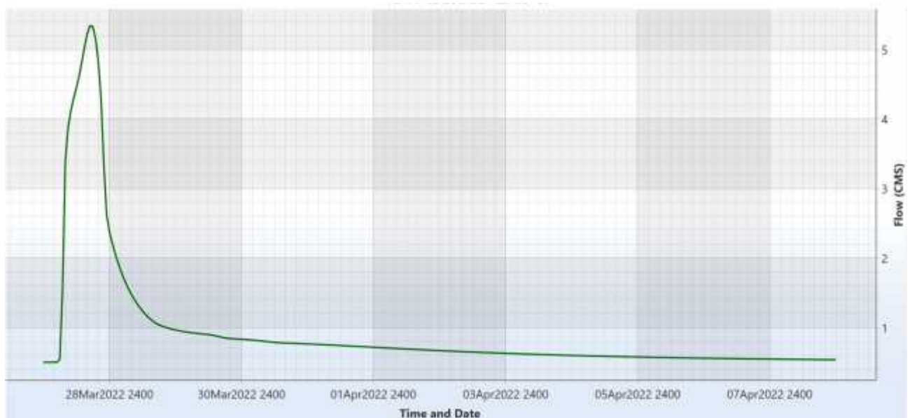
Figura 12: Hidrograma calculado a la salida del canal para 10 años de recurrencia.
