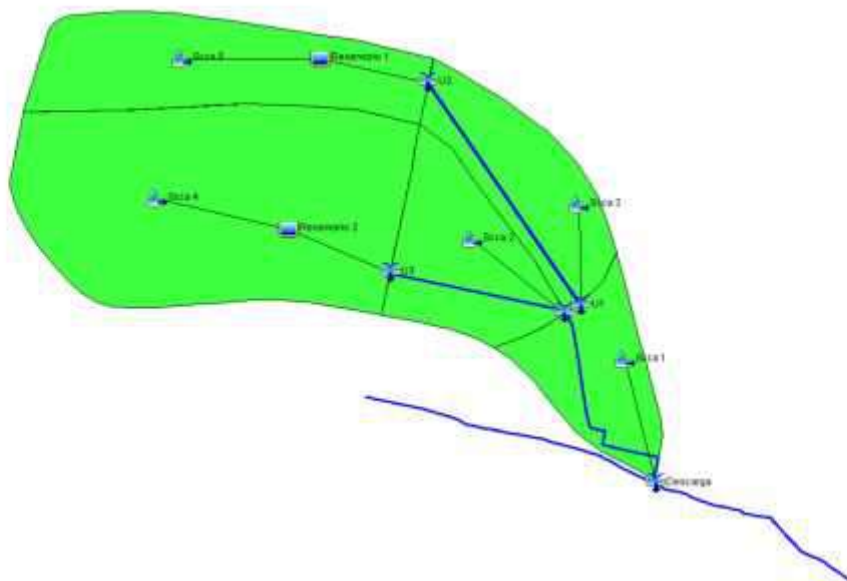
Figura 7: Esquema topológico del software HEC – HMS.
