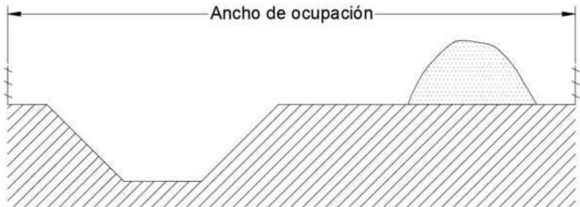
Figura 21: Ancho de ocupación tipo.
