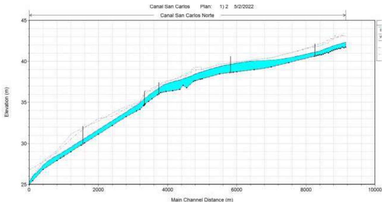
Figura 13: Perfil hidráulico del modelo HEC – RAS para 2 años de recurrencia.
