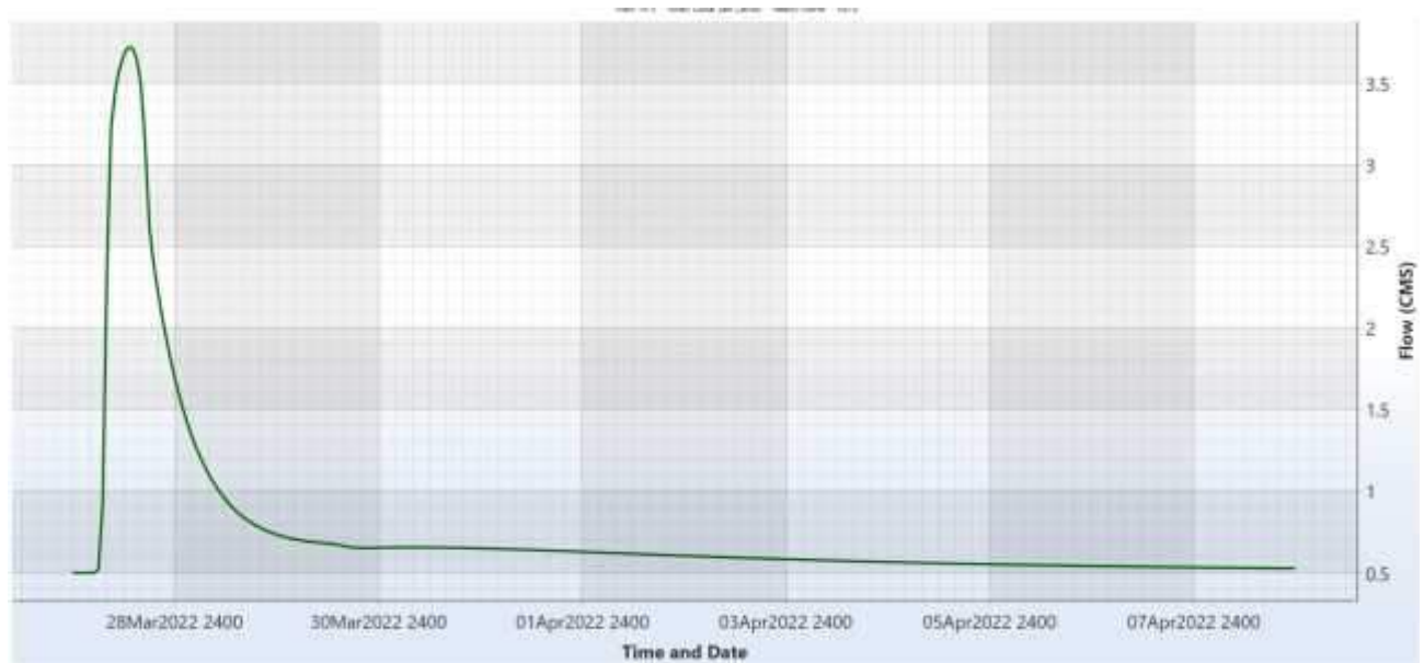
Figura 11: Hidrograma calculado a la salida del canal para 5 años de recurrencia.
