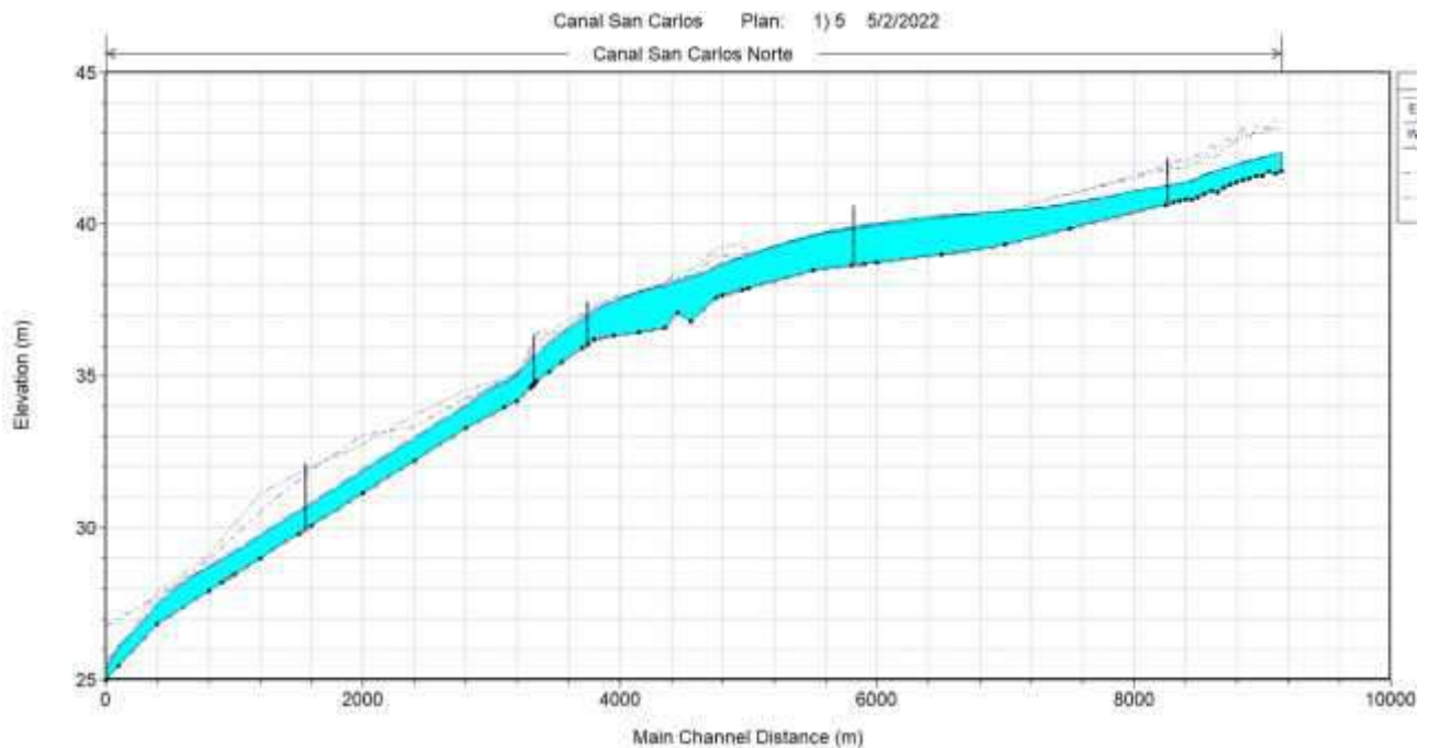
Figura 14: Perfil hidráulico del modelo HEC – RAS para 5 años de recurrencia.
