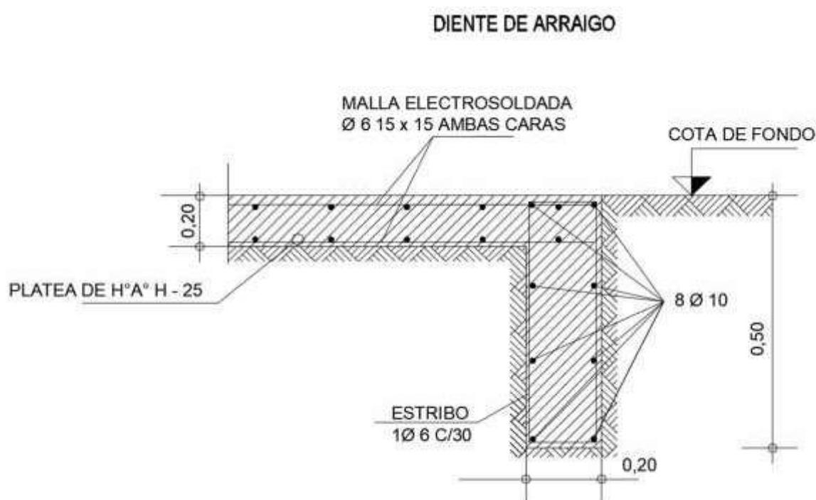
Figura 20: Detalle de platea y diente de arraigo a ejecutar a la entrada y salida de cada alcantarilla.
