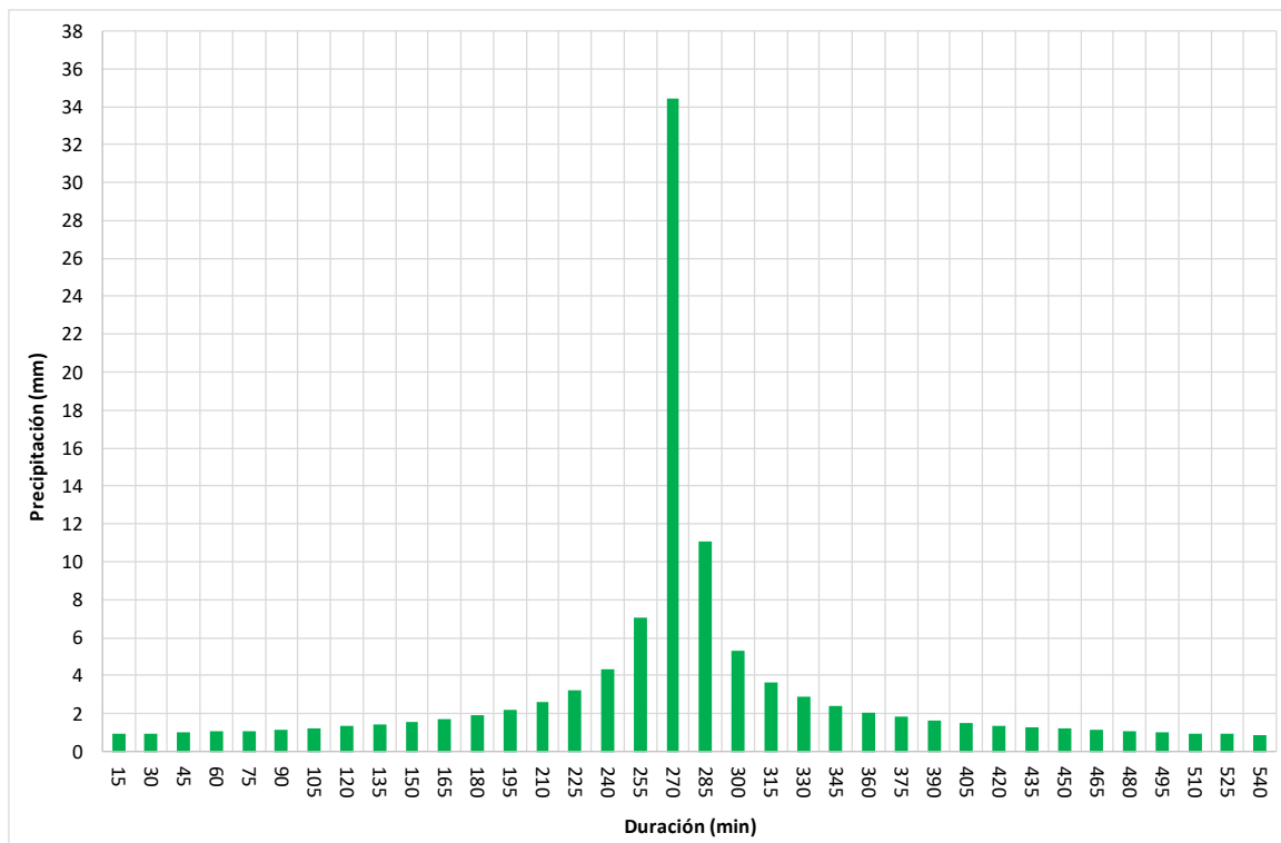
Figura 5: Hietograma de lluvia para una recurrencia de 10 años.
