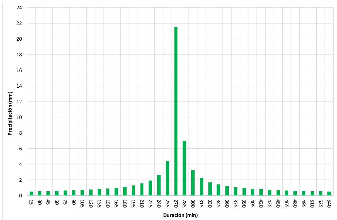
Figura 3: Hietograma de lluvia para una recurrencia de 2 años.
