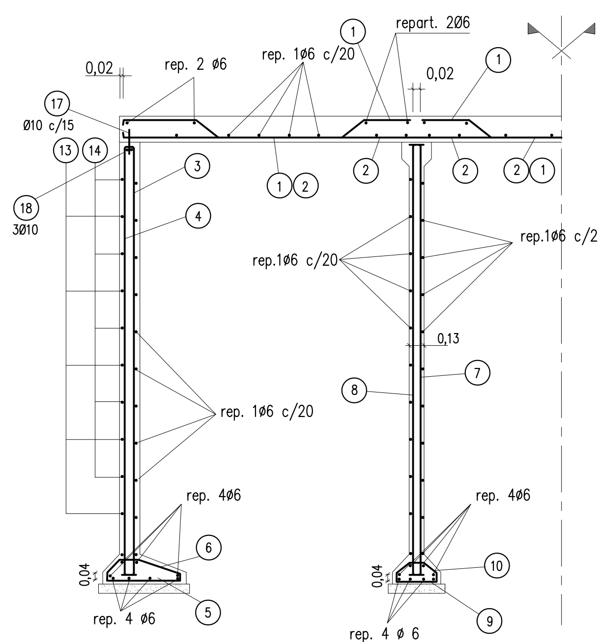
SECCION B-B
