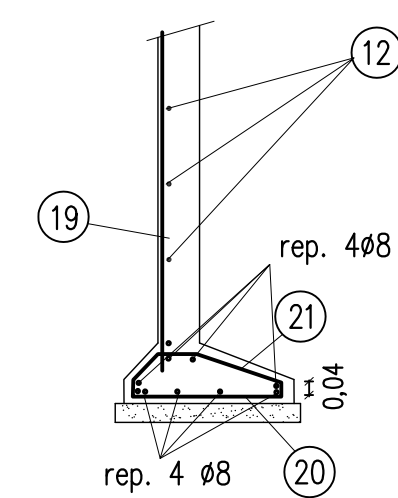
SECCION D-D
