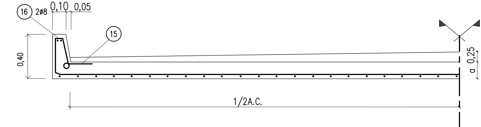
SEMI-SECCION C-C
