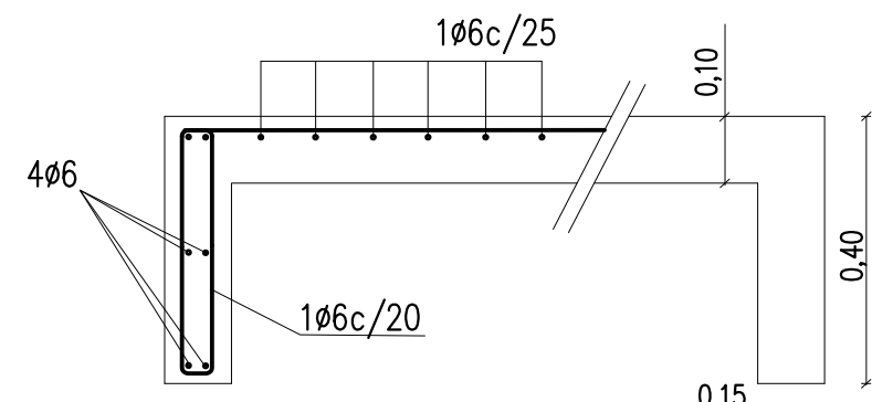
DETALLE PLATEA
