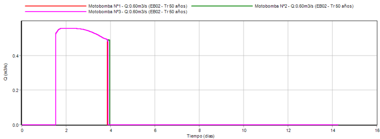
Figura N° 32: Caudal y tiempo de bombeo
