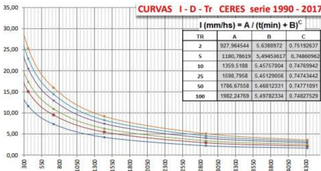
Figura N° 5: Curvas IDF de la Ciudad de Ceres (1990-2017).
