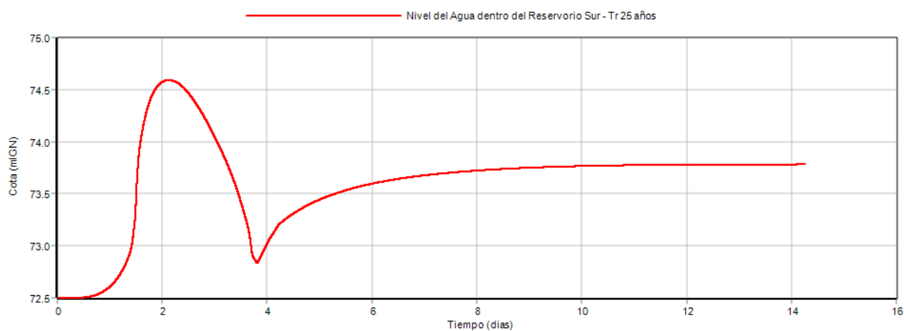
Figura N° 27: Variación de nivel dentro del reservorio para un tr de 25 años – nivel máximo disponible del reservorio 74.7 mIGN
