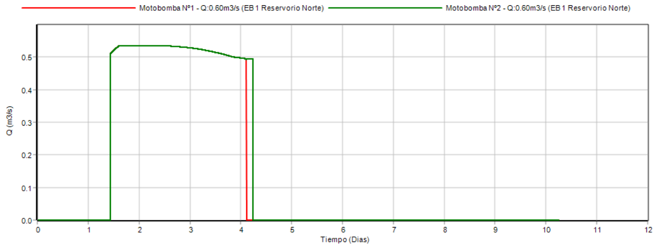
Figura N° 30: Caudal y tiempo de bombeo.
