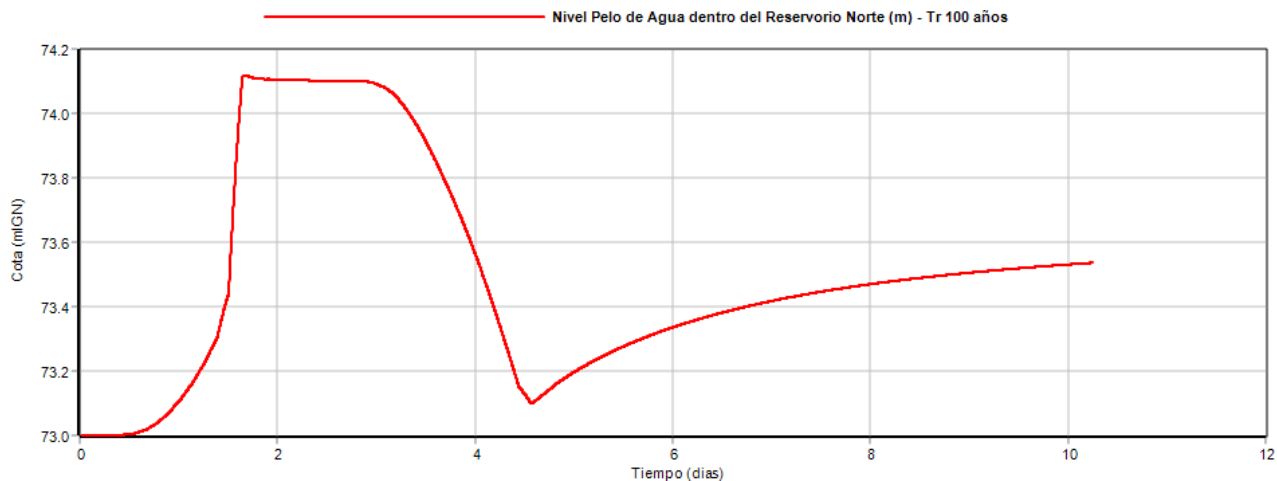
Figura N° 33: Variación de nivel dentro del reservoirio Norte para un tr de 100 años – nivel máximo disponible del reservoirio 74.3 mIGN
