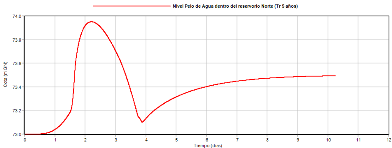
Figura N° 21: Variación de nivel dentro del reservorio para un tr de 5 años – nivel máximo disponible del reservorio 74.3 mIGN
