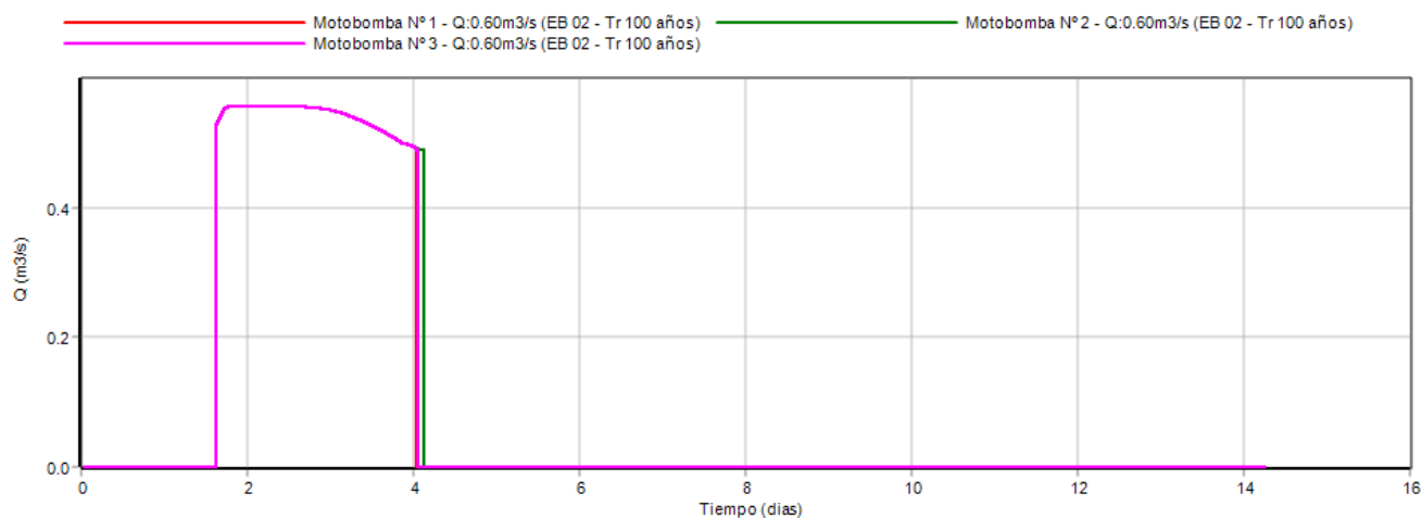
Figura N° 36: Caudal y tiempo de bombeo
