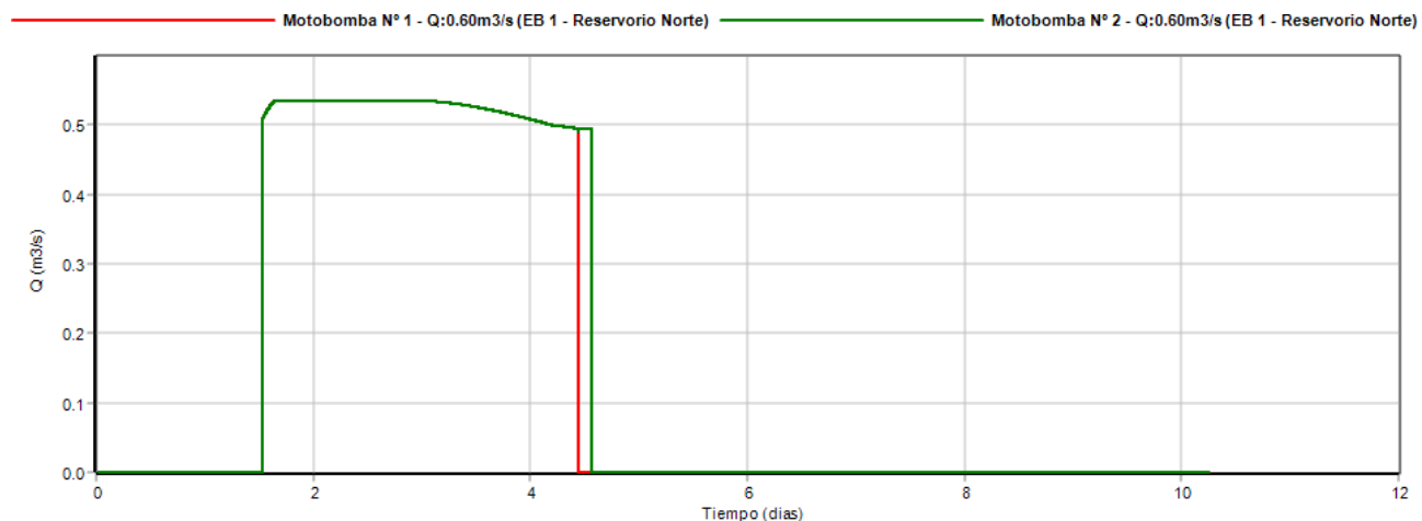
Figura N° 34: Caudal y tiempo de bombeo.
