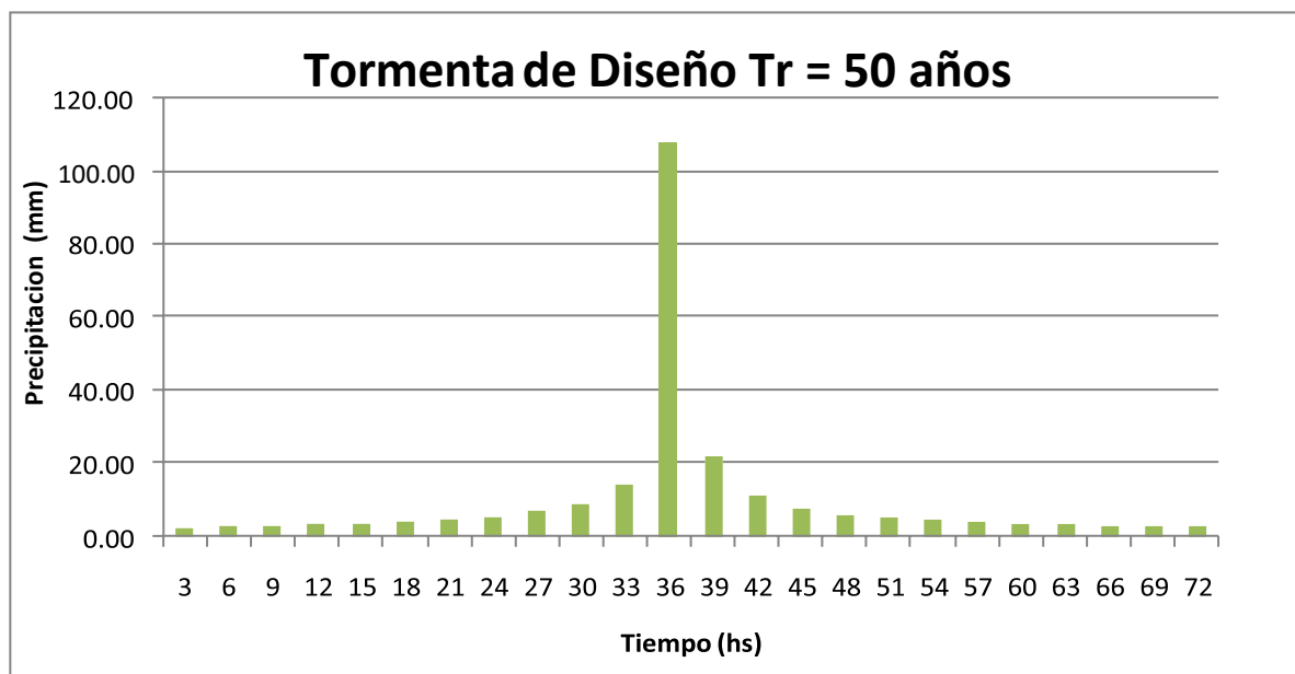
Figura N° 9: Tormenta para 3 días de duración y Tr: 50 años de recurrencia. Precipitación acumulada 245.85 mm
