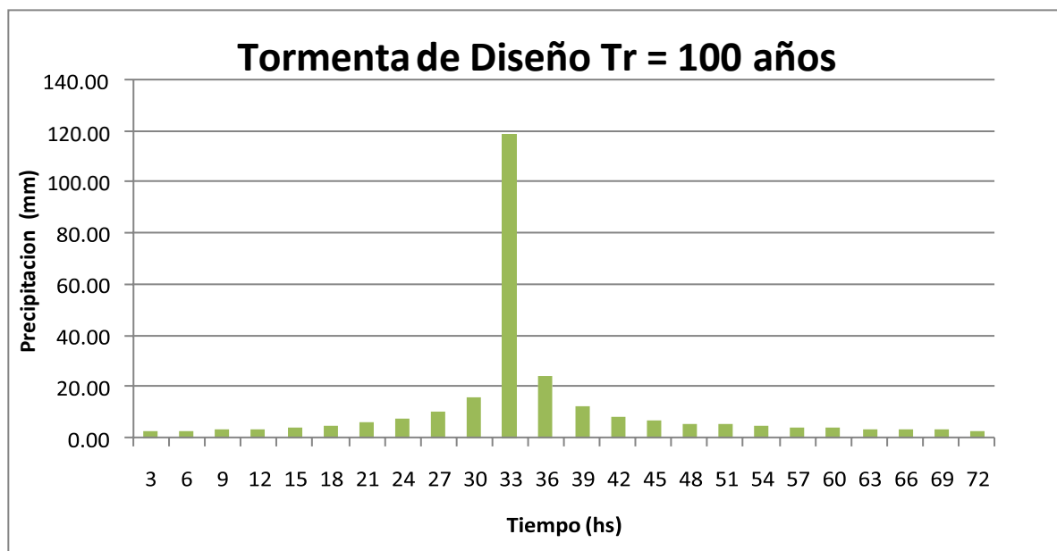
Figura N° 10: Tormenta para 3 días de duración y Tr: 100 años de recurrencia. Precipitación acumulada 271.48mm
