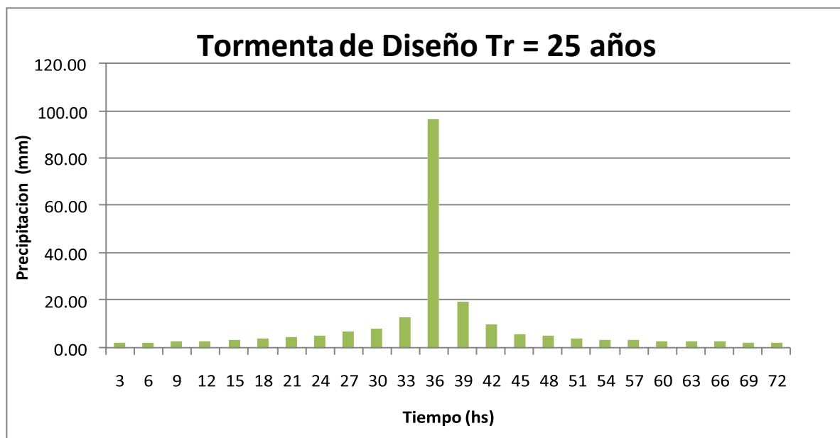
Figura N° 8: Tormenta para 3 días de duración y Tr: 25 años de recurrencia. Precipitación acumulada 220.51 mm
