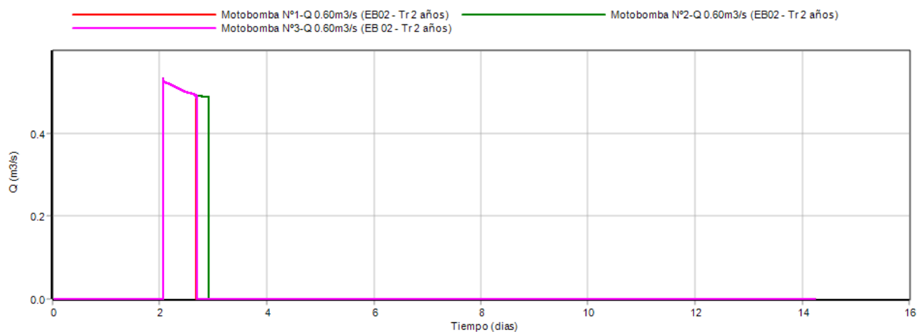
Figura N° 20: Caudal y tiempo de bombeo
