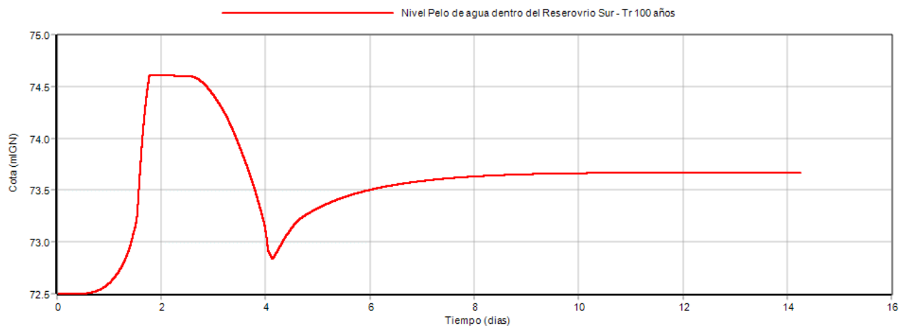
Figura N° 35: Variación de nivel dentro del reservorio Sur para un tr de 100 años – nivel máximo disponible del reservorio 74.7 mIGN
