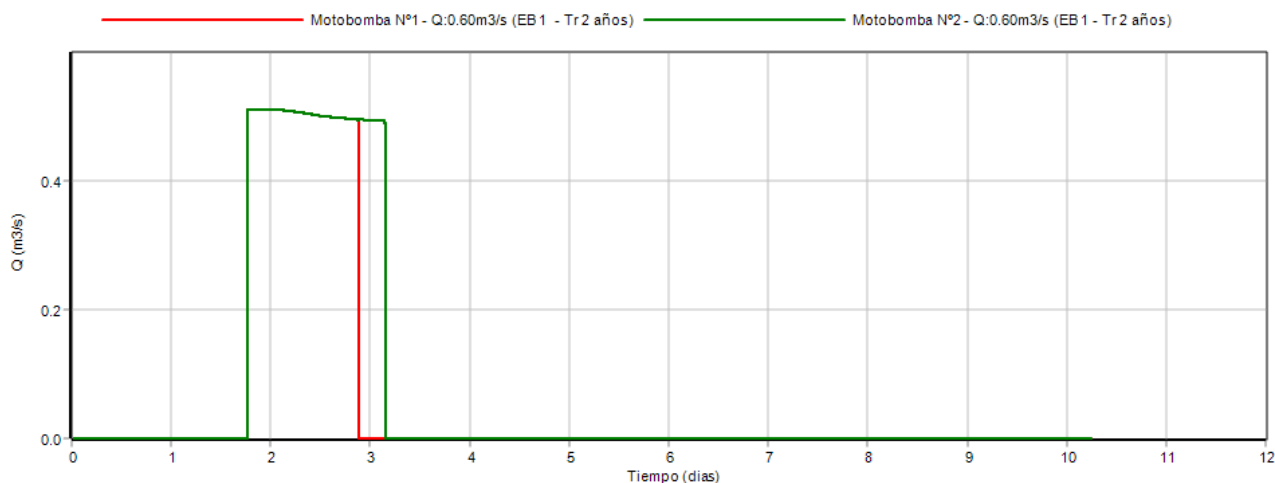
Figura N° 18: Caudal y tiempo de bombeo.
