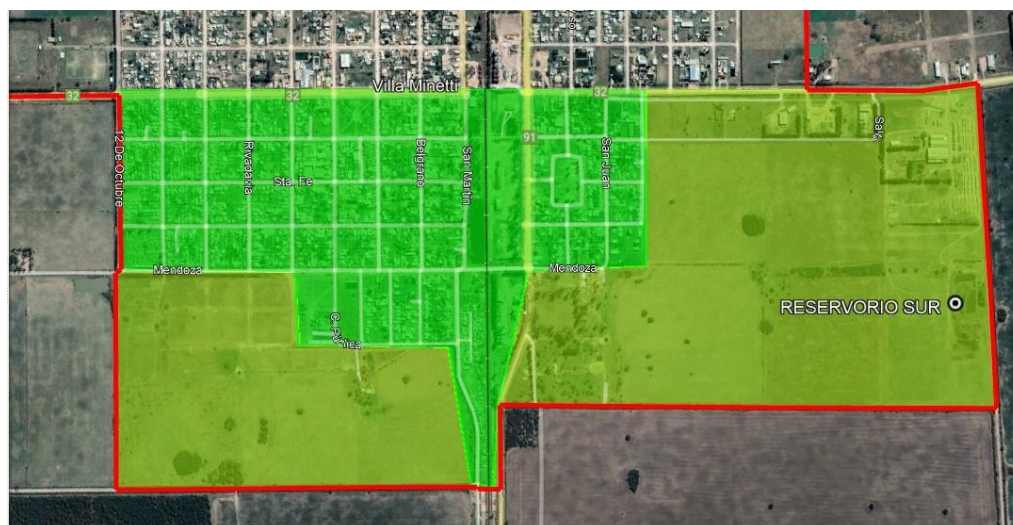
Figura N° 13: Discretización del área de estudio – Sector Sur
