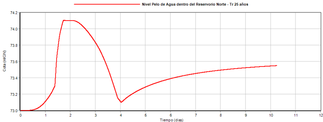
Figura N° 25: Variación de nivel dentro del reservorio para un tr de 25 años – nivel máximo disponible delreservorio 74.3 mIGN
