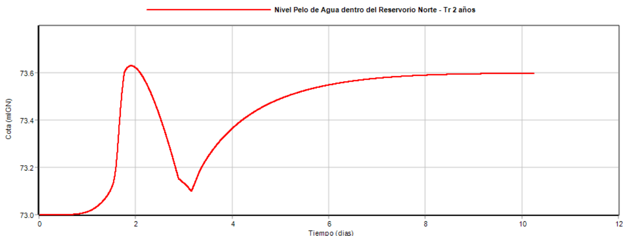
Figura N° 17: Variación de nivel dentro del reservorio para un tr de 2 años – nivel máximo disponible del reservorio 74.3 mIGN
