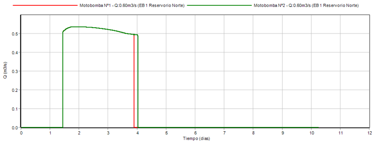
Figura N° 26: Caudal y tiempo de bombeo.
