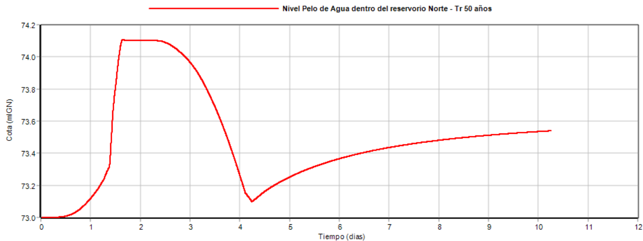
Figura N° 29: Variación de nivel dentro del reservorio para un Tr de 50 años – nivel máximo disponible del reservorio 74.3 mIGN
