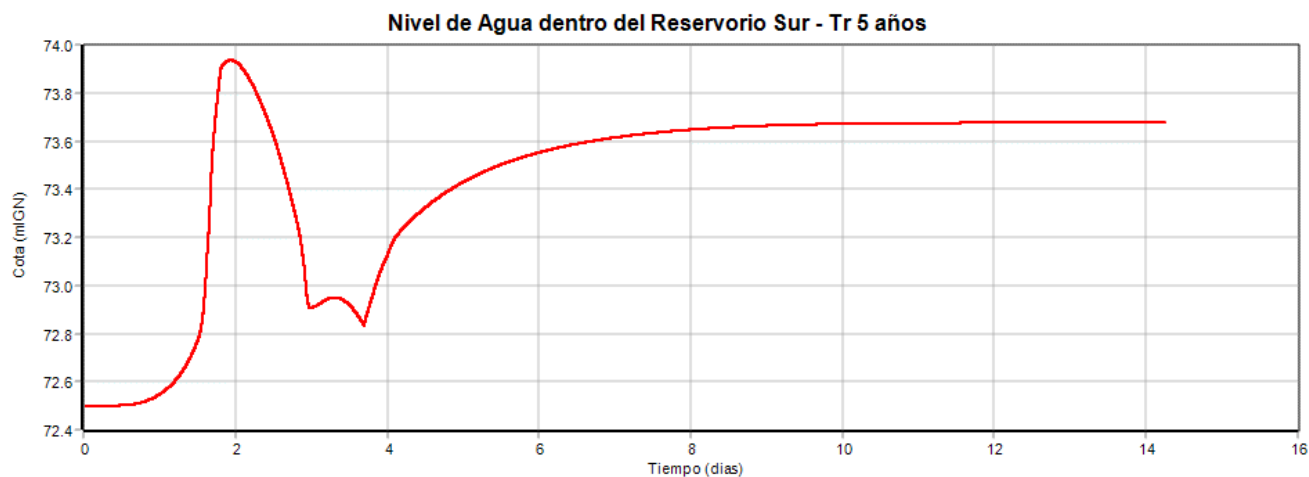
Figura N° 23: Variación de nivel dentro del reservorio para un tr de 5 años – nivel máximo disponible del reservorio 74.7 mIGN
