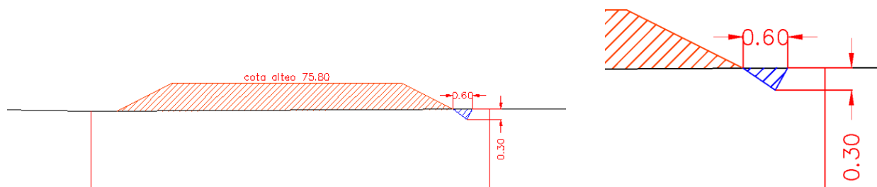
Figura N° 37: Esquema de cuneta perimetral interna de terraplén.
