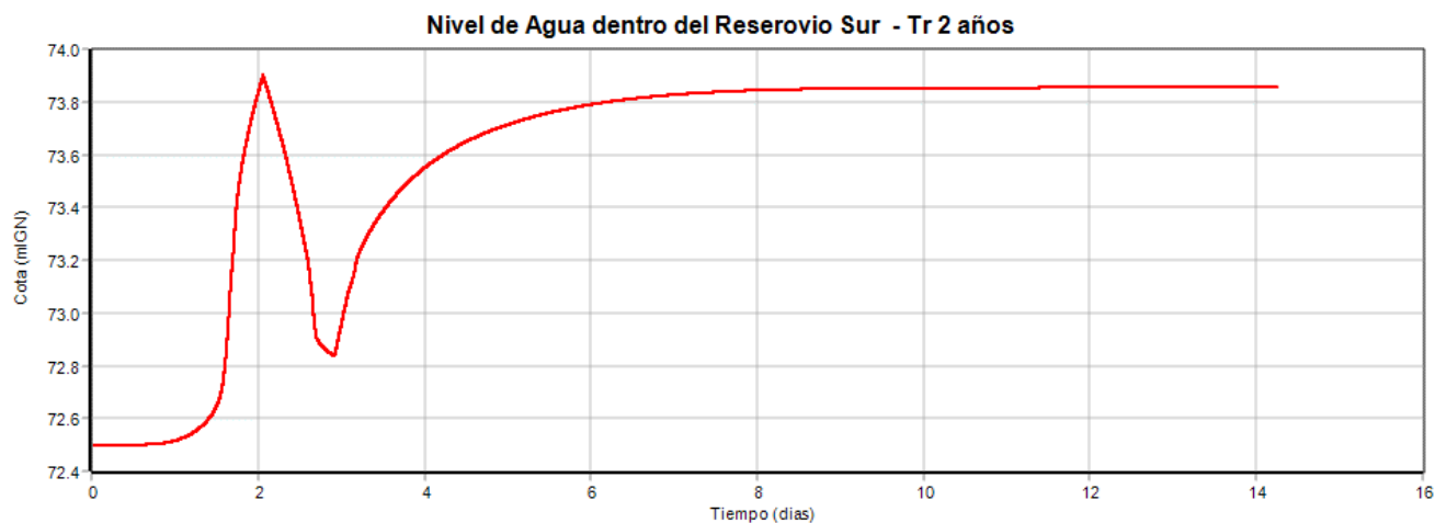
Figura N° 19: Variación de nivel dentro del reservorio para un tr de 2 años – nivel máximo disponible del reservorio 74.7 mIGN
