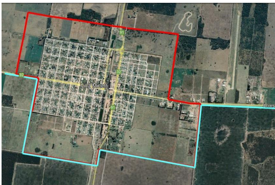
Figura N° 38: Trazo Canal Exterior Sur (existente)
