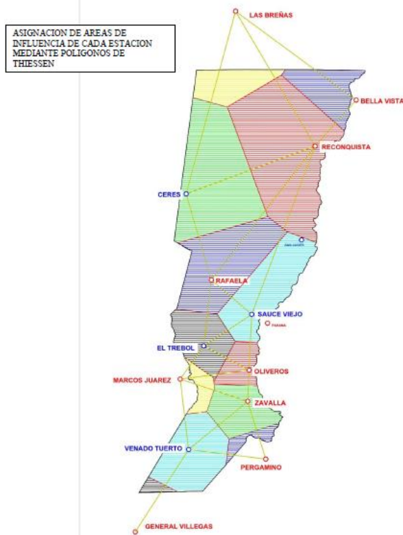
Figura N° 4: Polígonos de Thiessen – Distribución de Estaciones
