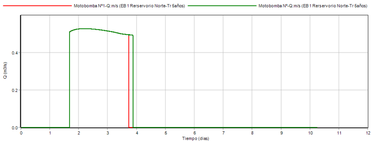
Figura N° 22: Caudal y tiempo de bombeo.
