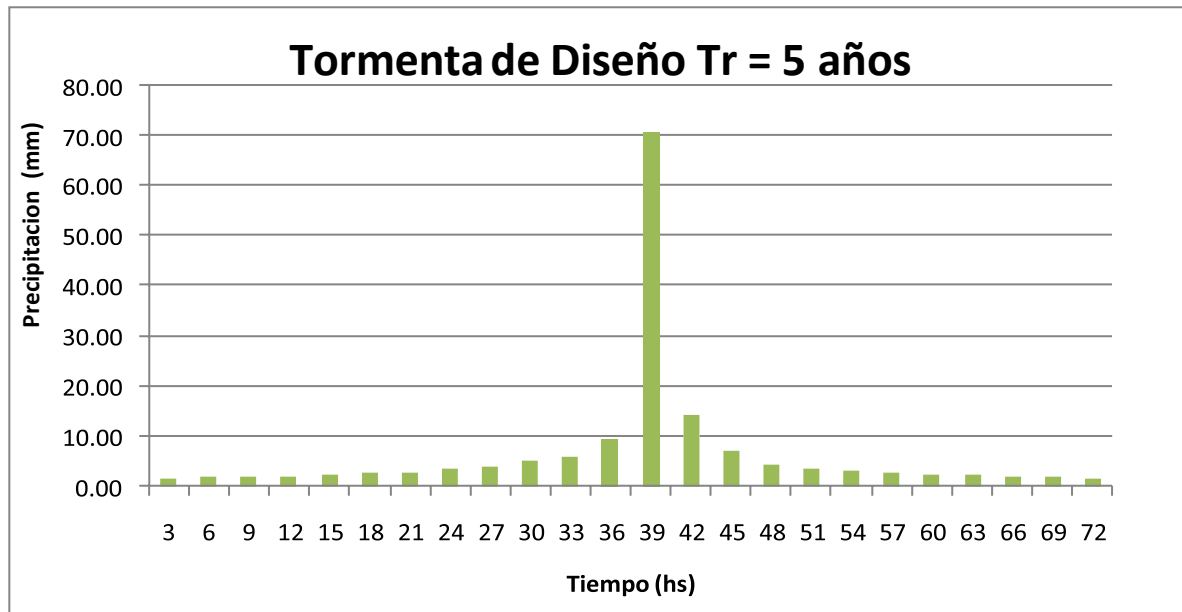
Figura N° 7: Tormenta para 3 días de duración y Tr: 5 años de recurrencia. Precipitación acumulada 161.26 mm
