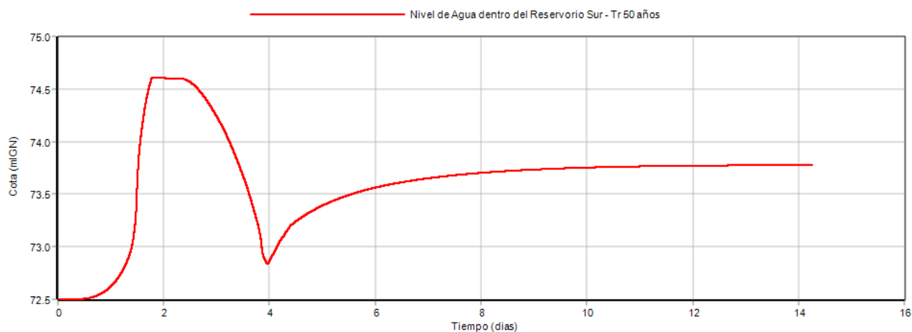
Figura N° 31: Variación de nivel dentro del reservorio para un tr de 50 años – nivel máximo disponible del reservorio 74.7 mIGN
