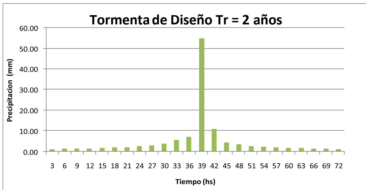
Figura N° 6: Tormenta para 3 días de duración y Tr: 2 años de recurrencia. Precipitación acumulada 123.26 mm
