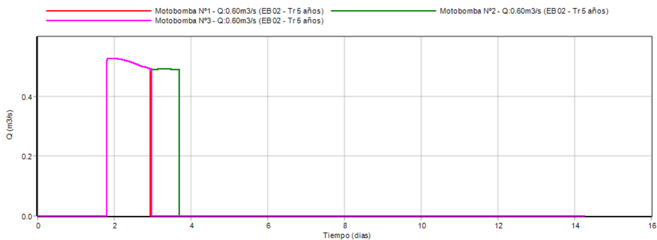
Figura N° 24: Caudal y tiempo de bombeo
