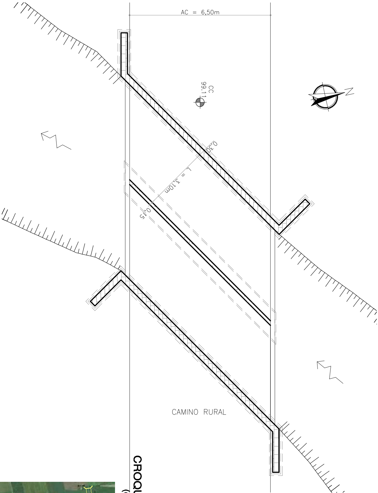
PLANTA
