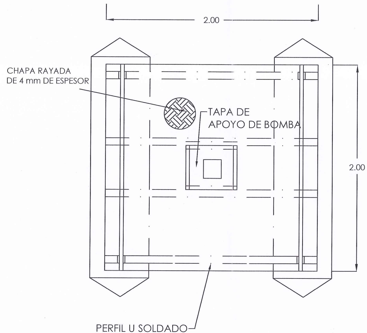
DETALLE PLANTA
