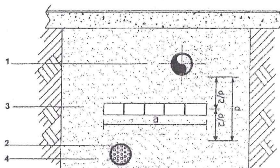
Figura 2a Protección con ladrillos Paralelismo
