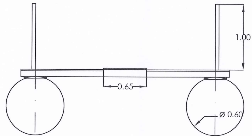
VISTA ANTERIOR PONTÓN
