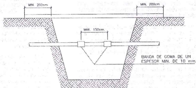
SUSPENSION DE UNA CAÑERÍA
