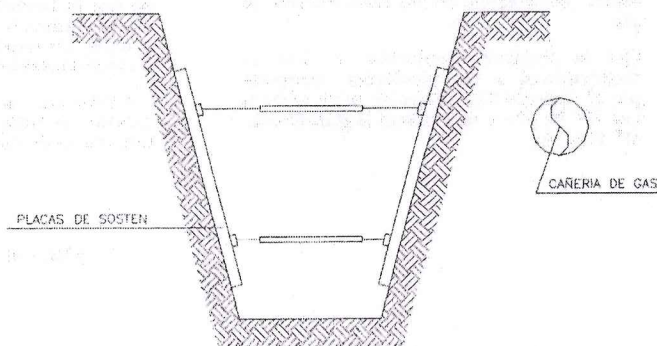
REFUERZO SOBRE PAREDES DE LA ZANJA
