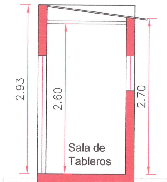
CORTE A-A
