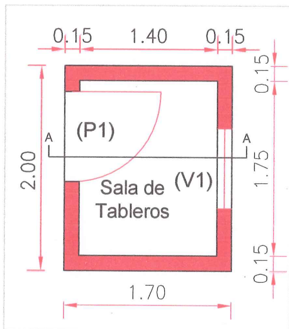
PLANTA
