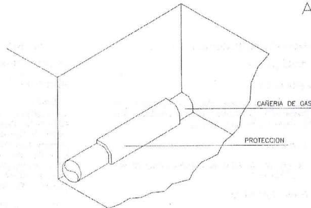
PROTECCION CON CAMISA
