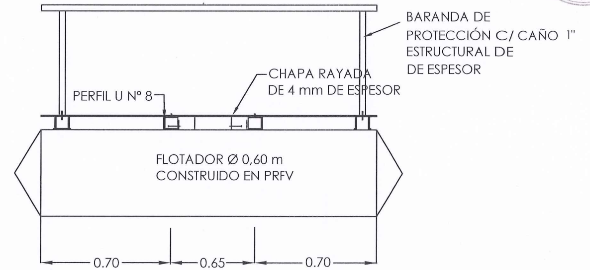
VISTA LATERAL DERECHA
