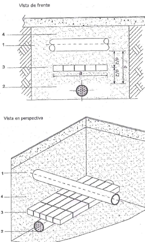
Figura 2b Protección con ladrillos Cruce
