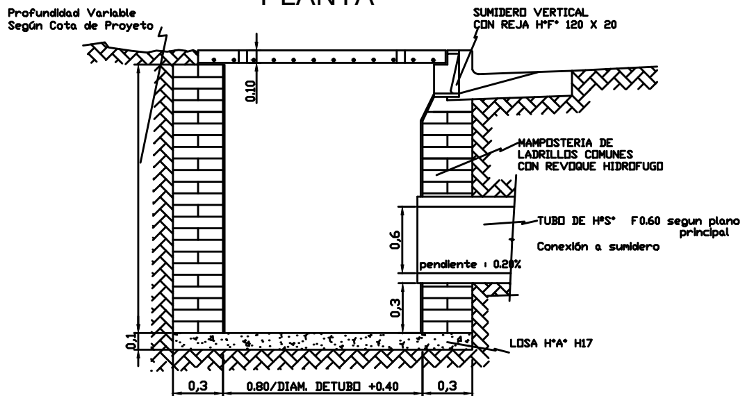
CORTE A-A
