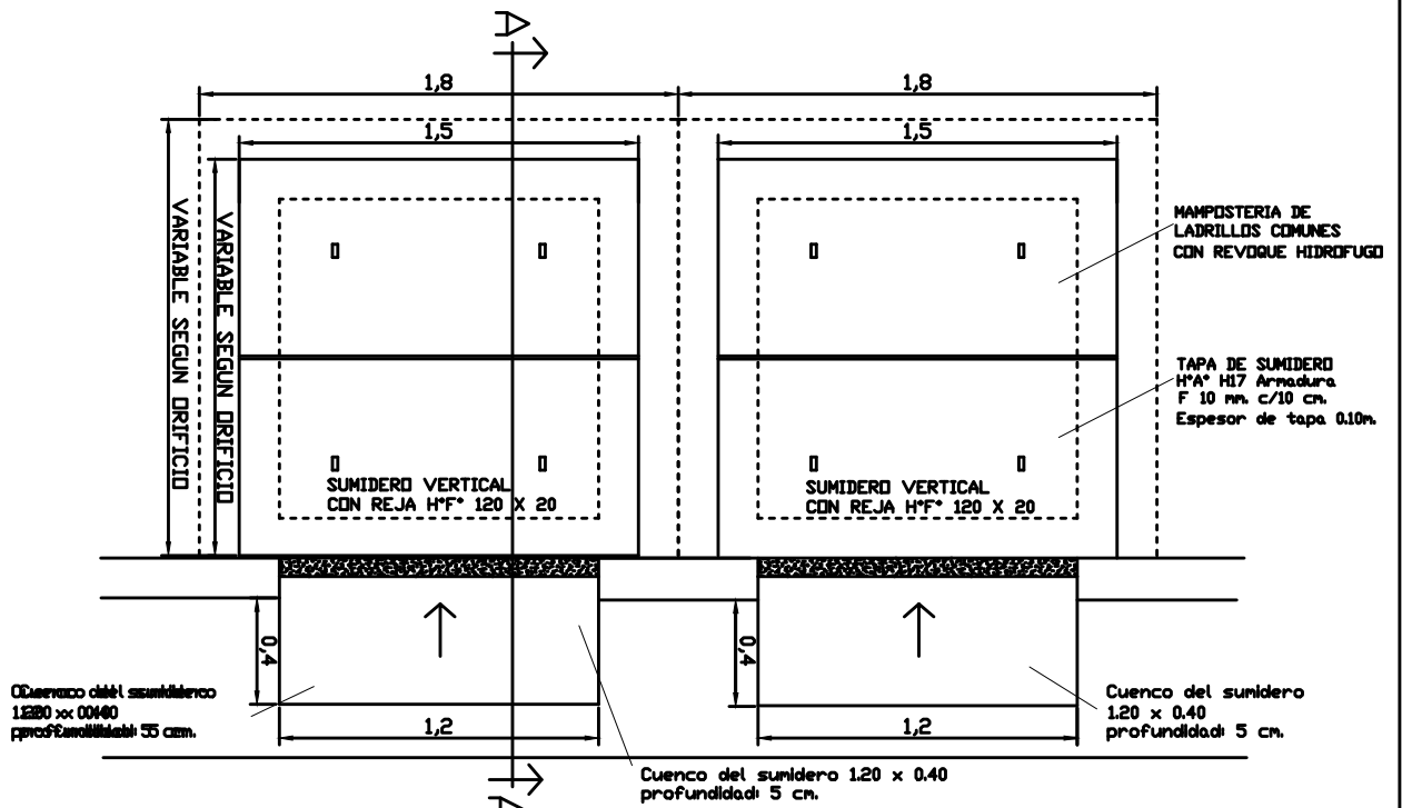
PLANTA
