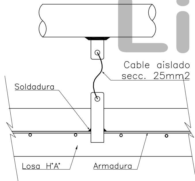
DETALLE 4 CONEXION EQUIPOTENCIAL ENTRE ARMADURA LOSA H°A° Y CAÑERIA AEREA
