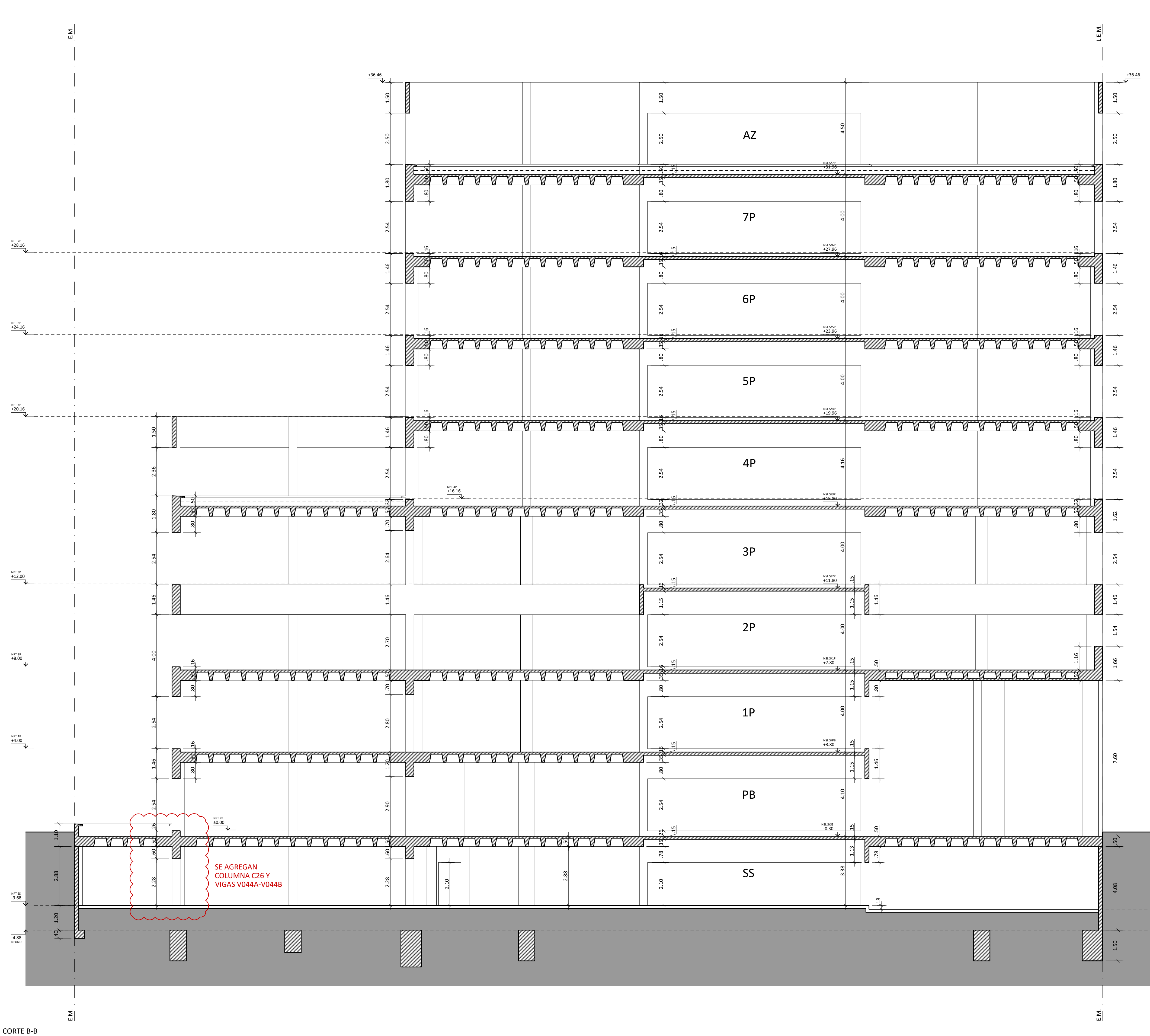
CORTE B-B
