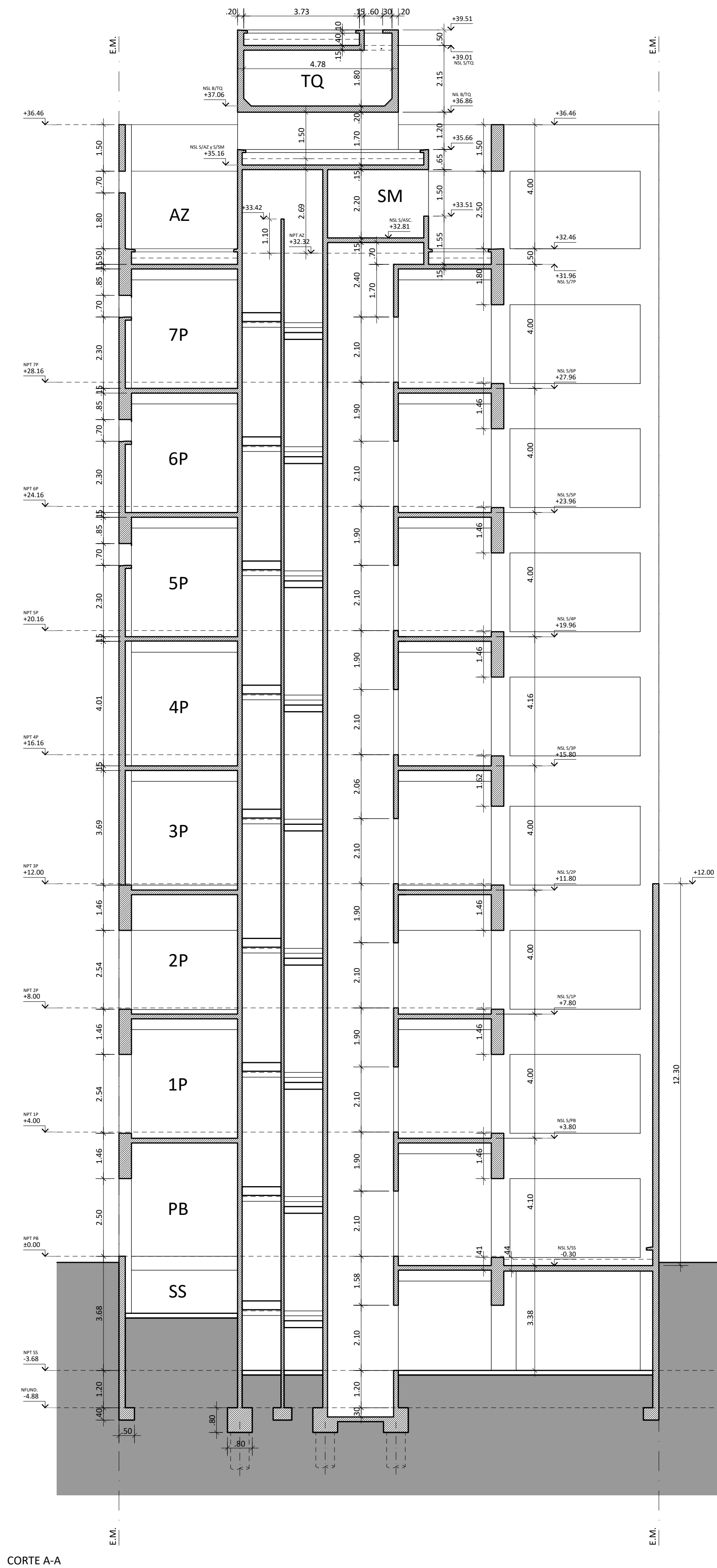
CORTE A-A
