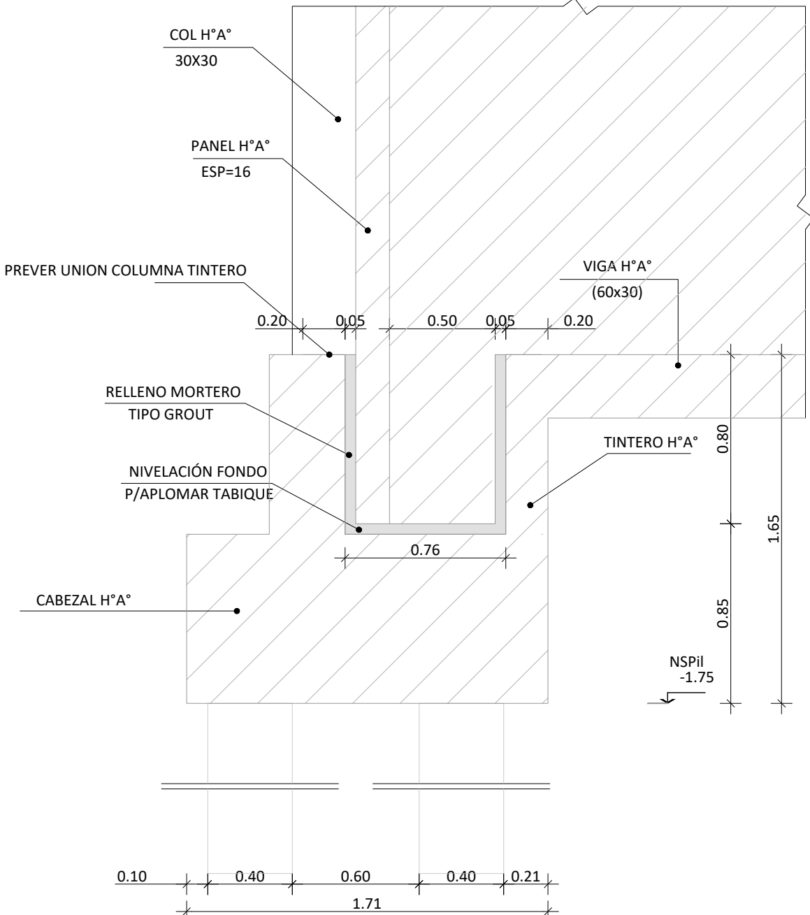
DETALLE - FUNDACIONES B06 - ESC 1.25
