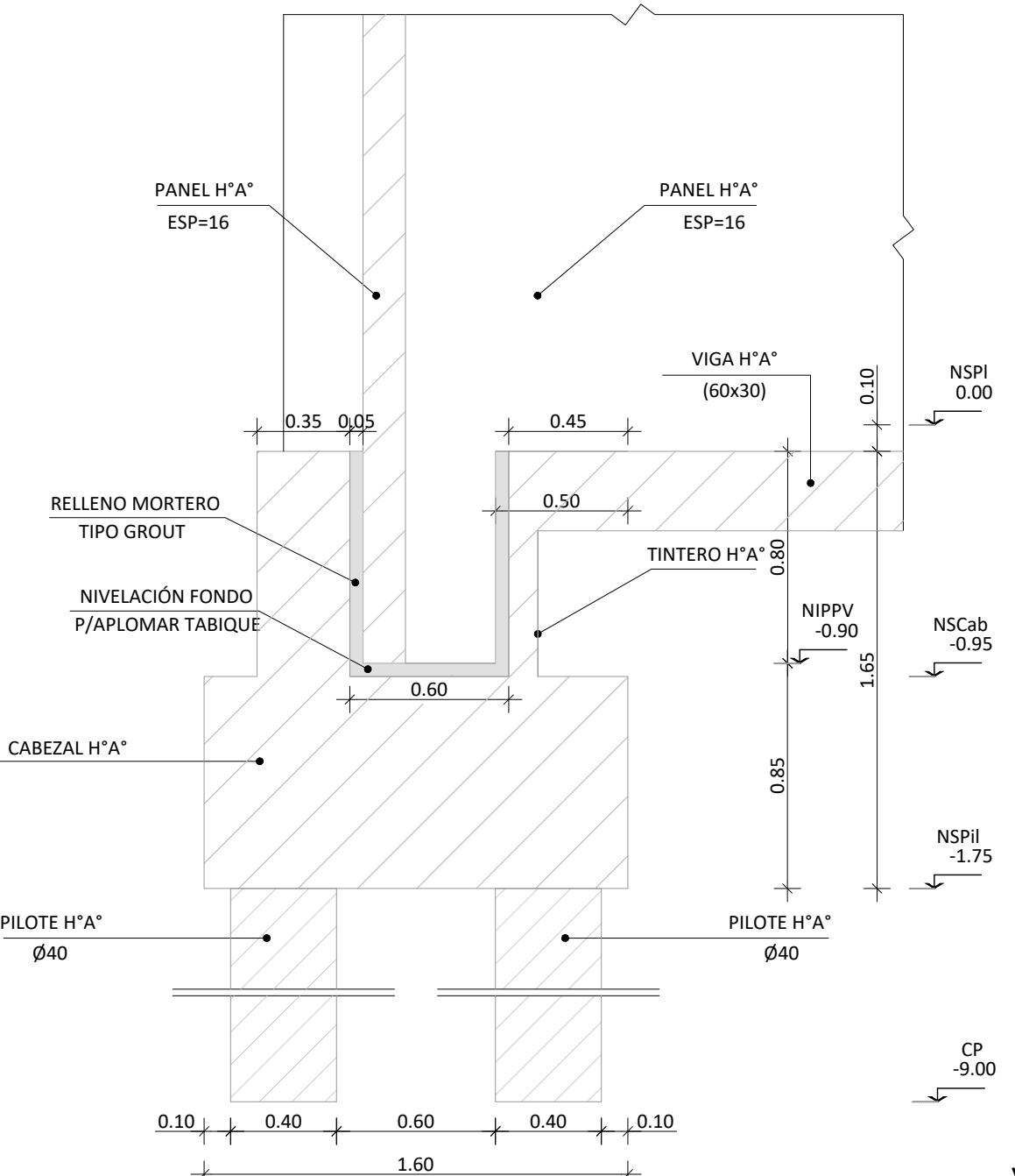
DETALLE - FUNDACIONES B08 - ESC 1.25
