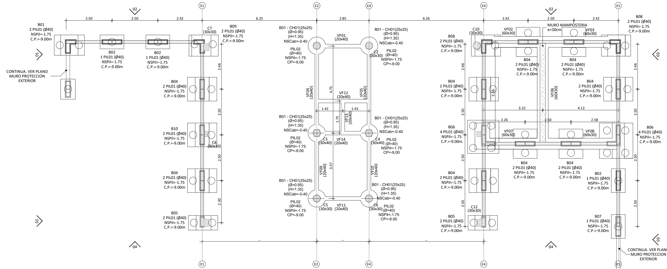
PLANTA DE FUNDACIONES
