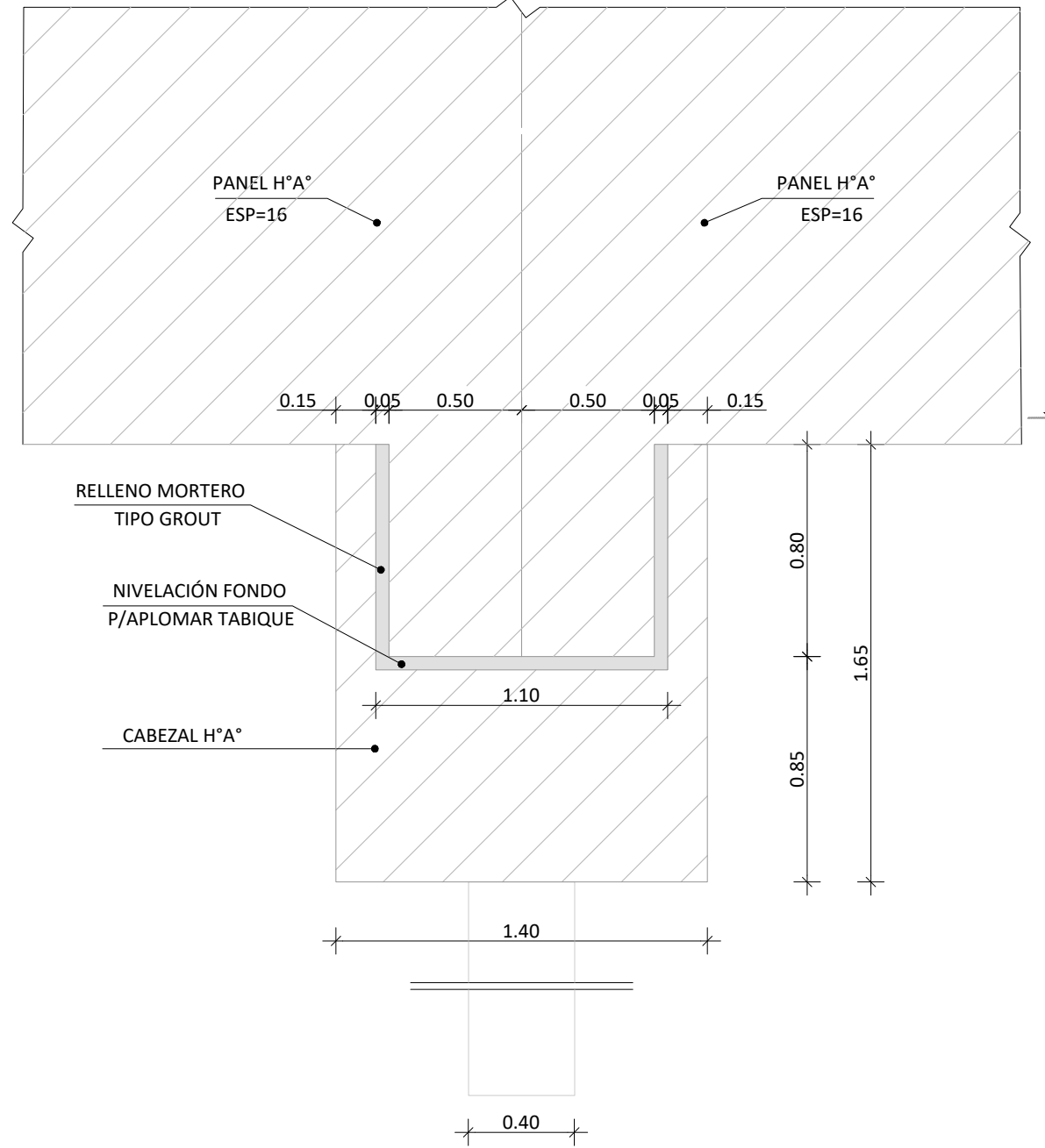
DETALLE - FUNDACIONES B02 - ESC 1.25
