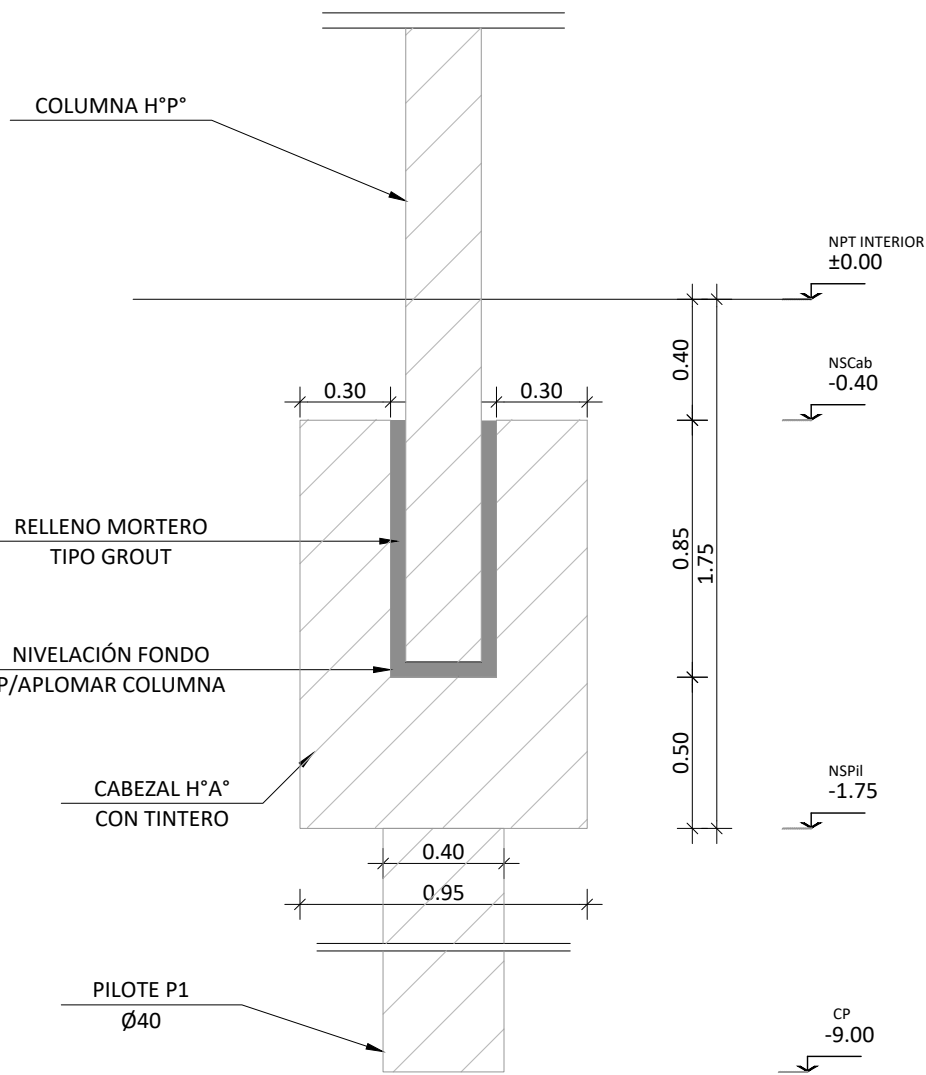
DETALLE - FUNDACIONES B08 - ESC 1.25
