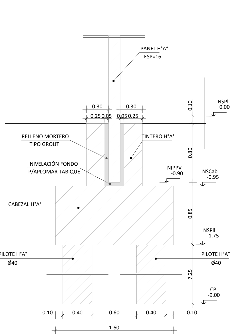
DETALLE - FUNDACIONES B04 - ESC 1.25
