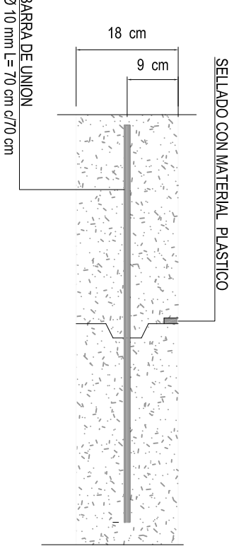
JUNTA LONG. DE CONSTRUCCION TIPO ENSAMBLADA
