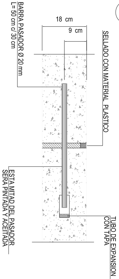
JUNTA TRANSVERSAL DE EXPANSION
