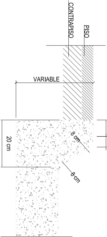
DISEÑO DE CORDONES PERFIL CORDON TIPO
