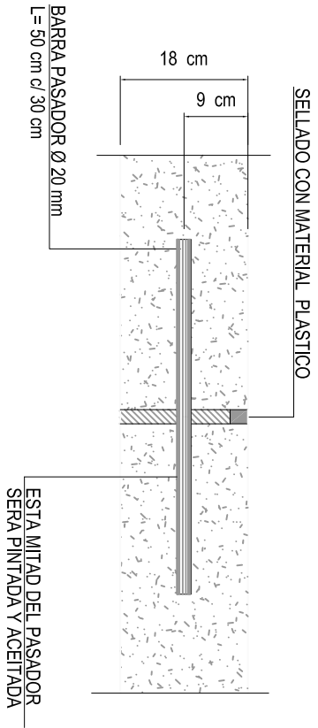
JUNTA TRANSVERSAL DE CONTRACCION TIPO SIMULADA
