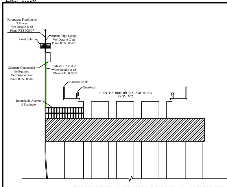
Corte A-A Esc.: 1:100
