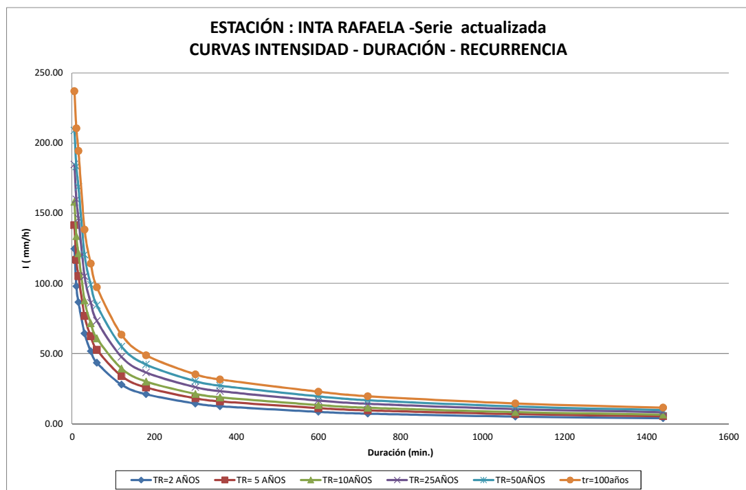
Imagen 4: Curvas I – D – F - Rafaela
