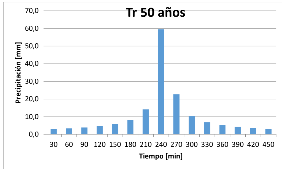
Imagen 9: Hietograma de diseño para 50 años de recurrencia obtenidos de la IDF de Rafaela.
