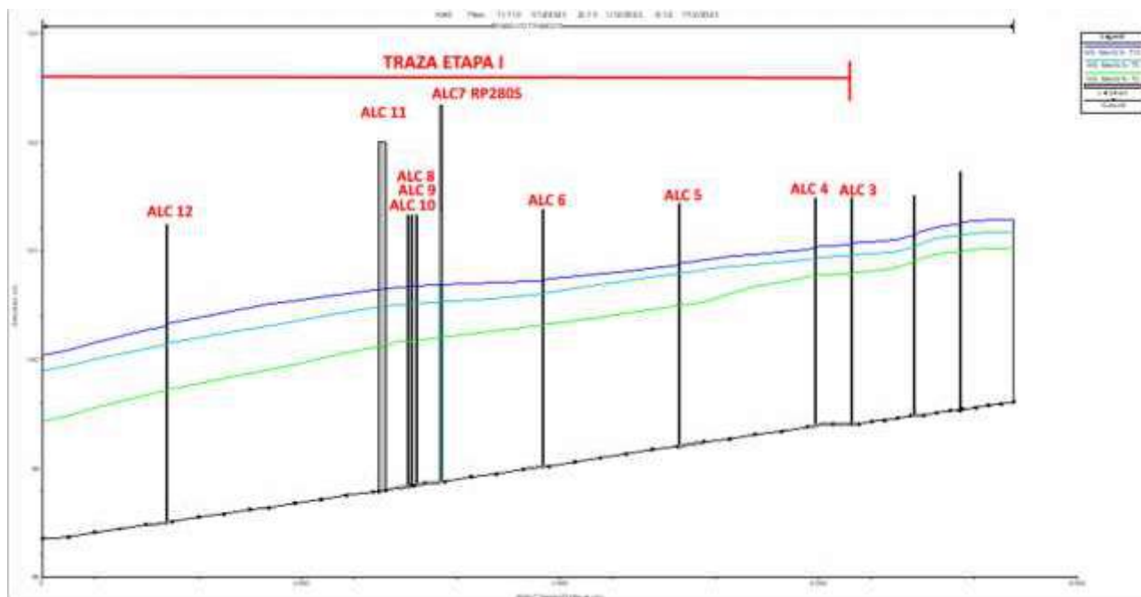
Imagen 14: Perfil longitudinal canal perimetral Eusebia y Carolina.
