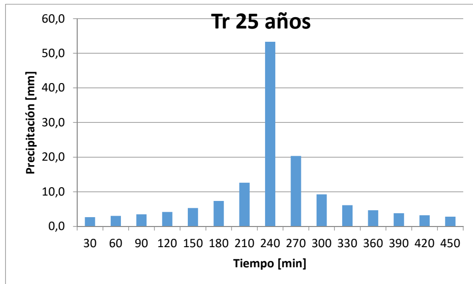
Imagen 8: Hietograma de diseño para 25 años de recurrencia obtenidos de la IDF de Rafaela.
