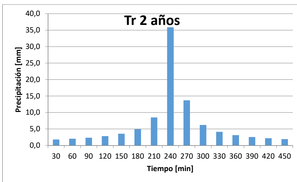
Imagen 5: Hietogramas de diseño para 2 años de recurrencia obtenidos de la IDF de Rafaela.
