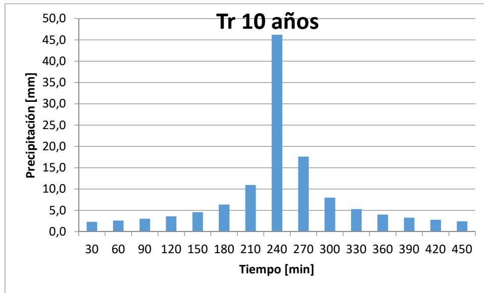
Imagen 7: Hietogramas de diseño para 10 años de recurrencia obtenidos de la IDF de Rafaela.
