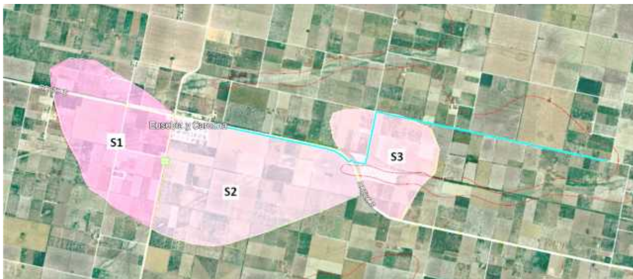
Imagen 3 -Subcuencas de aporte.
