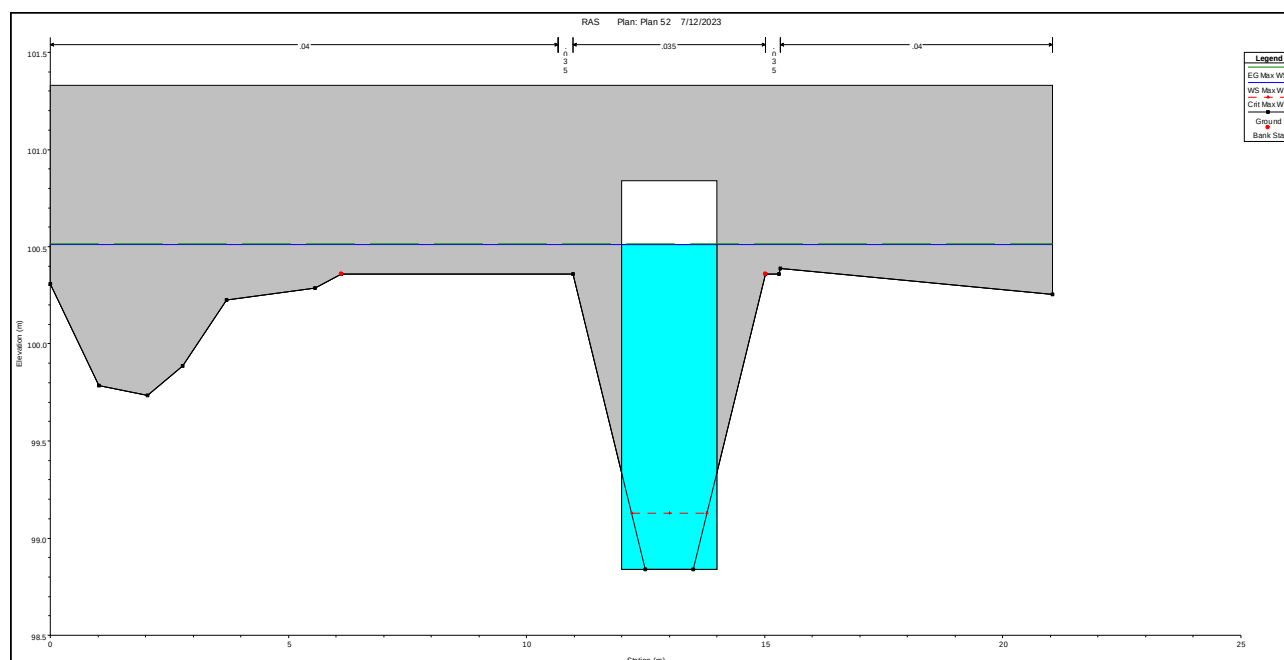
Imagen 13: Canal perimetral Eusebia y Carolina. A8 - Alcantarilla de cruce en camino comunal. Prog. 2857.10 m. Recurrencia de verificación, TR 5 años.
