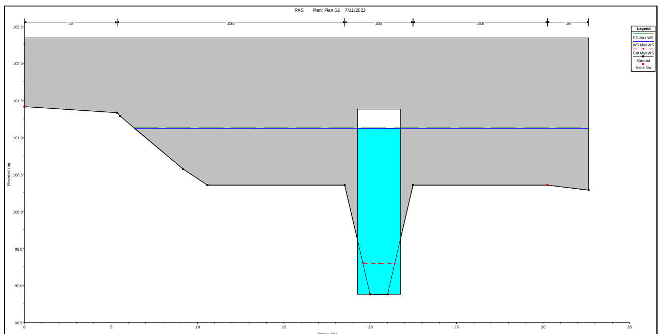
Imagen 12: Canal perimetral Eusebia y Carolina. A7 - Alcantarilla de cruce en RP280-S. Prog. 3047 m. Recurrencia de verificación, TR 50 años.
