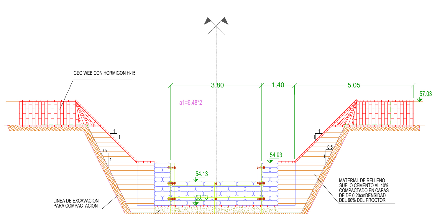
Seccion III - III
