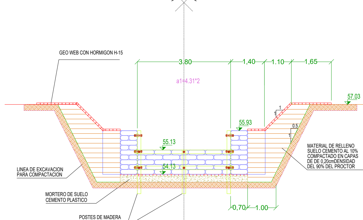
Seccion V - V
