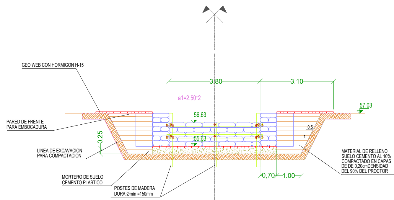
Seccion II - II
