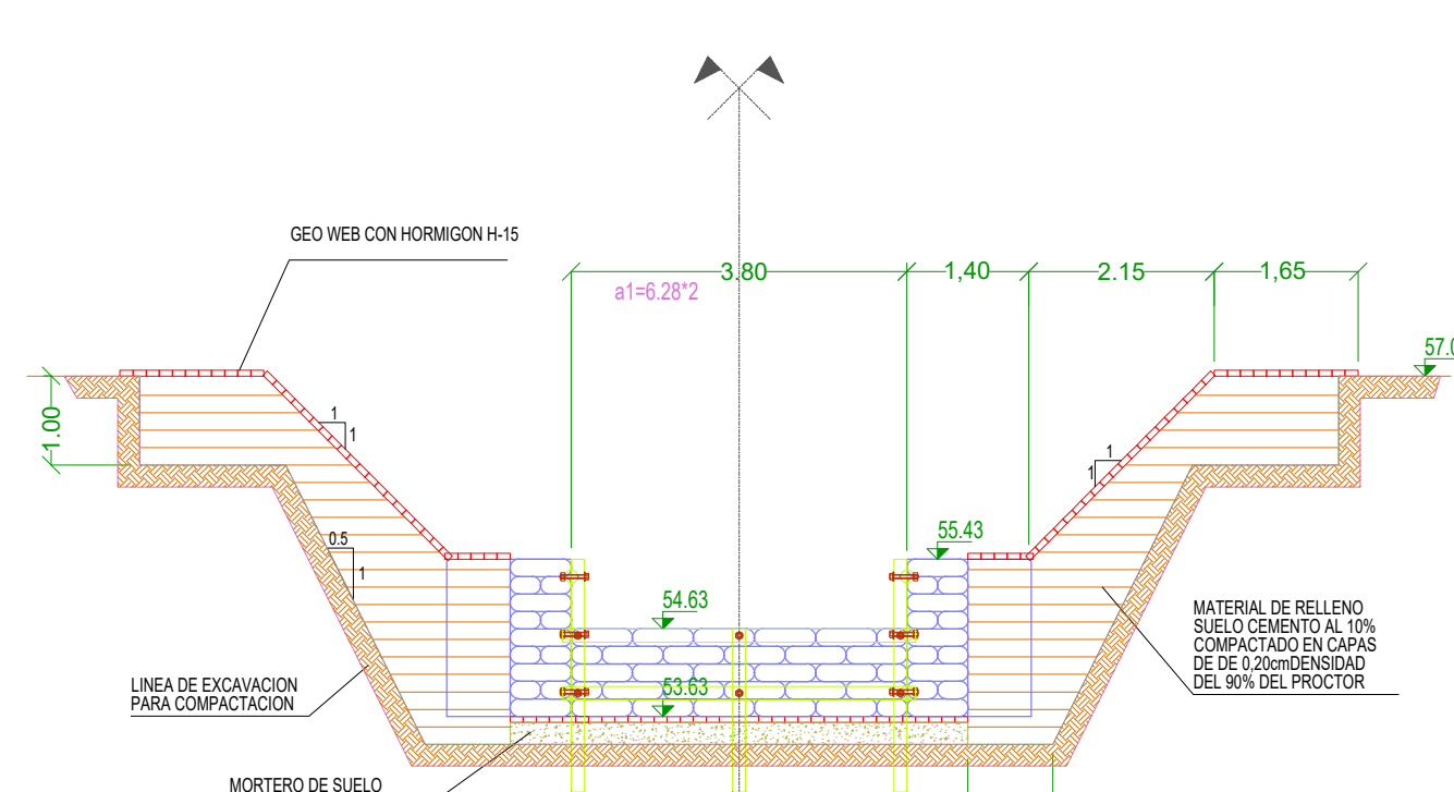
Seccion VI - VI
