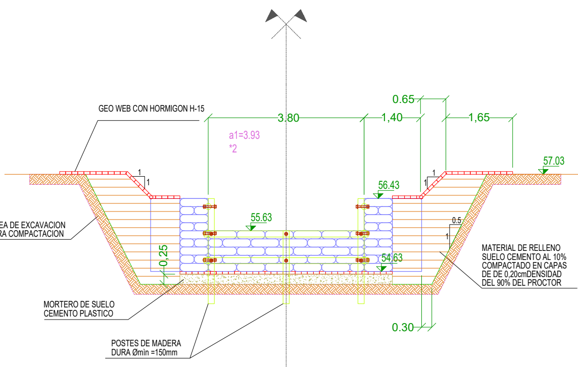
Seccion IV - IV
