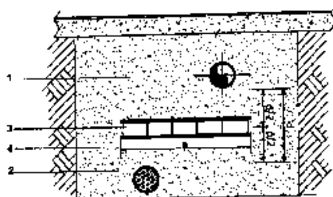
Figura 5a Protección con ladrillos más planchas de caucho sintético o placas de PRPV Paralelismo
