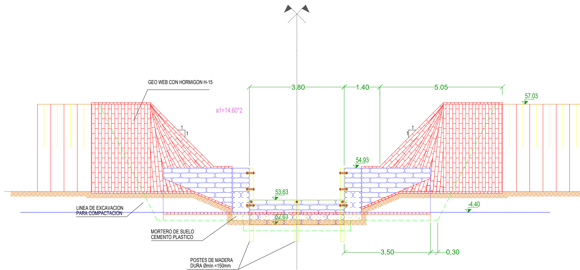
Seccion VIII - VIII
