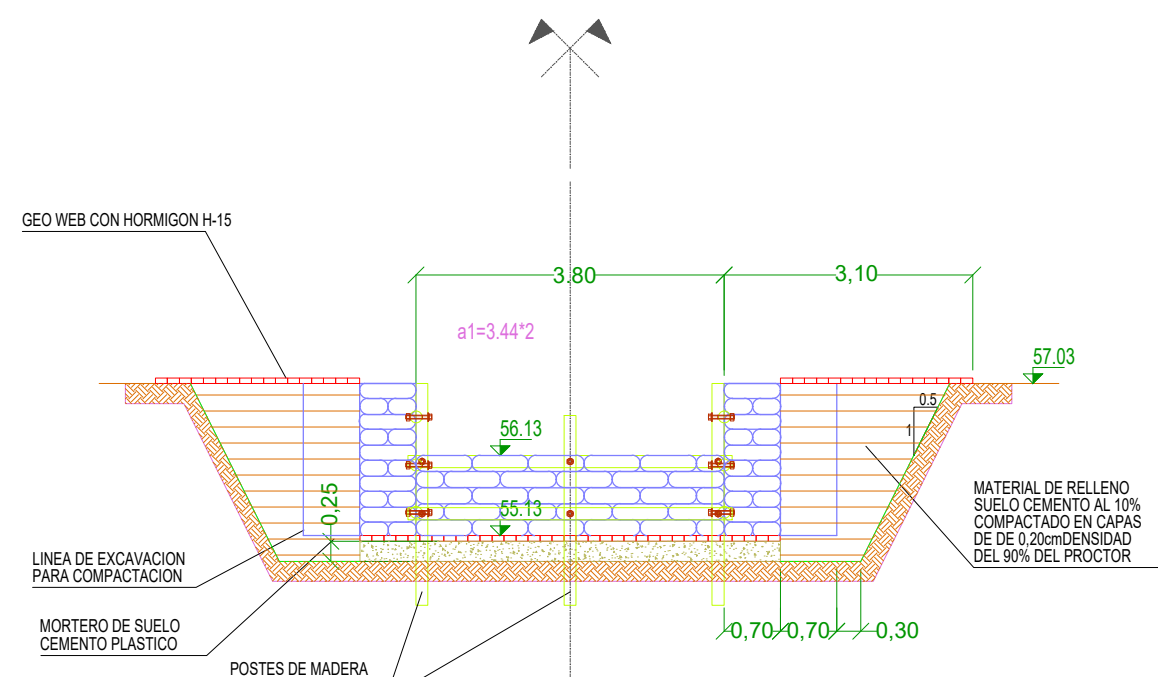
Seccion III - III
