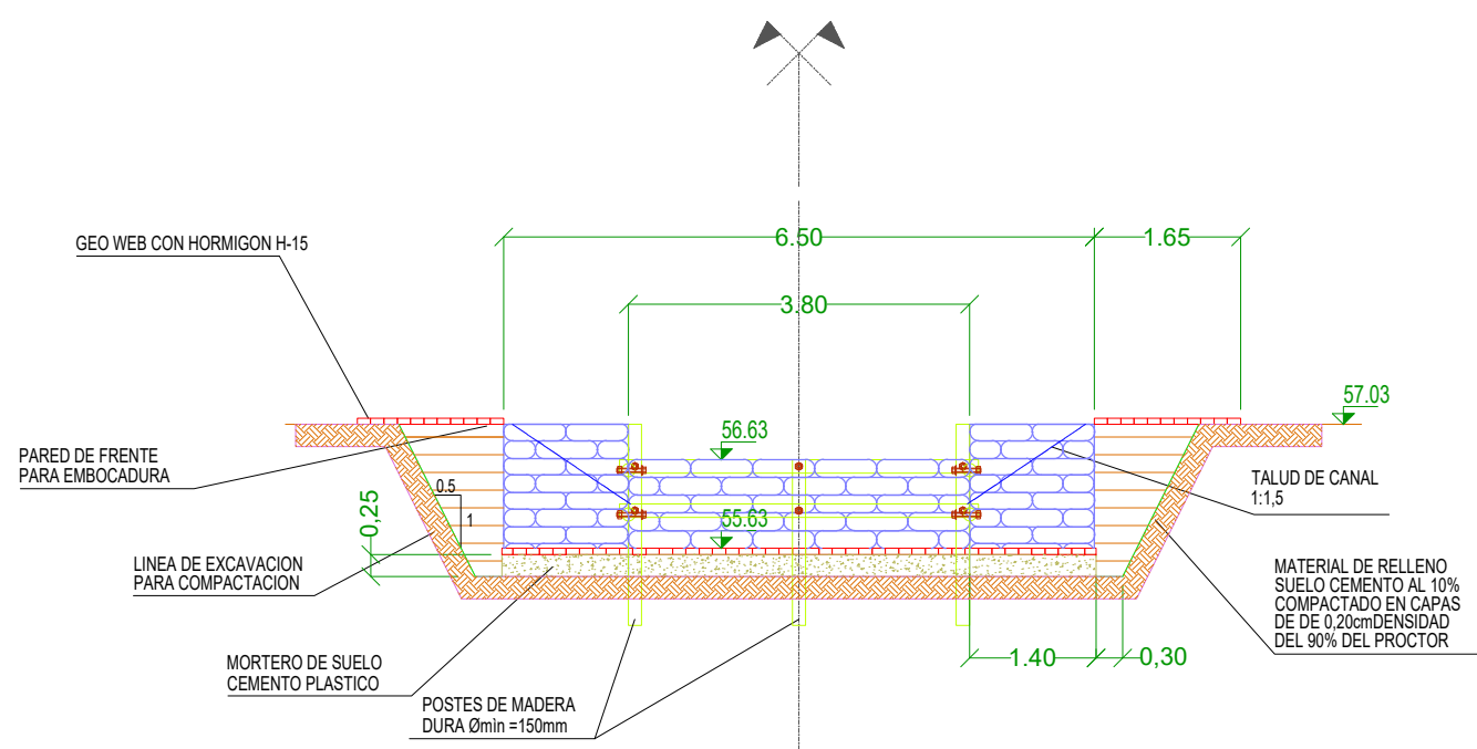
Seccion I - I
