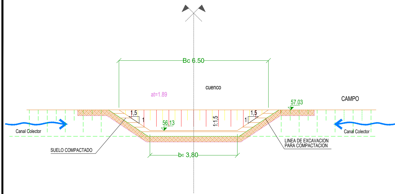
Seccion A - A
