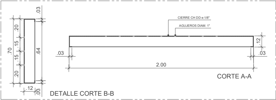
CORTE B-B
