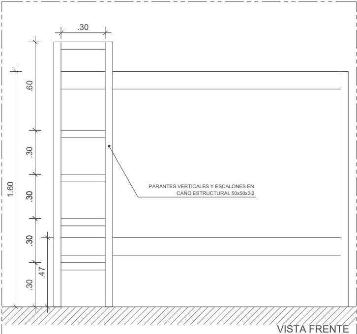
VISTA FRENTE
