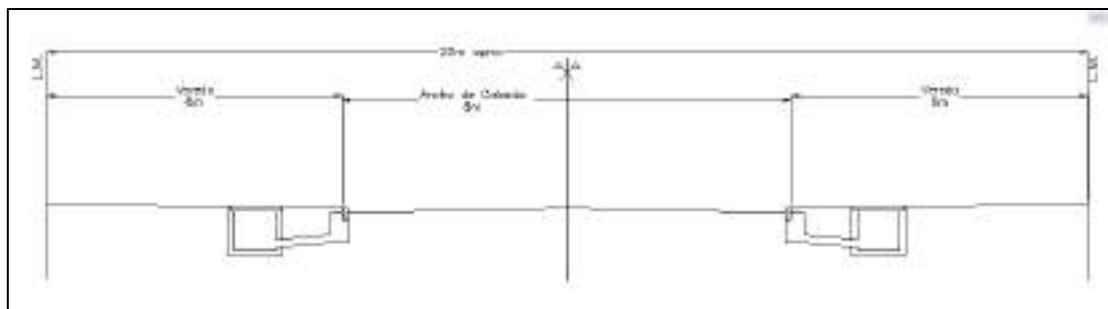
Figura 6 – Perfil de una sección vial tipo, con albañales cerrados y obras de captación
