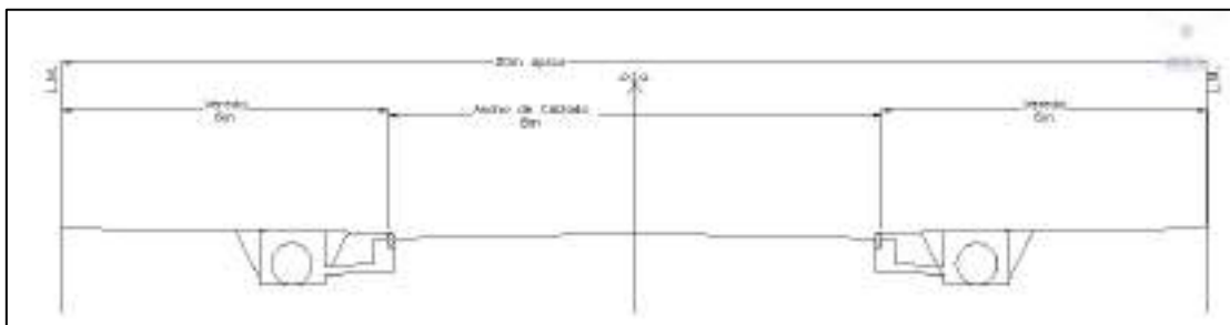
Figura 7 – Perfil tipo de una sección que propone entubar los desagües en vereda con cañerías PEAD por ejemplo.
