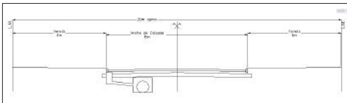
Figura 8 – Perfil tipo de una sección tipo con conducto pluvial enterrado y obra de captación (sumideros).-
