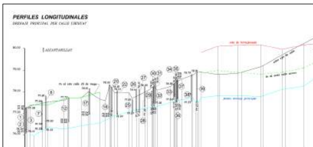
Figura 4 – Perfil de la traza en estudio (Fuente relevamiento SRH MlyT).-
