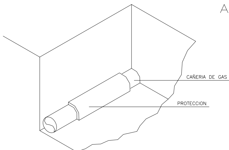
PROTECCION CON CAMISA FIG. 1
