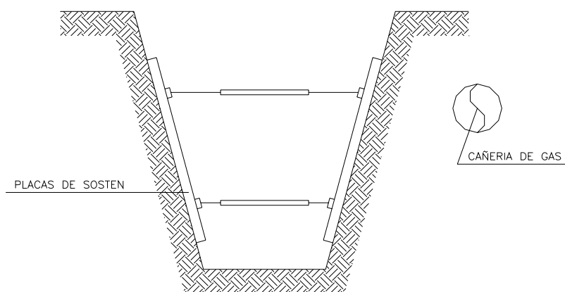
REFUERZO SOBRE PAREDES DE LA ZANJA FIG. 3
