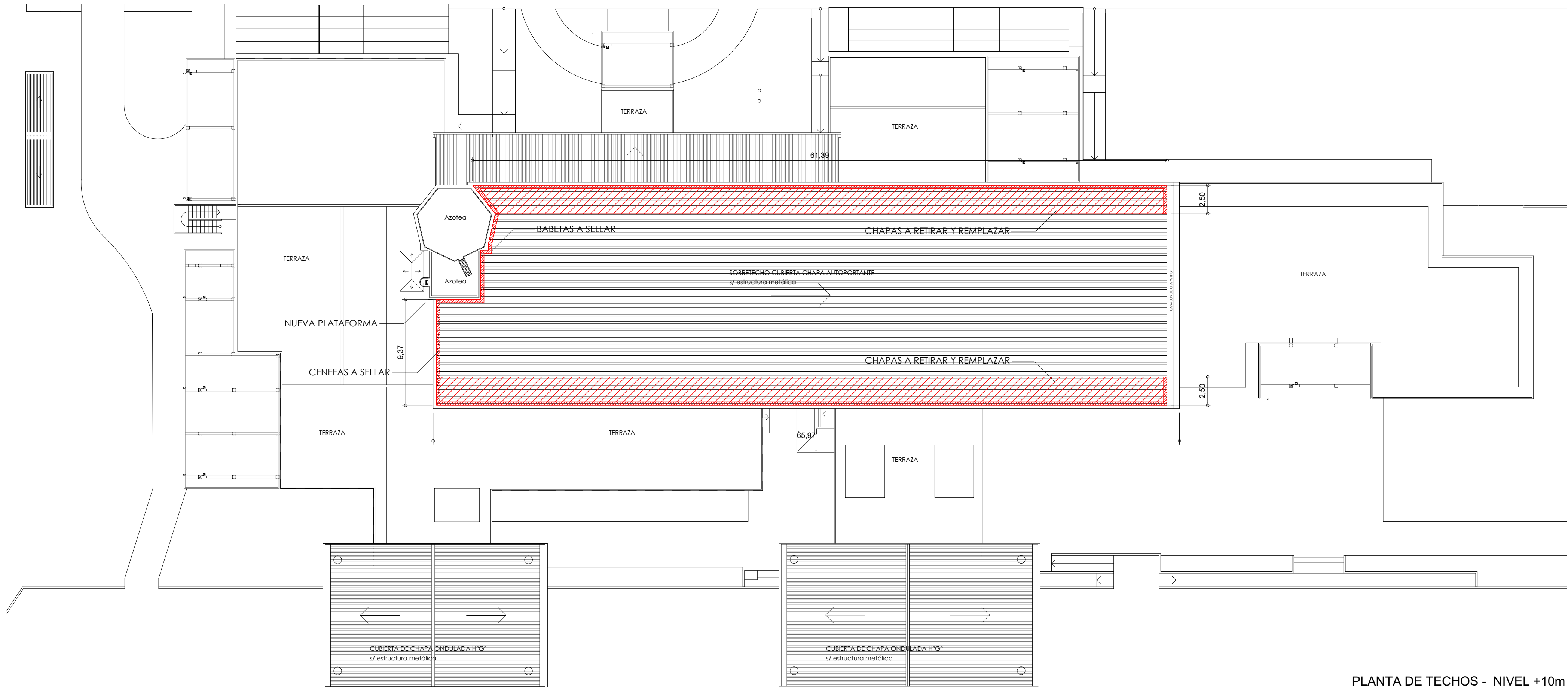
PLANTA DE TECHOS - NIVEL +10m
