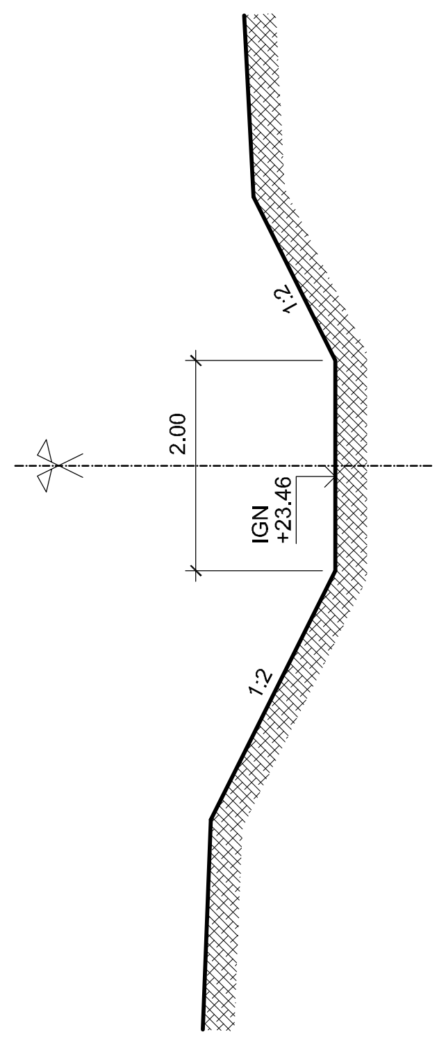
DETALLE 2 . 1:50
