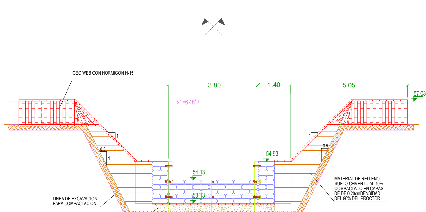
Seccion III - III
