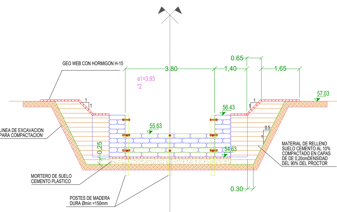
Seccion IV - IV
