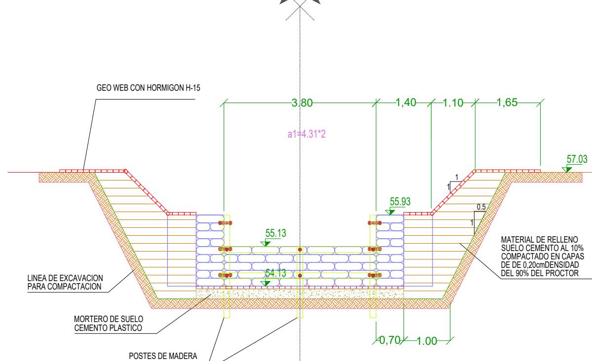
Seccion V - V
