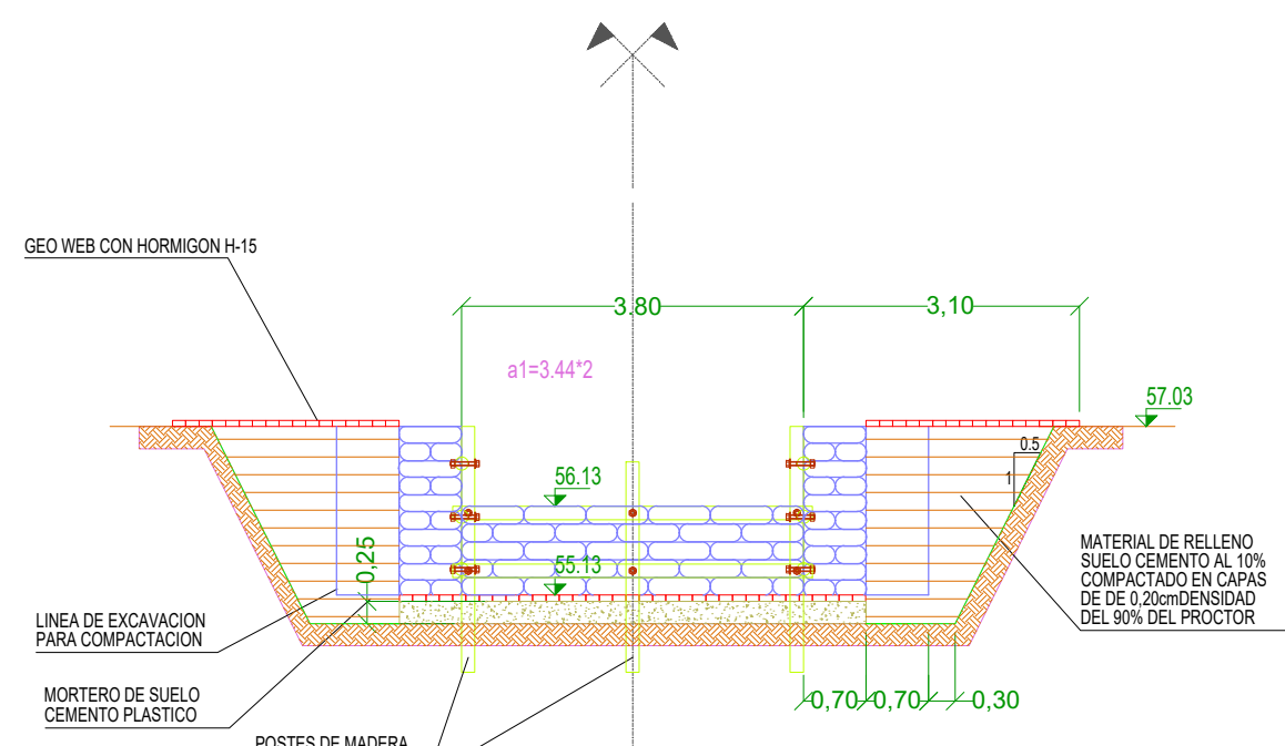
Seccion III - III
