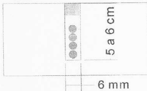
Figura: Corte transversal de la espira en el pavimento.
