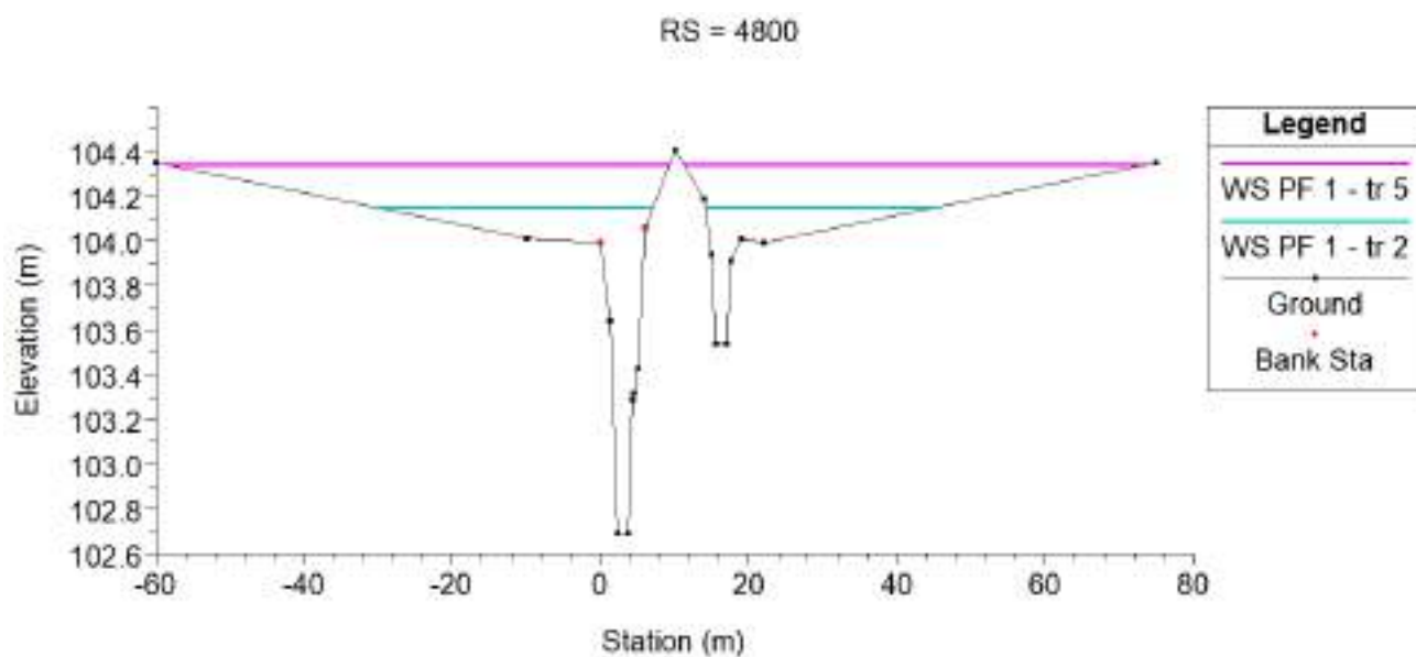
Imagen 21: (4+800) - Proyecto - Resultados: TR=2 cian, TR=5 en magenta.
