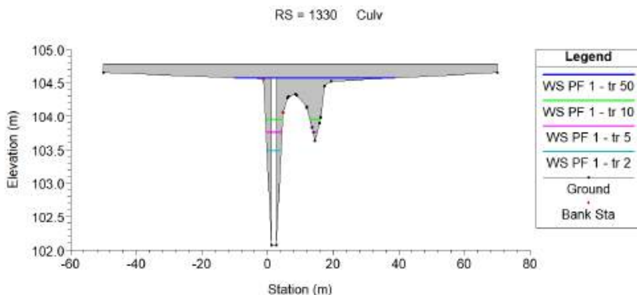
Imagen 30: Alcantarilla 6 - Resultados: TR=2 cian , TR=5 magenta TR=10 verde (diseño) y TR=50 Azul (verificación).
