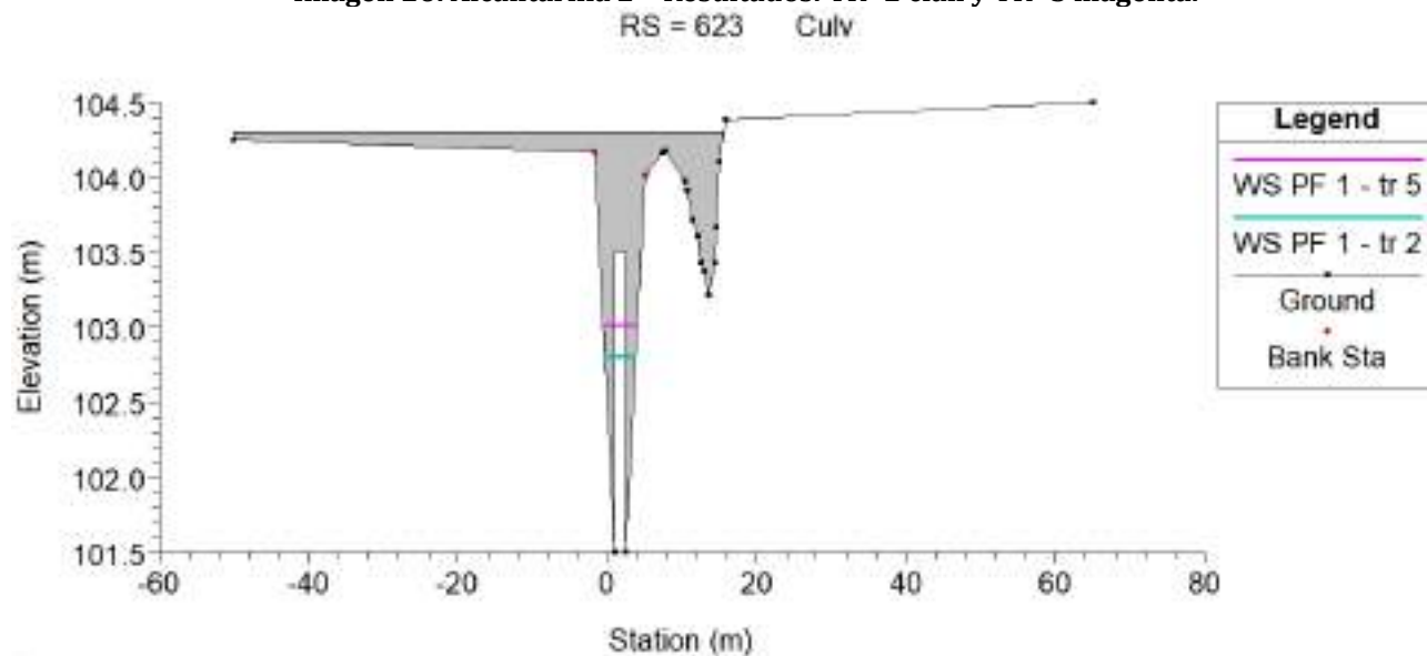
Imagen 27: Alcantarilla 3 - Resultados: TR=2 cian y TR=5 magenta.
