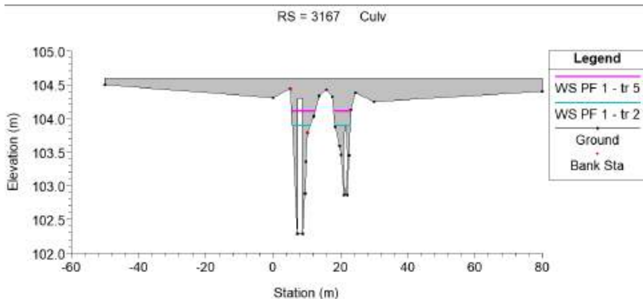
Imagen 35: Alcantarilla 5 - Resultados: TR=2 cian y TR=5 magenta.
