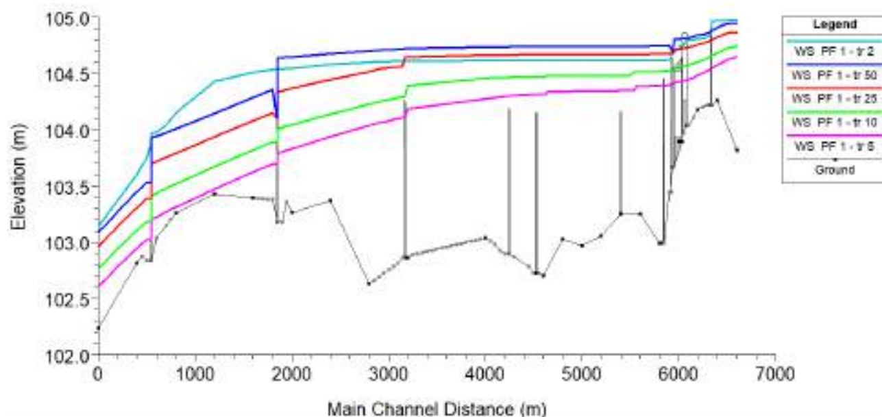
Imagen 13: Perfil longitudinal Rural – Situación Actual – Resultados: TR=2 en cian, TR=5 en magenta, TR=10 en verde, TR=25 en rojo y TR=50 azul.
