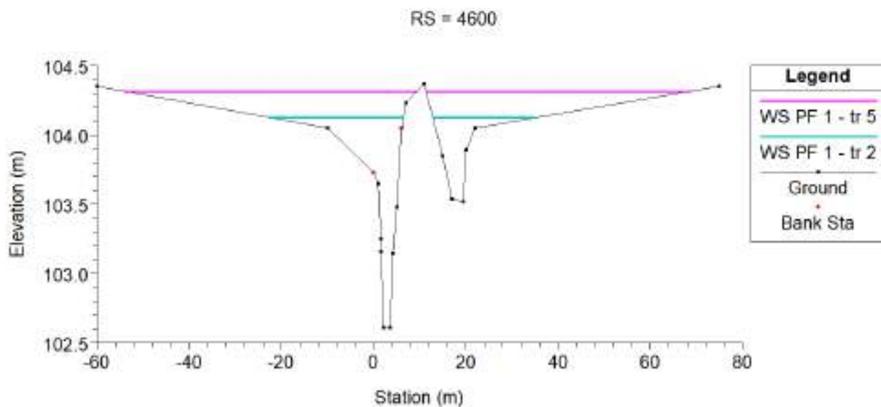
Imagen 20: (4+600) - Proyecto - Resultados: TR=2 cian, TR=5 en magenta.
