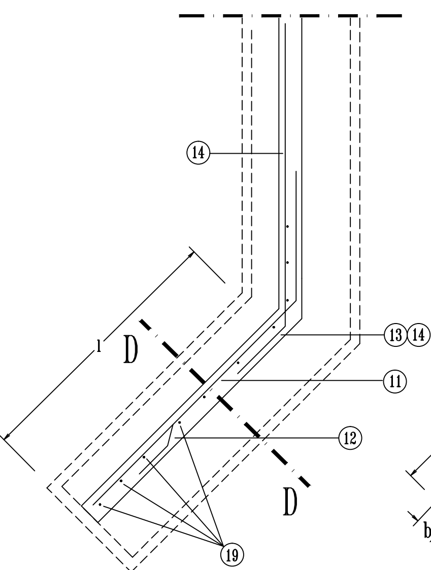
DETALLE MURO DE ALA CON ZAPATA DE FUNDACION
