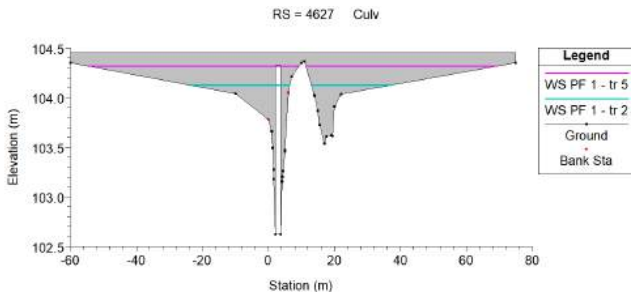
Imagen 36: Alcantarilla 13 - Resultados: TR=2 cian y TR=5 magenta.
