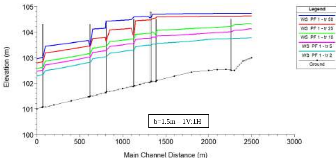
Imagen 16: Perfil longitudinal Urbano – Situación Proyecto- Resultados: TR=2 en cian, TR=5 en magenta, TR=10 en verde, TR=25 en rojo y TR=50 azul.
