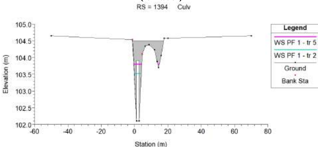
Imagen 31: Alcantarilla 8 - Resultados: TR=2 cian y TR=5 magenta.
