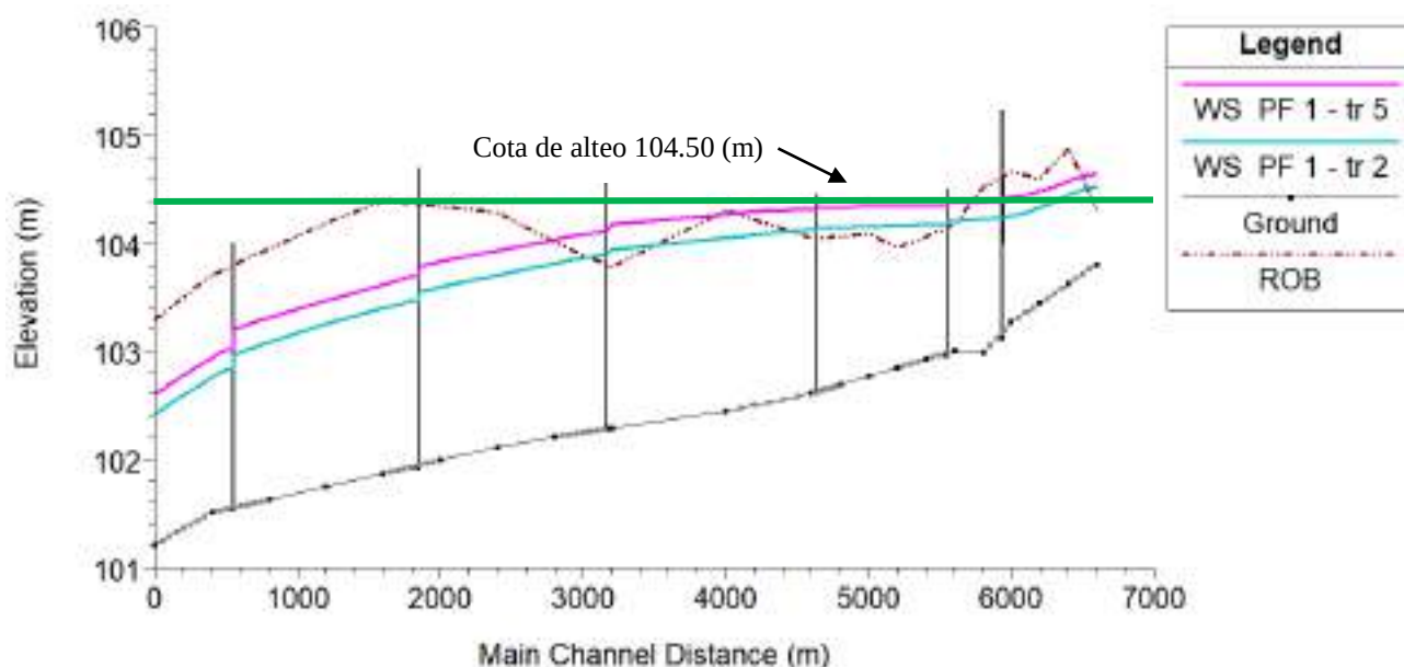
Imagen 17: Perfil longitudinal Rural – Situación Proyecto- Resultados: TR=2 en cian y TR=5 en magenta – tramo de progresiva 2800 a 5600 en el que se debe altear a cota 104.50 (m)
