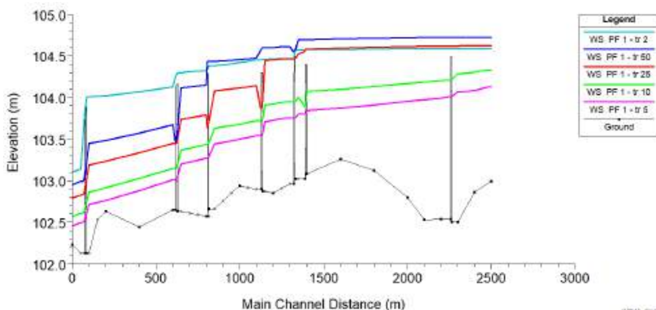
Imagen 14: Perfil longitudinal Urbano - Situación Actual - Resultados: TR=2 en cian, TR=5 en magenta, TR=10 en verde, TR=25 en rojo y TR=50 azul.
