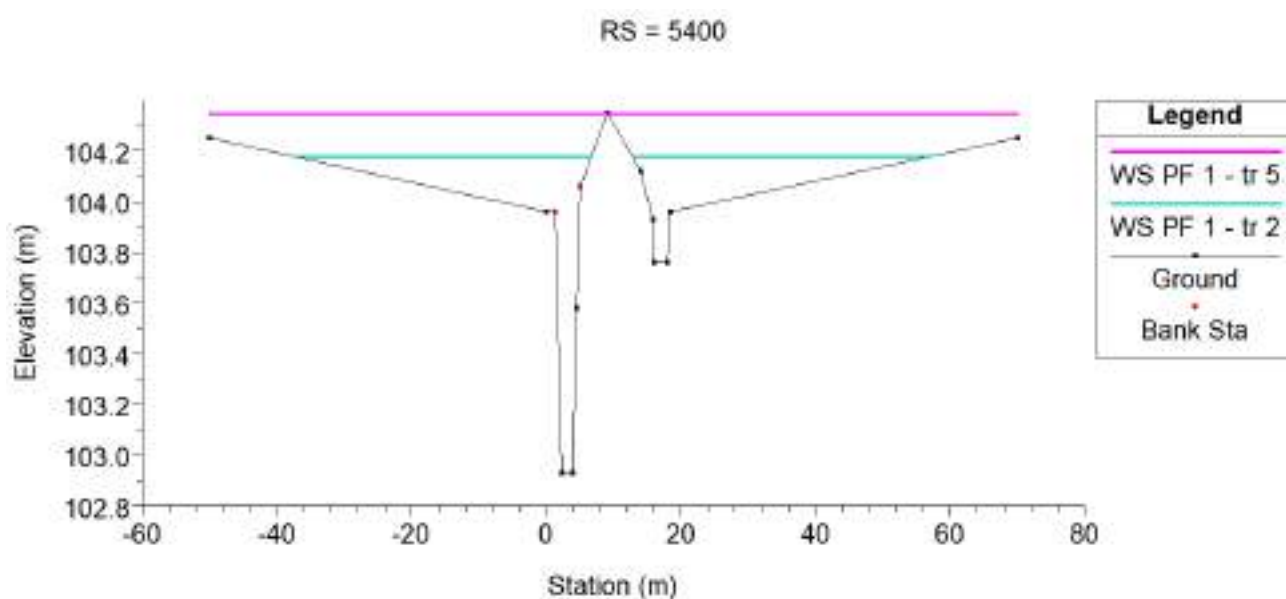
Imagen 24: (5+400) – Proyecto – Resultados: TR=2 cian, TR=5 en magenta.
