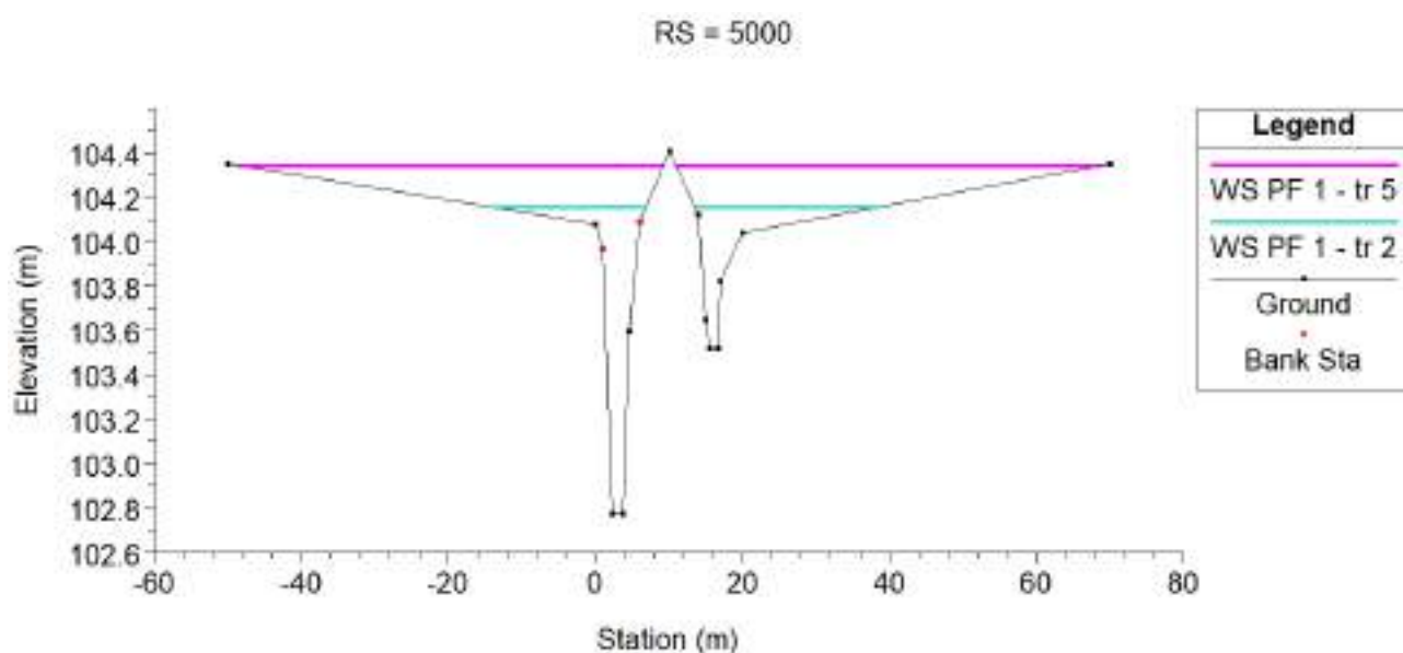
Imagen 22: (5+000) - Proyecto - Resultados: TR=2 cian, TR=5 en magenta.
