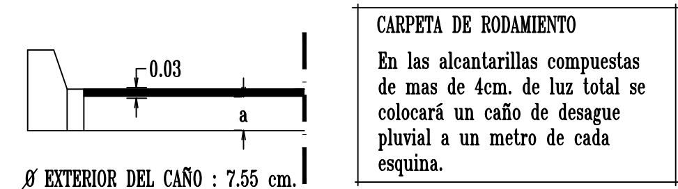
CAÑO DESAGUE PLUVIAL DE FIBROCEMENTO
