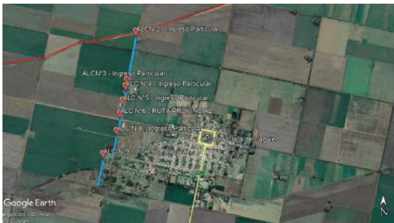
Imagen 4: Ubicación de alcantarillas existentes en canal urbano
