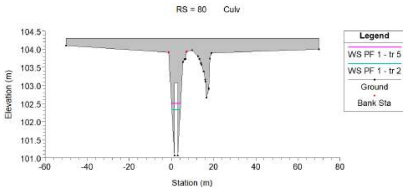
Imagen 26: Alcantarilla 2 - Resultados: TR=2 cian y TR=5 magenta.
