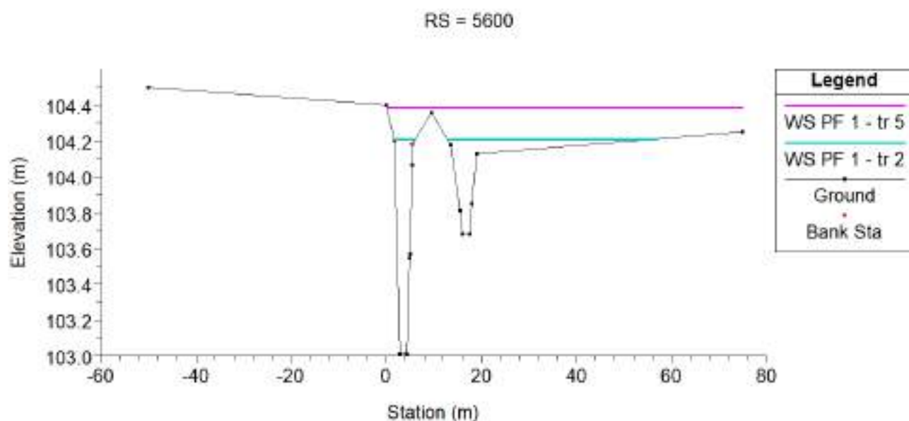
Imagen 25: (5+600) – Proyecto – Resultados: TR=2 cian, TR=5 en magenta.
