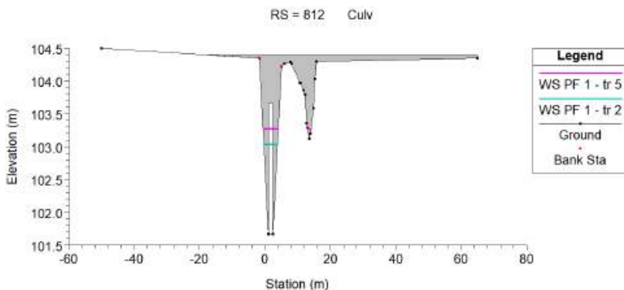
Imagen 28: Alcantarilla 4 - Resultados: TR=2 cian y TR=5 magenta.
