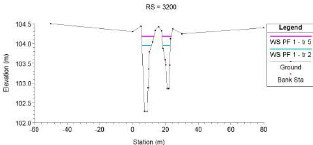
Imagen 18: (3+200) - Proyecto - Resultados: TR=2 cian, TR=5 en magenta.
