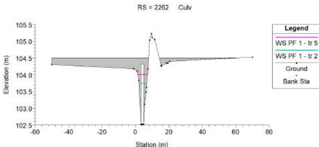
Imagen 32: Alcantarilla 9 - Resultados: TR=2 cian y TR=5 magenta.
