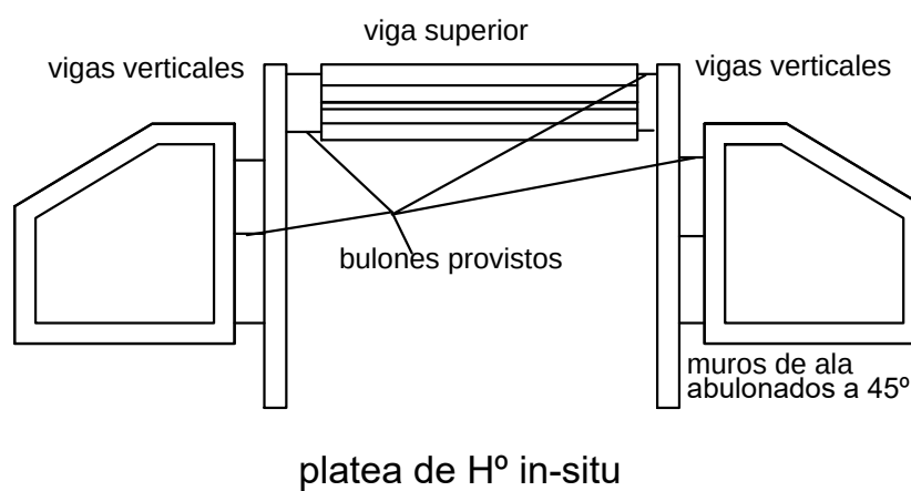
Vista frontal del cabezal
