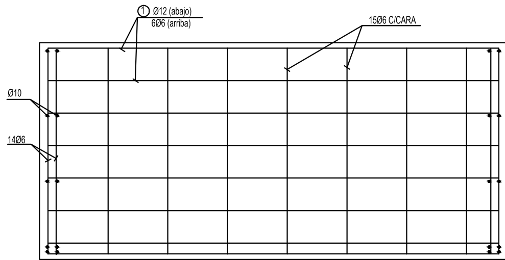
VISTA SUPERIOR ARMADURAS
