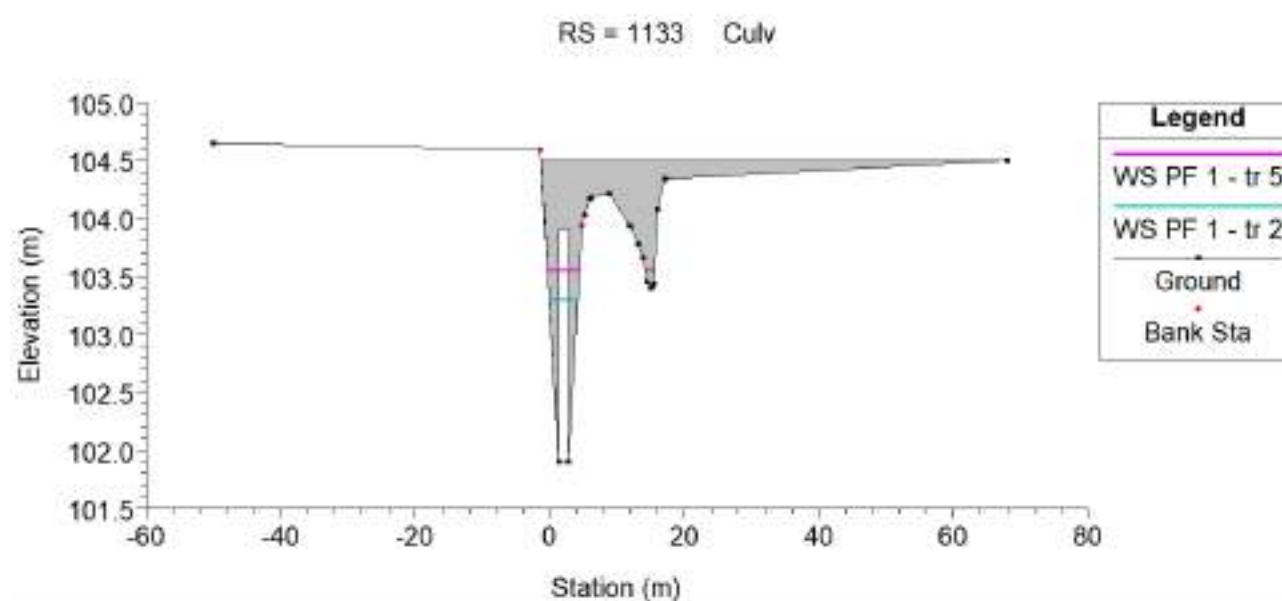
Imagen 29: Alcantarilla 5 - Resultados: TR=2 cian y TR=5 magenta
