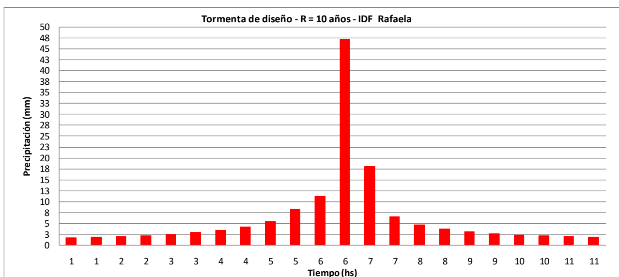
Imagen 9: Hietograma de diseño para 10 años de recurrencia obtenido de la IDF de Rafaela.
