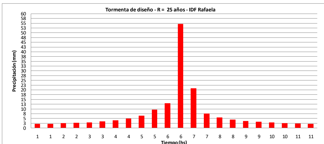
Imagen 10: Hietograma de diseño para 25 años de recurrencia obtenido de la IDF de Rafaela.
