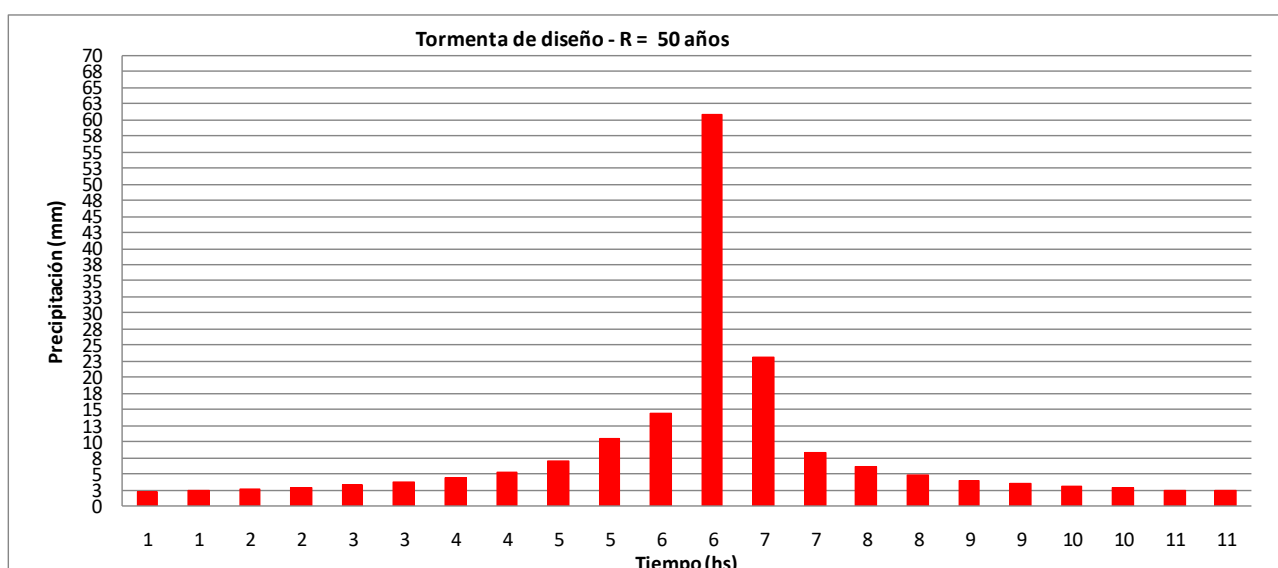
Imagen 11: Hietograma de diseño para 50 años de recurrencia obtenido de la IDF de Rafaela.
