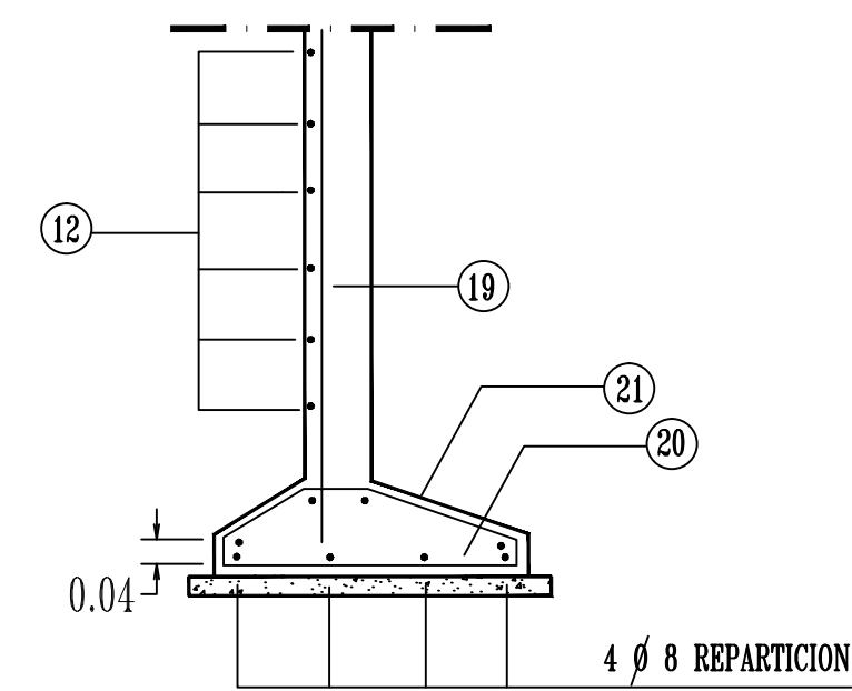
SECCION D-D
