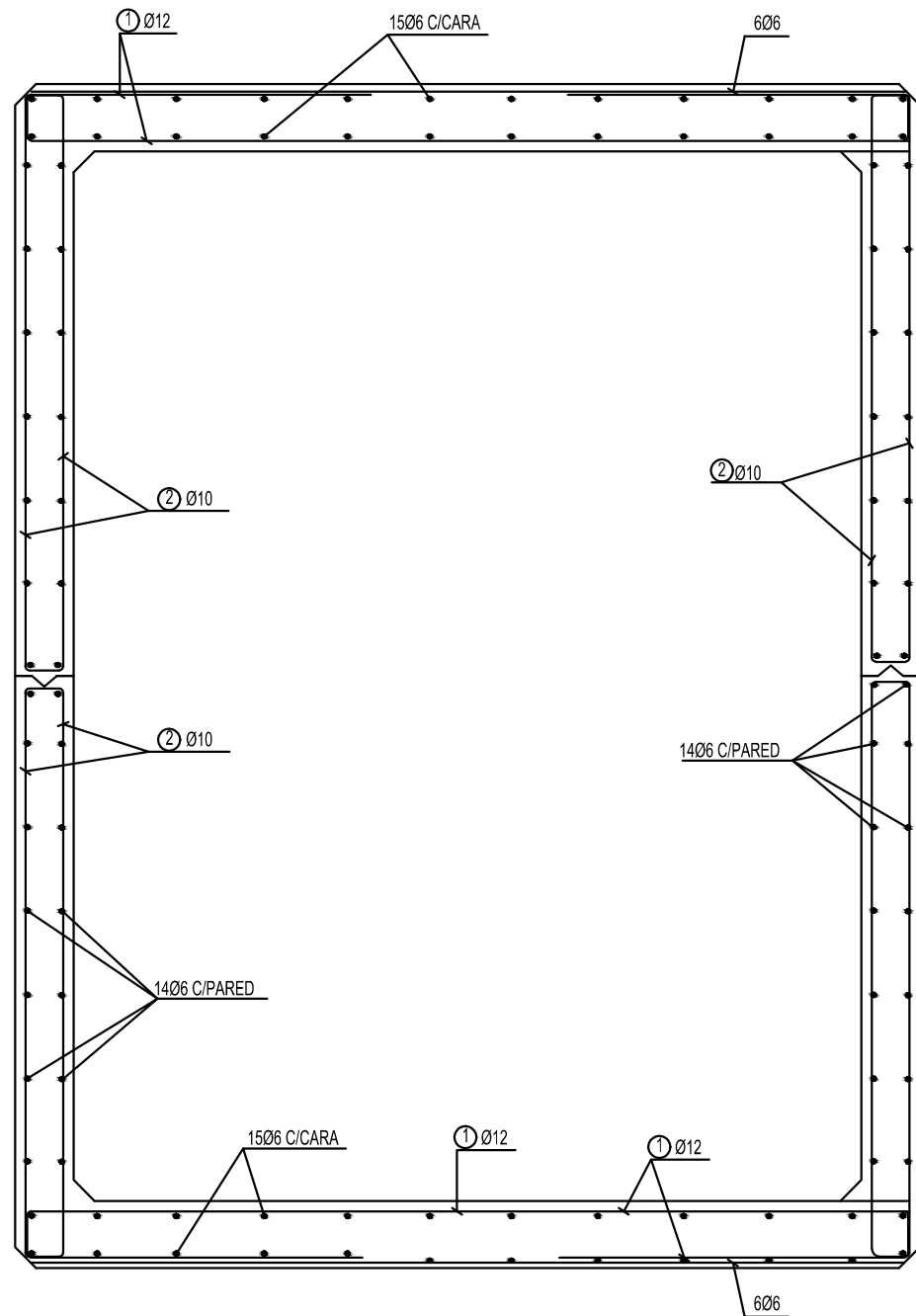
FRENTE DOBLE U ARMADURAS
