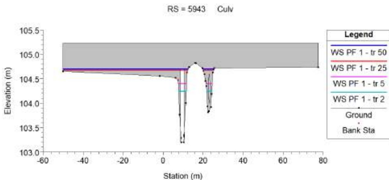
Imagen 38: Alcantarilla 16 - Resultados: TR=2 cian , TR=5 magenta TR=25 rojo (diseño) y TR=50 Azul (verificación)
