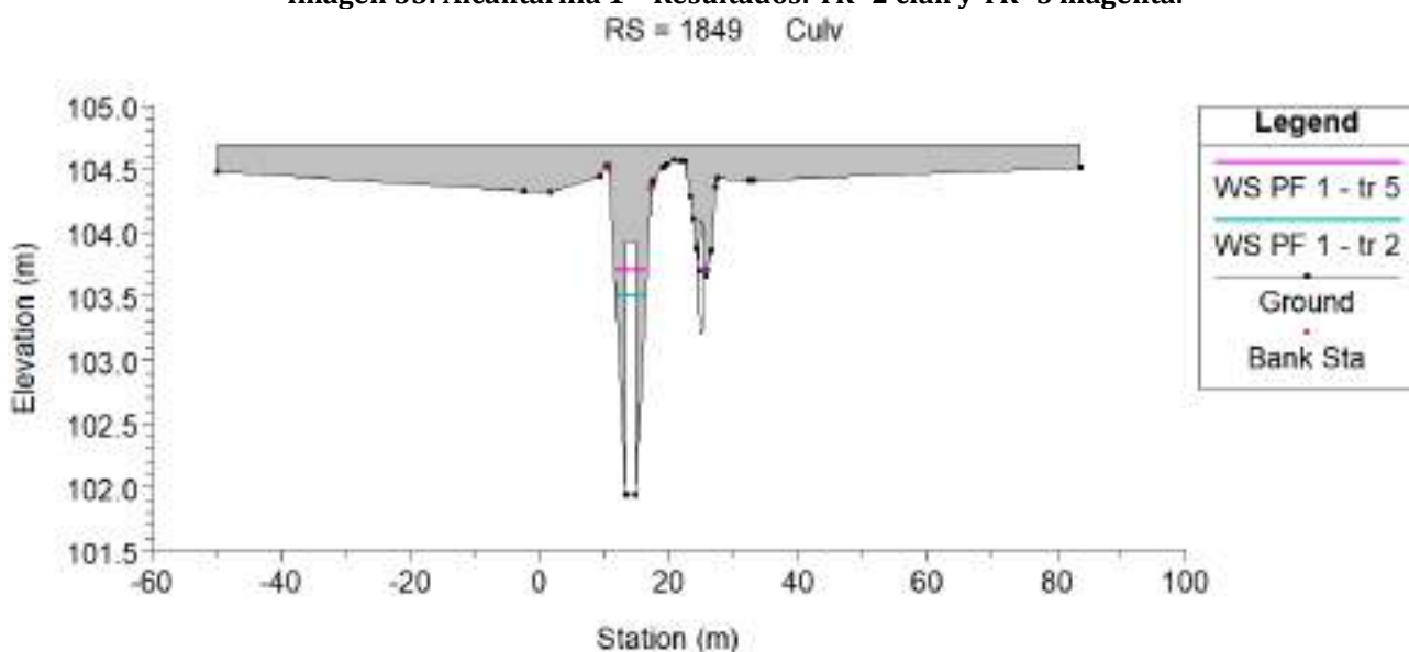
Imagen 34: Alcantarilla 4 - Resultados: TR=2 cian y TR=5 magenta.
