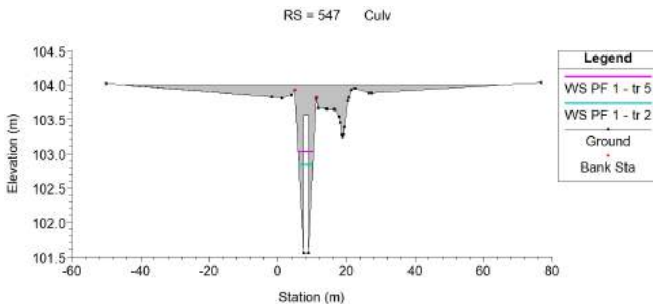
Imagen 33: Alcantarilla 1 - Resultados: TR=2 cian y TR=5 magenta.
