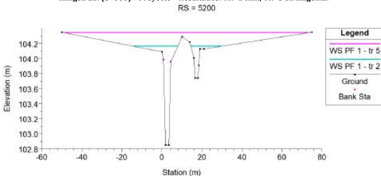
Imagen 23: (5+200) - Proyecto - Resultados: TR=2 cian, TR=5 en magenta.
