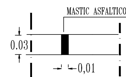
DETALLE DE JUNTA
