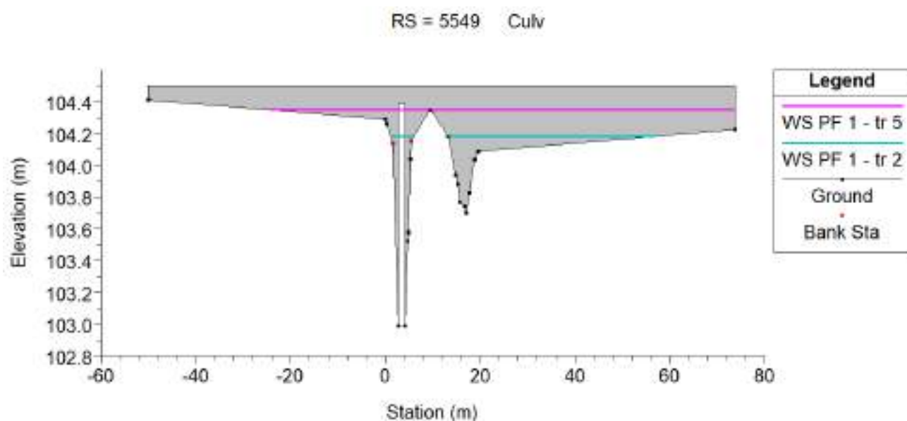
Imagen 37: Alcantarilla 15 - Resultados: TR=2 cian y TR=5 magenta.
