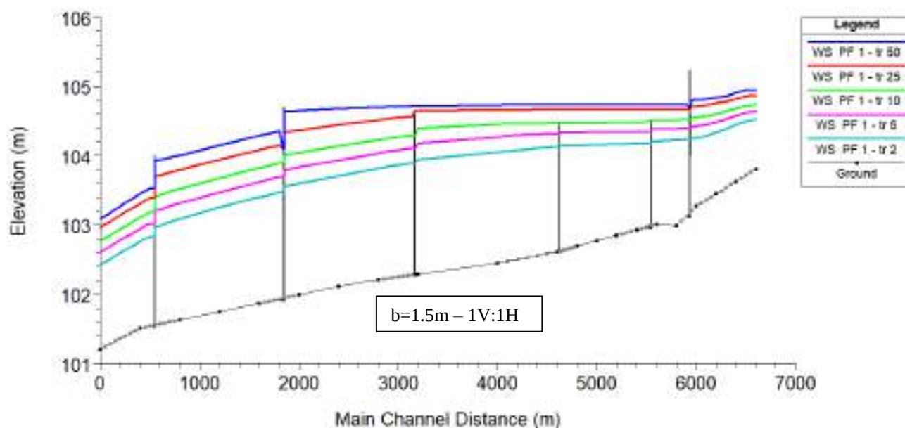
Imagen 15: Perfil longitudinal Rural - Situación Proyecto - Resultados: TR=2 en cian, TR=5 en magenta, TR=10 en verde, TR=25 en rojo y TR=50 azul.
