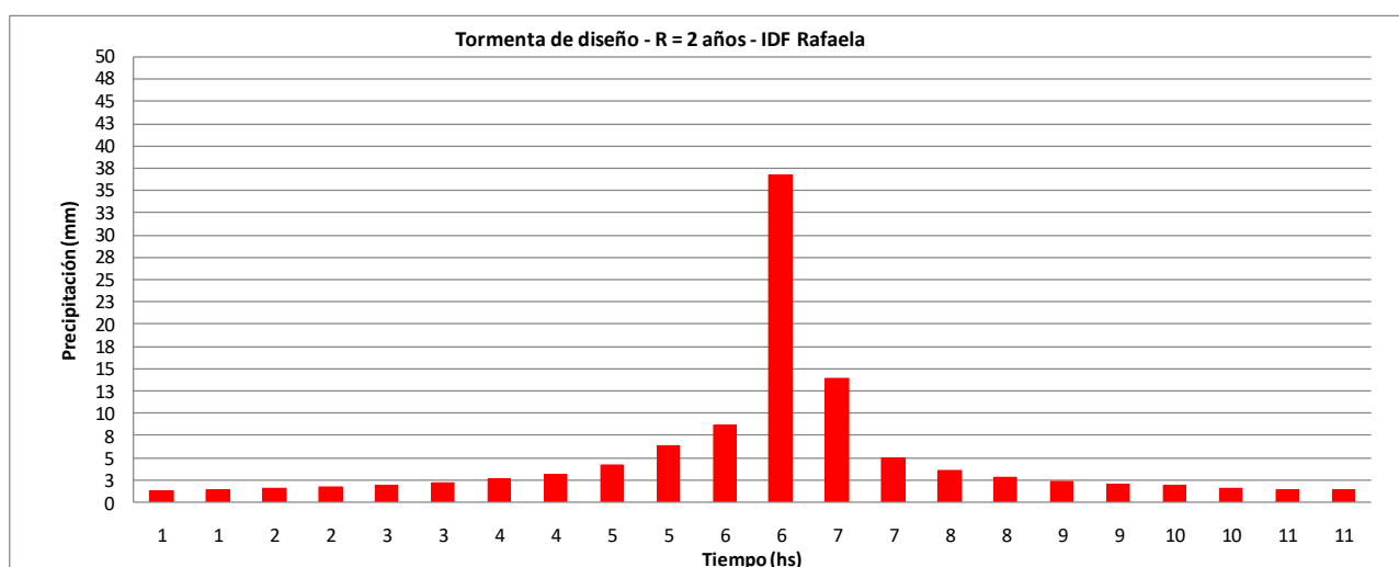
Imagen 7: Hietograma de diseño para 2 años de recurrencia obtenido de la IDF de Rafaela.
