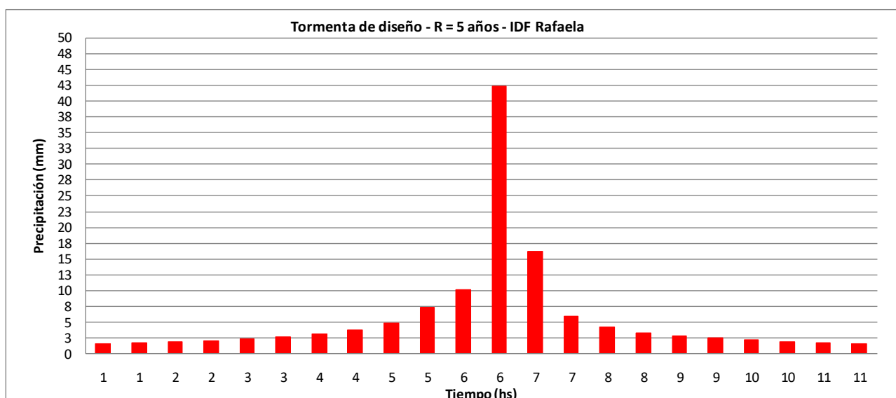
Imagen 8: Hietograma de diseño para 5 años de recurrencia obtenido de la IDF de Rafaela.
