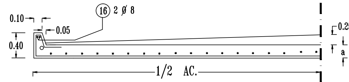
DETALLE PLATEA
