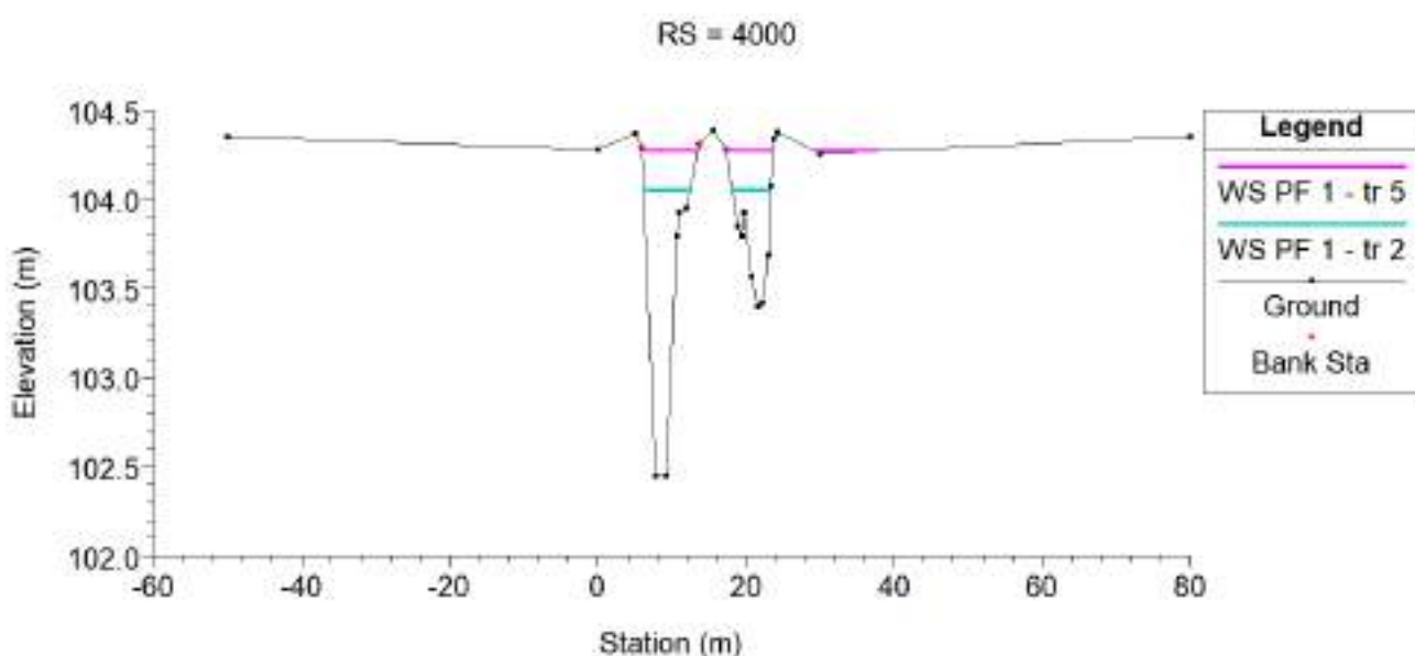
Imagen 19: (4+000) - Proyecto - Resultados: TR=2 cian, TR=5 en magenta.
