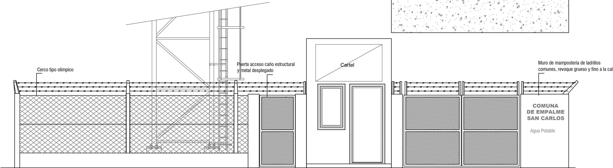
FACHADA SUR Esc. 1:50
