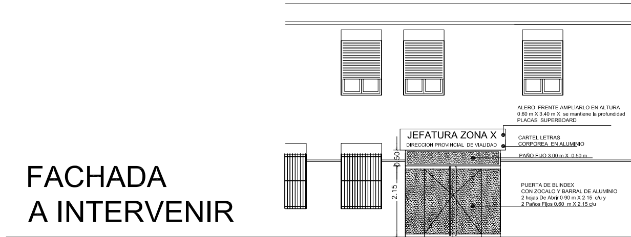
DETALLE: FACHADA INGRESO PRINCIPAL A INTERVENIR
