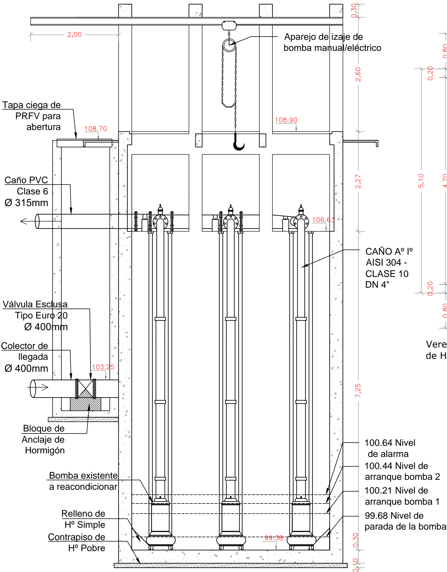
CORTE A-A
