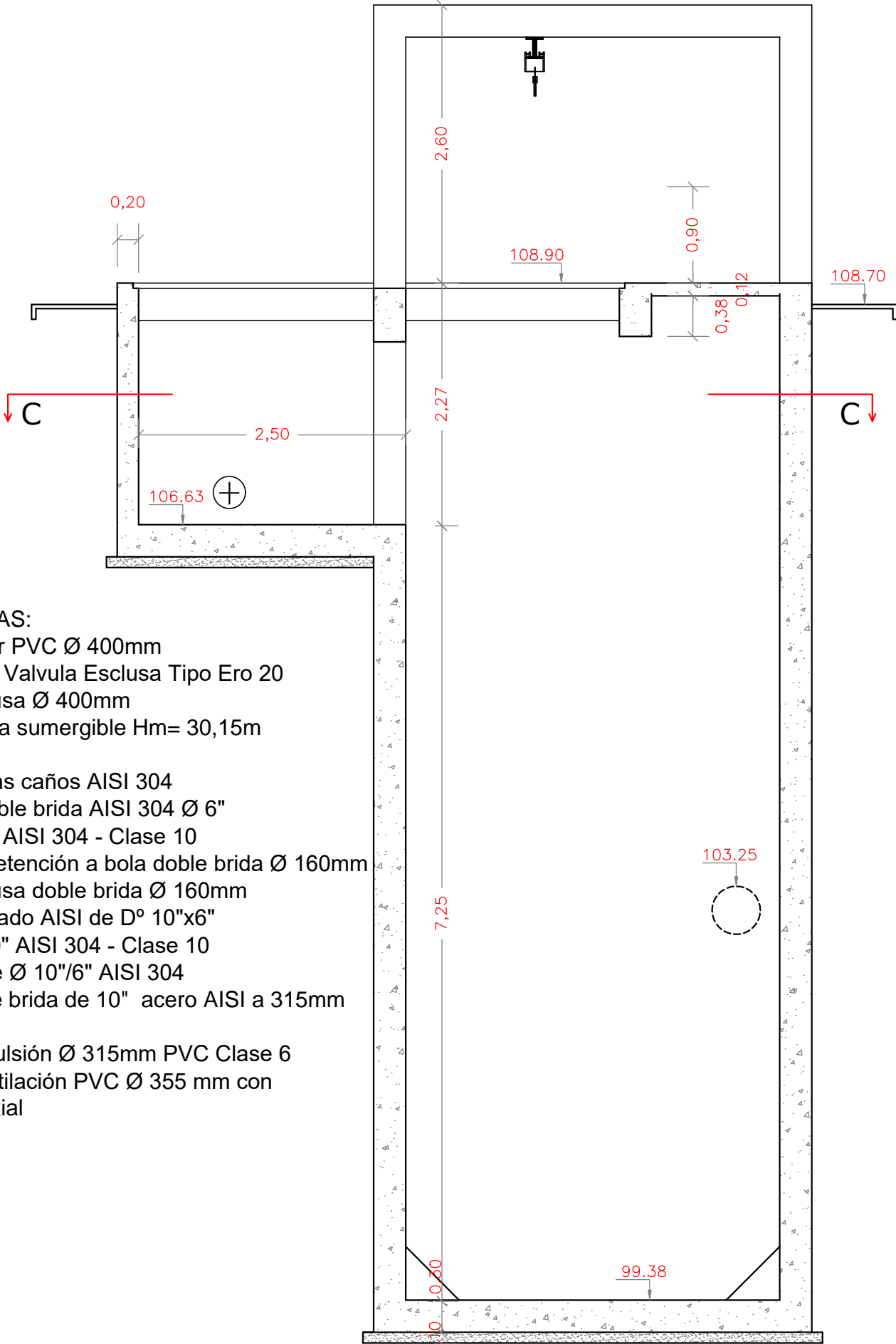
CORTE B-B
