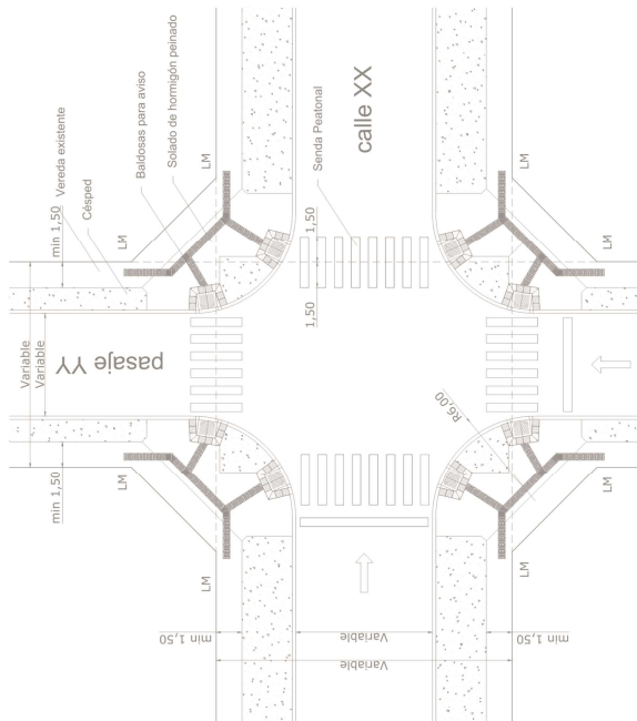
DETALLE DE ESQUINA TIPO - ENCUENTRO DE CALLE CON PASAJE
