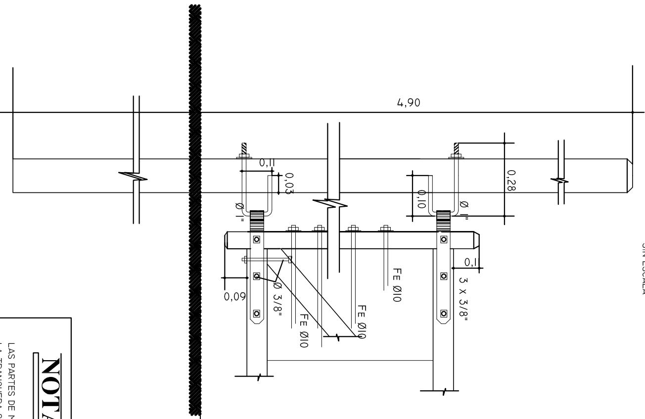
DETALLE B
