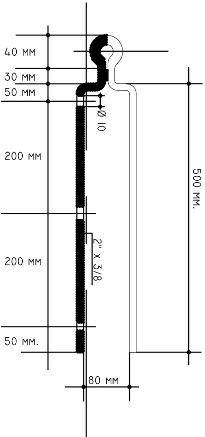
DETALLE DE BISAGRA
