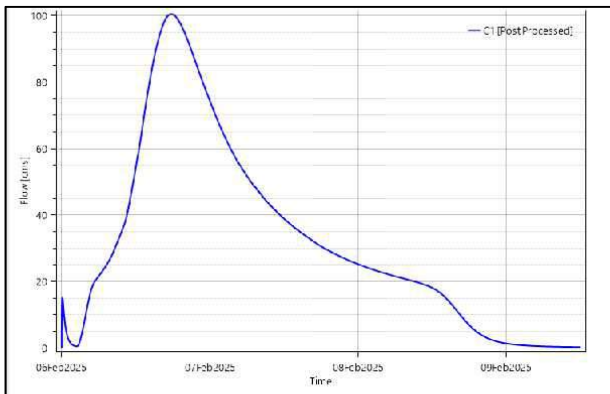
Imagen 19: Hidrograma de descarga total del sistema
