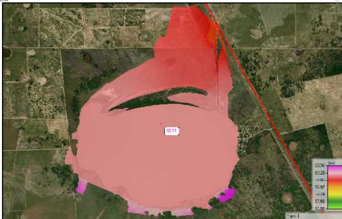
Imagen 22: Mancha máxima generada para el hidrograma teórico – Q no permanente
