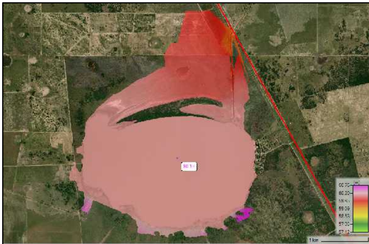
Imagen 16: Mancha máxima generada para el hidrograma teórico – Q permanente
