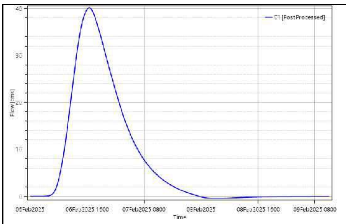
Imagen 21: Hidrograma de descarga "lengua" aliviadora
