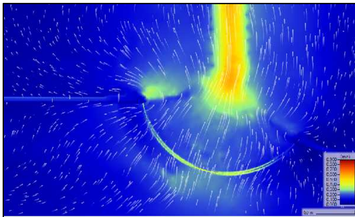
Imagen 23: Distribución del flujo máximo – Q no permanente
