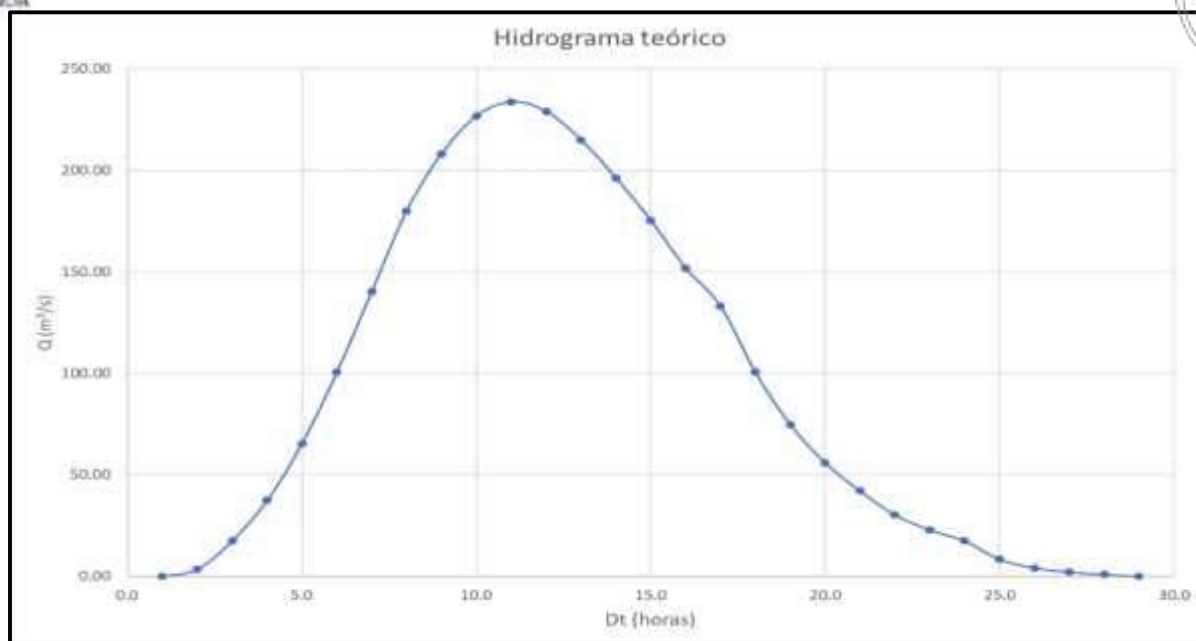
Imagen 15: Hidrograma para condición de flujo no permanente
