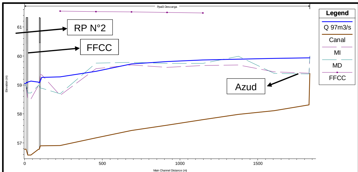
Imagen 25: Perfil Longitudinal canal con resultados Q permanente
