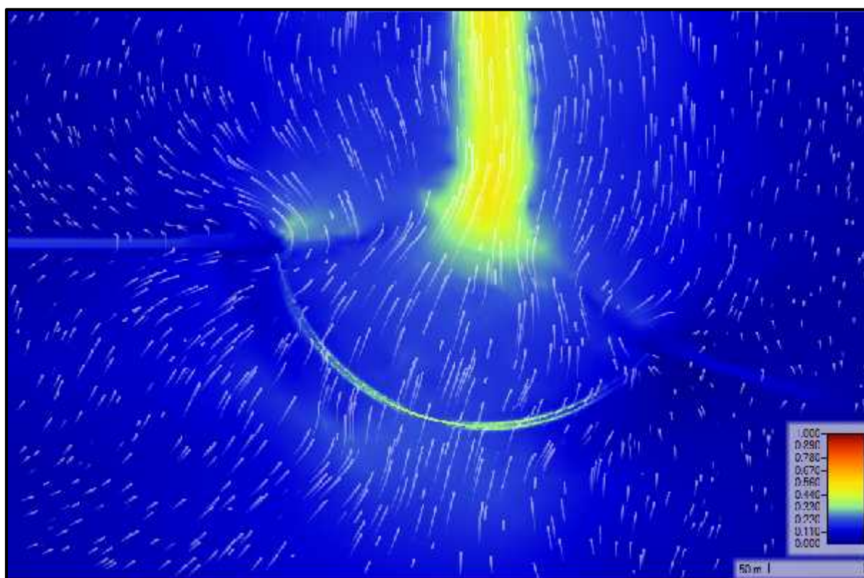
Imagen 18: Distribución del flujo en sector de descarga – Q permanente
