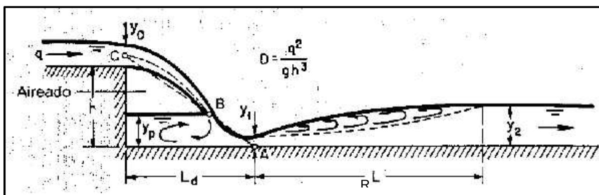
Imagen 28: Geometría de flujo en un vertedero de caída recta 5
