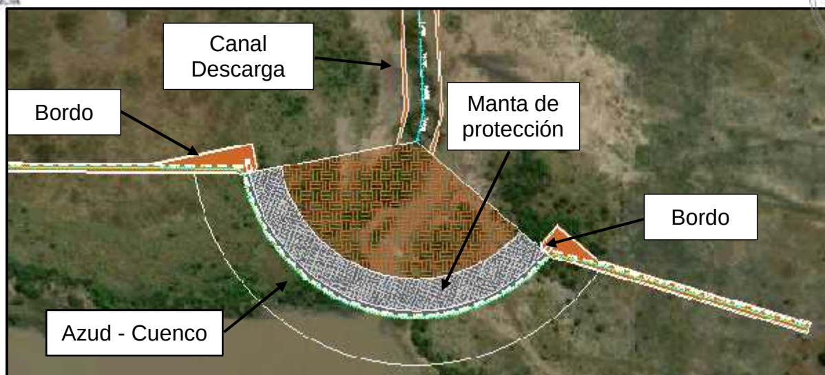
Imagen 8: Planta de azud, cuenco y bordo
