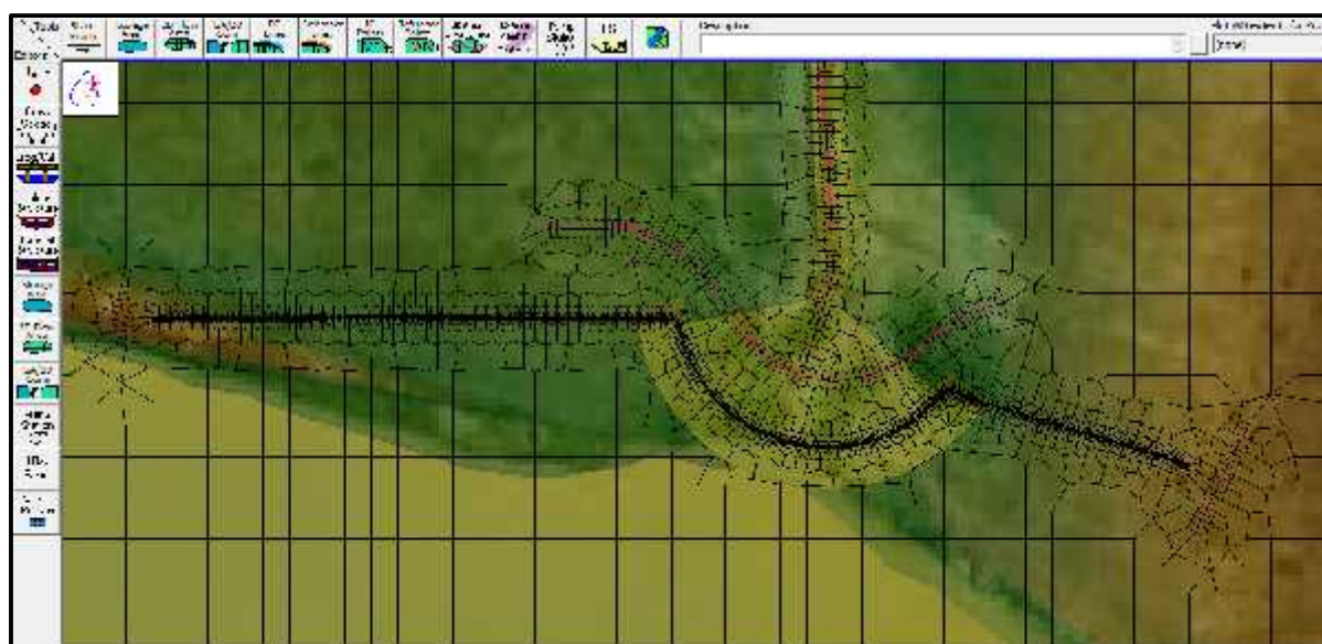
Imagen 13: Malla del área 2D en sector de obras
