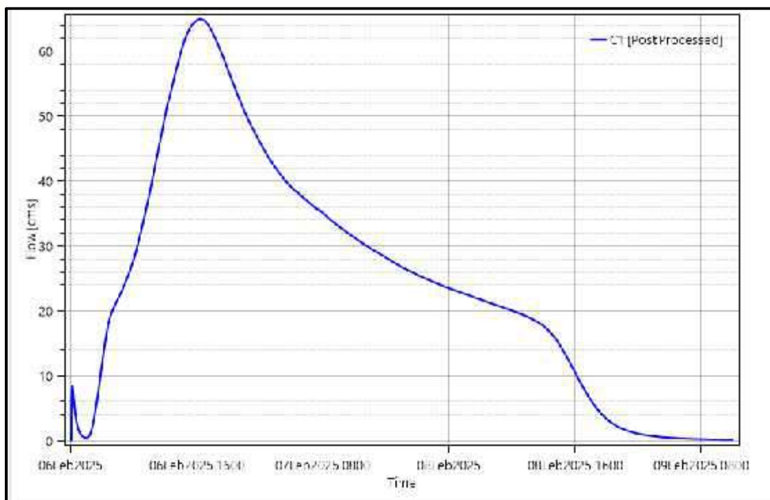
Imagen 20: Hidrograma de descarga azud-bordo-Canal Ppal N°3
