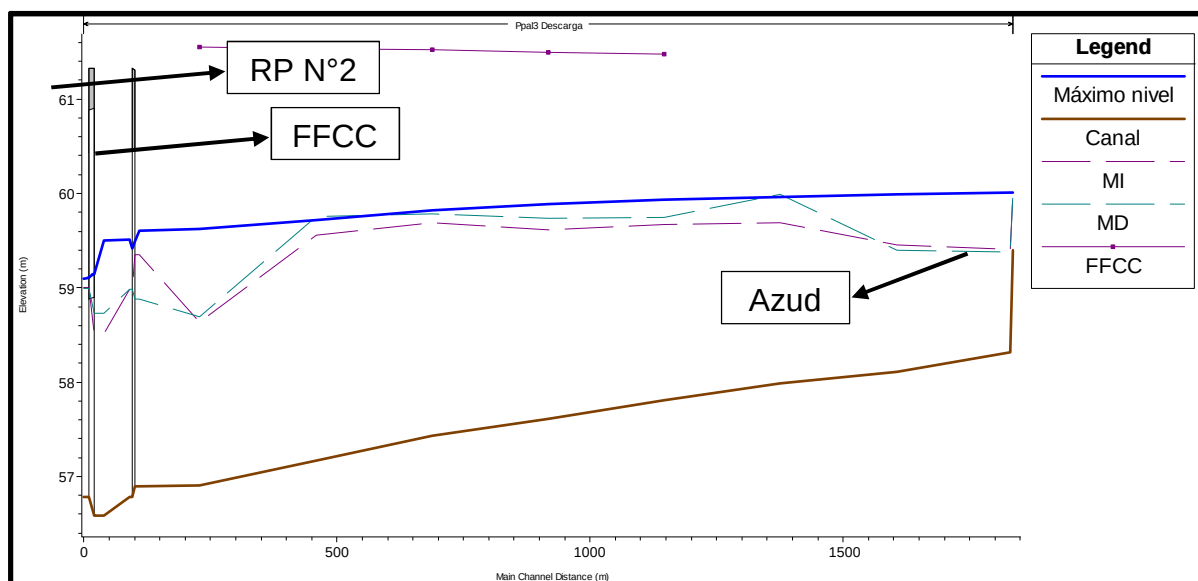
Imagen 26: Perfil Longitudinal con nivel máximo alcanzado para Q no permanente
