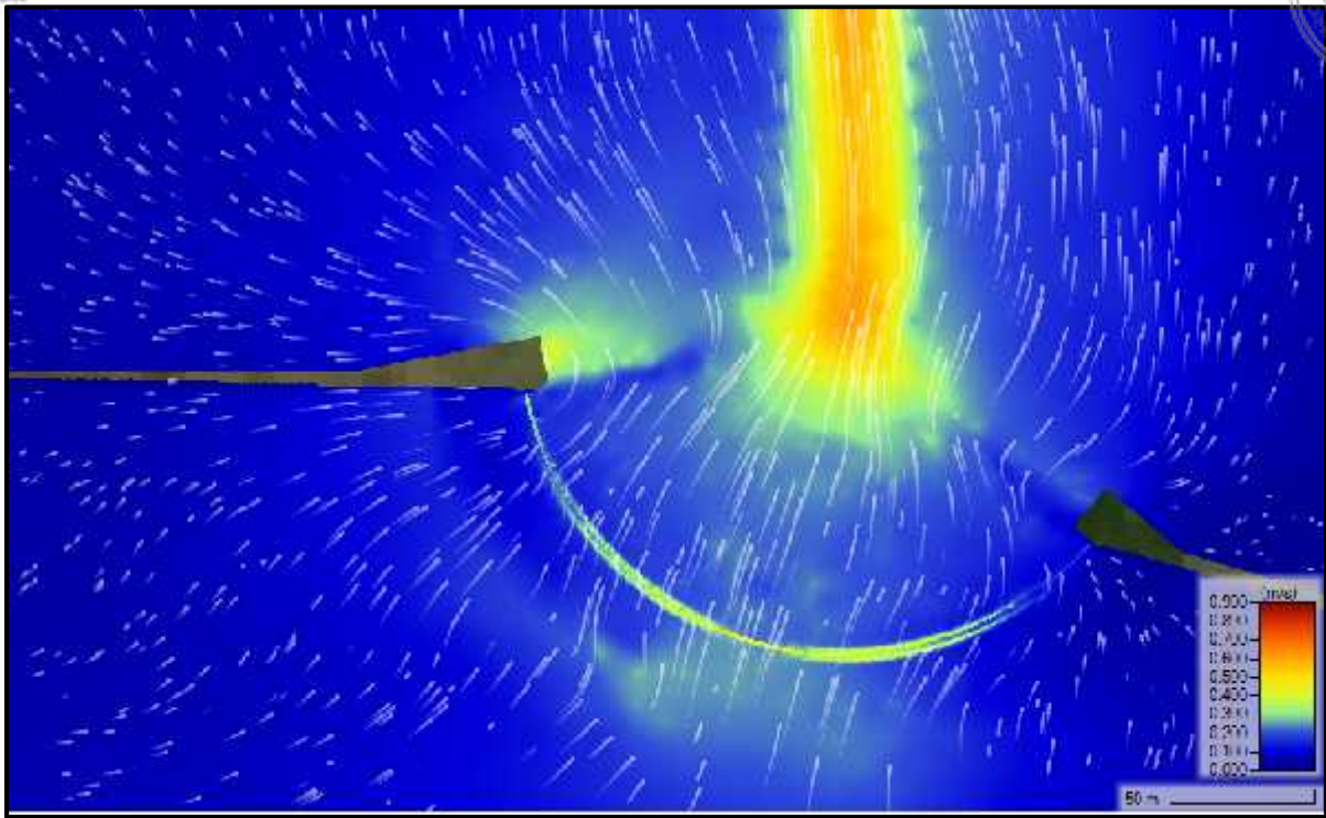
Imagen 24: Distribución del flujo previo desborde – Q no permanente
