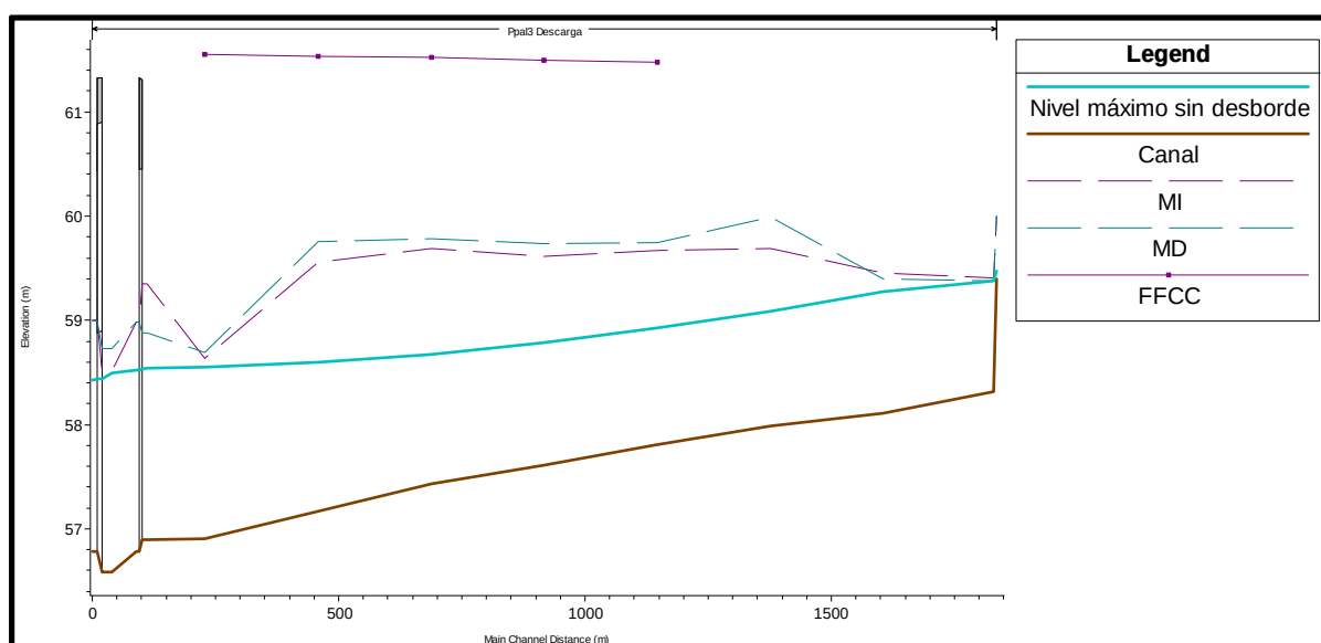
Imagen 27: Perfil Longitudinal con nivel máximo sin desborde
